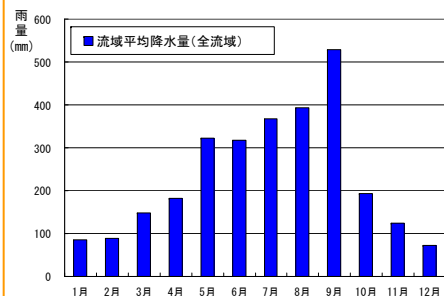
仁淀川の年平均降水量
