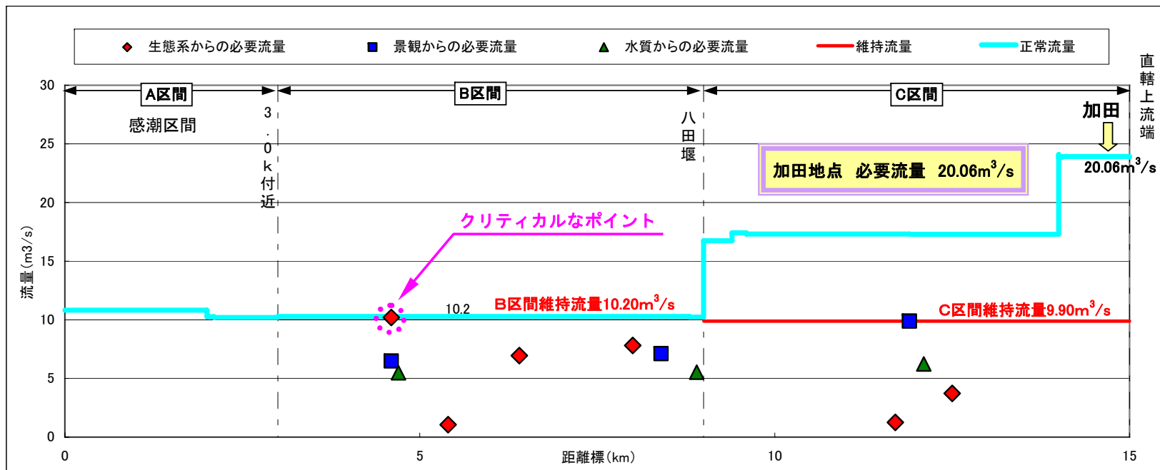
図 6-1 (2) 仁淀川水収支縦断図 非かんがい期 (3/1~3/31)
