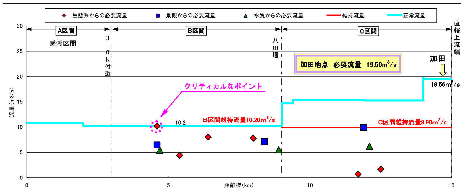
図 6-1 (1) 仁淀川水収支縦断図 非かんがい期 (1/1~2/28)
