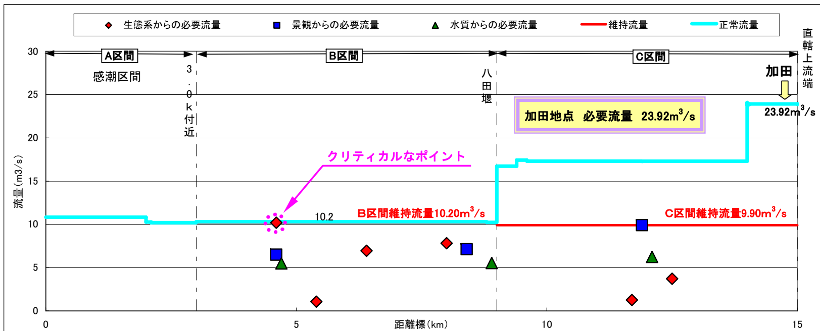
図 6-1 (4) 仁淀川水収支縦断図 かんがい期 (5/1~9/30)
