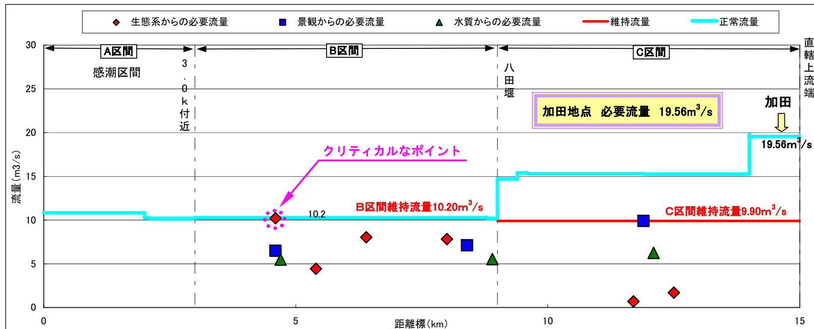
図 6-1 (6) 仁淀川水収支縦断図 非かんがい期 (11/1~12/31)
