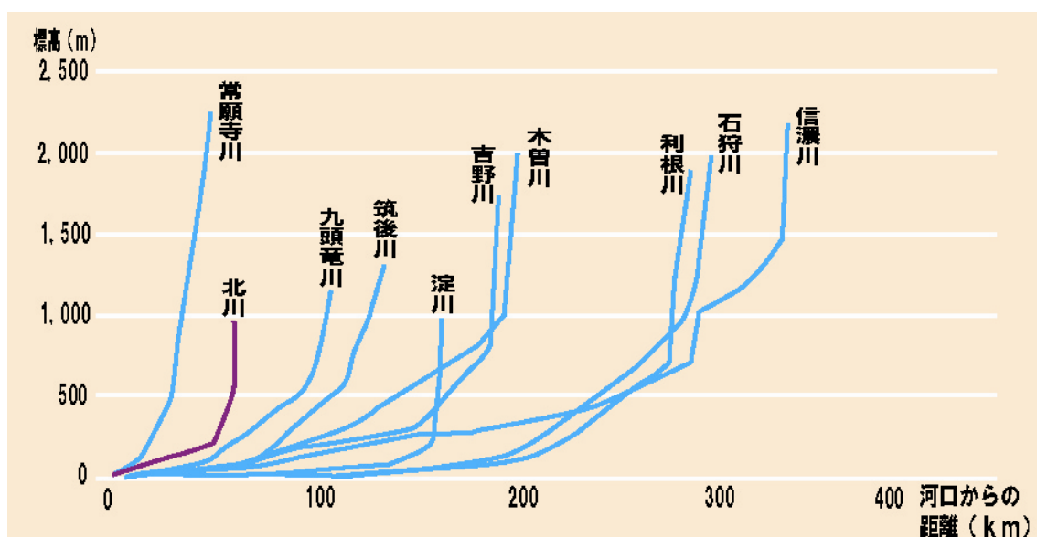
図 8-1 北川と主要河川の河床縦断模式図
