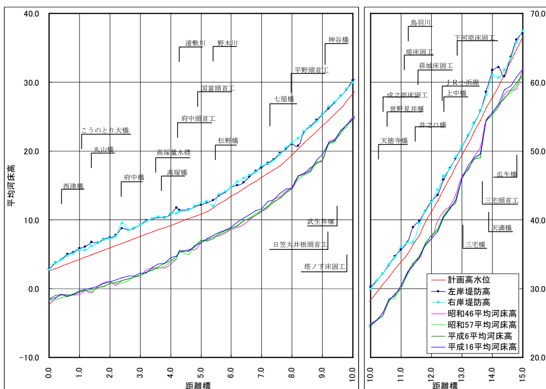
図 8-5 河床の経年変化縦断面図
