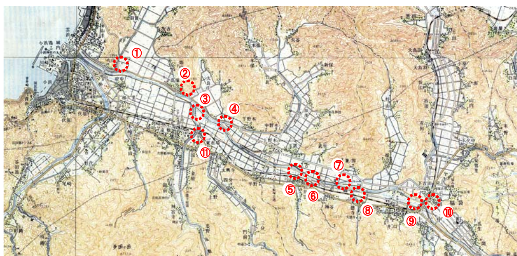
霞堤位置図
