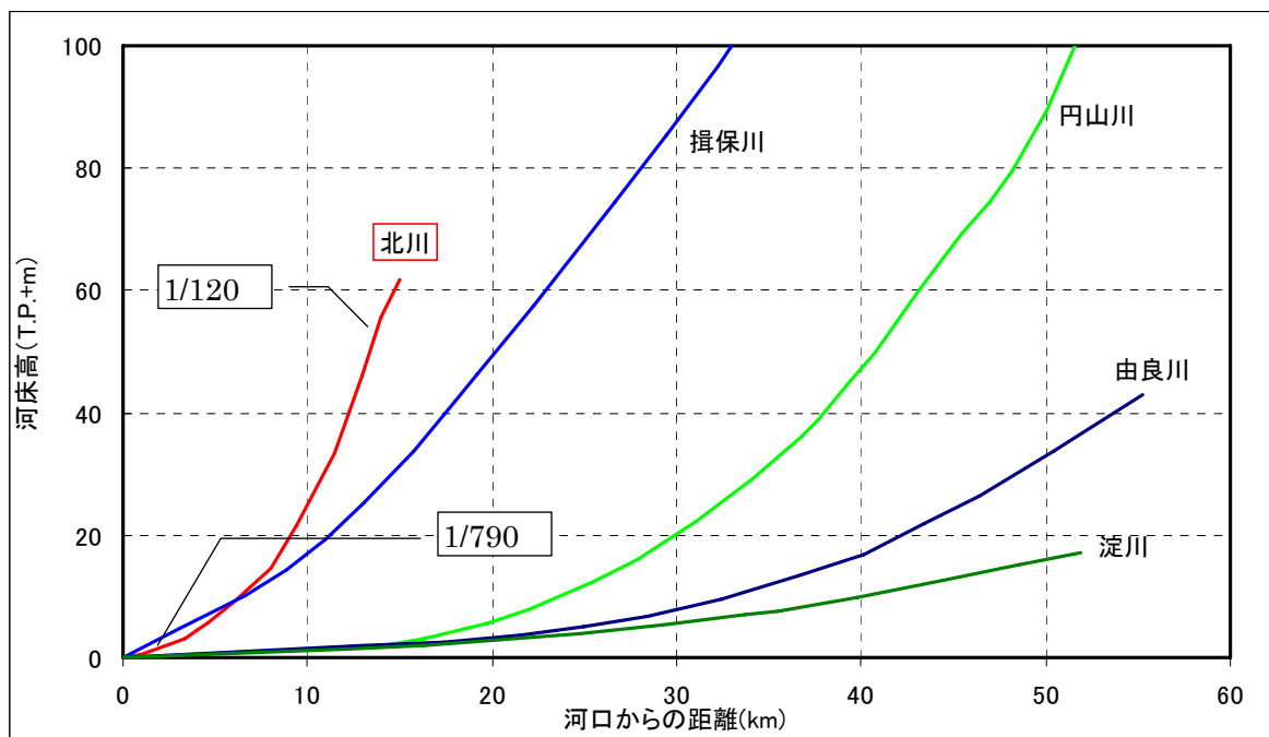
図 8-2 北川縦断図
