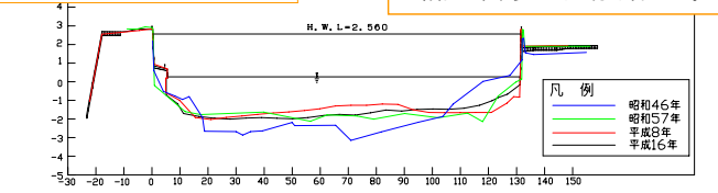
河口部経年変化横断面
