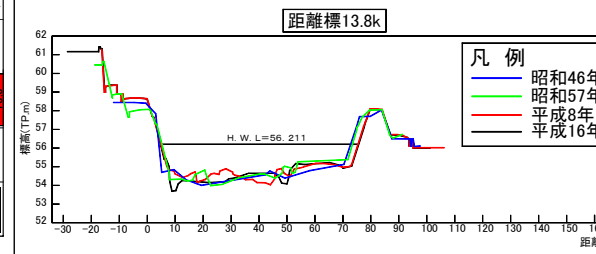
昭和46年度～平成16年度横断面比較図
