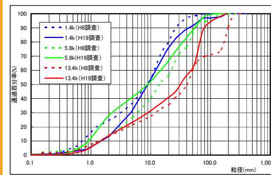
粒径加積曲線（H8, H19）
