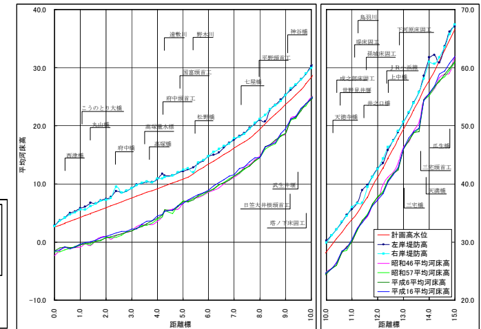
昭和46年度～平成16年度河床経年変化図
