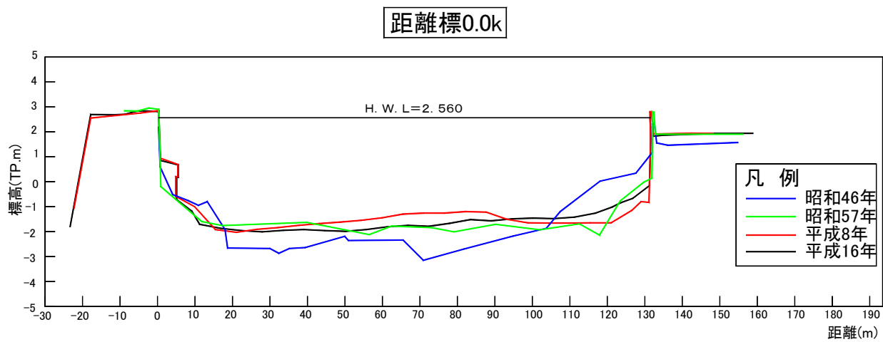
図3-2 北川河口部(0.0k)の横断図
