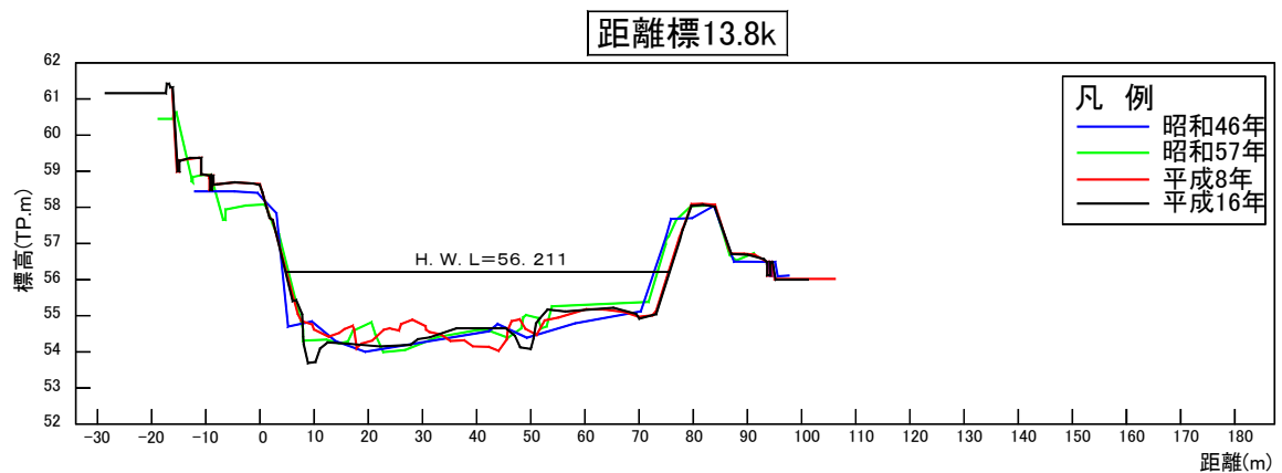
図2-4(2) 代表横断面図（北川13.8k）
