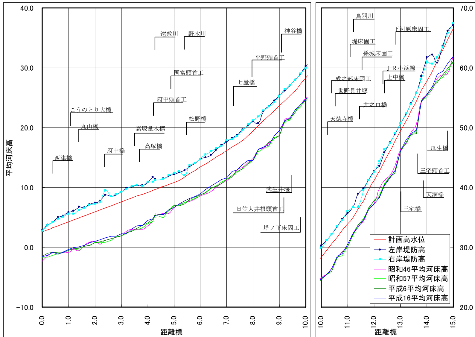
図2-2 北川平均河床高縦断図（昭和46年から平成16年）
