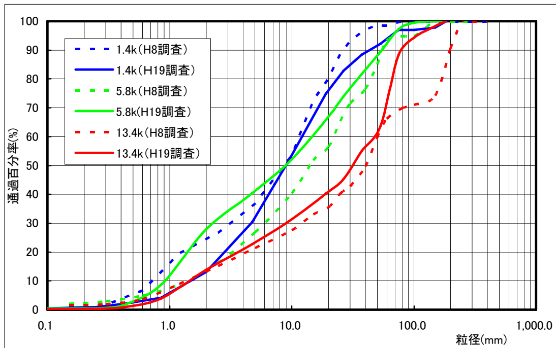
図2-3 北川河床材料変化図
