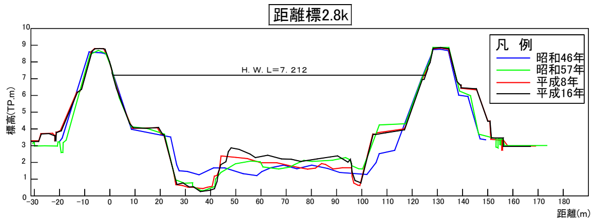
図2-4(1) 代表横断面図（北川2.8k）
