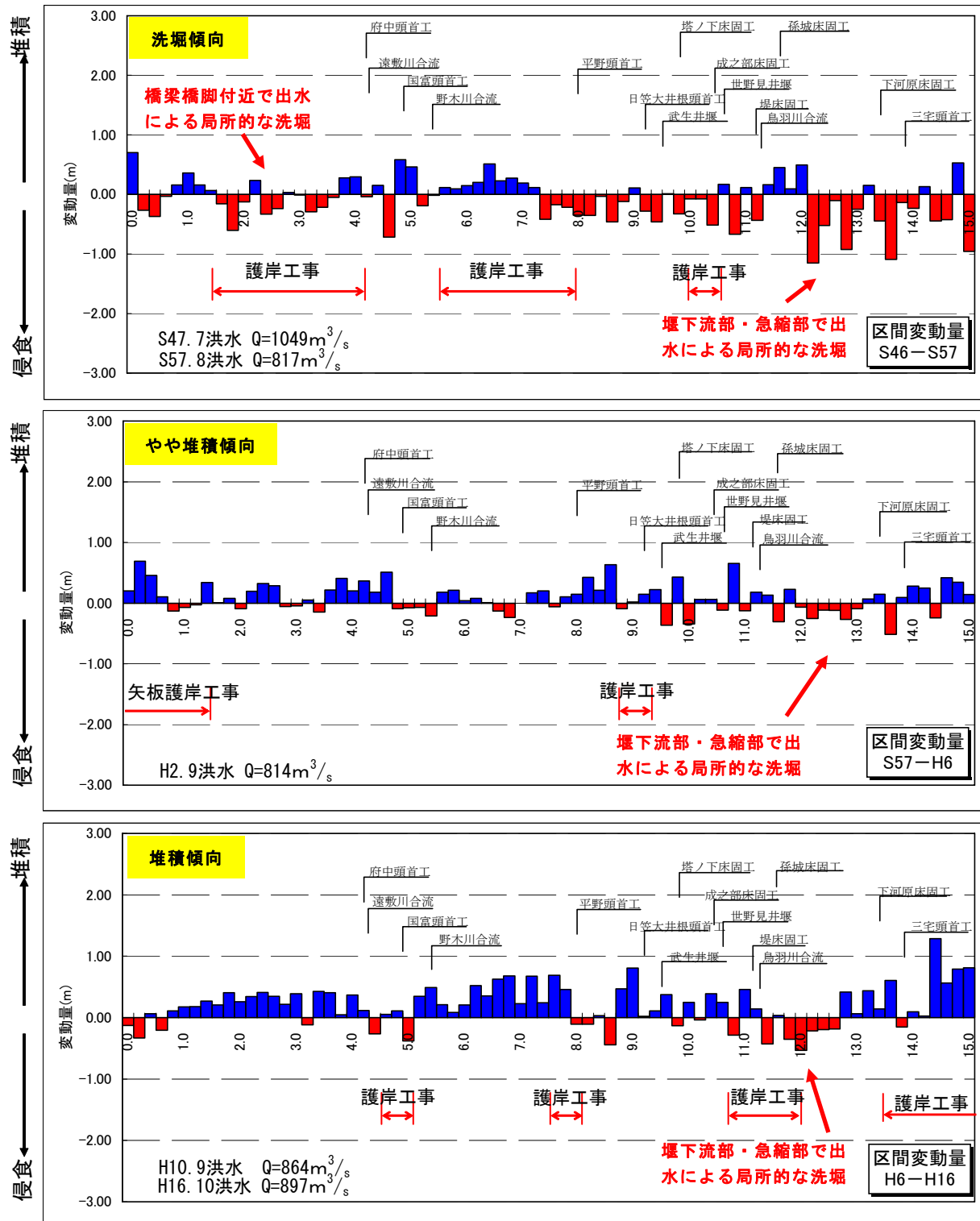
図2-1 北川平均河床高変化量の経年変化図（昭和46年～平成16年）
