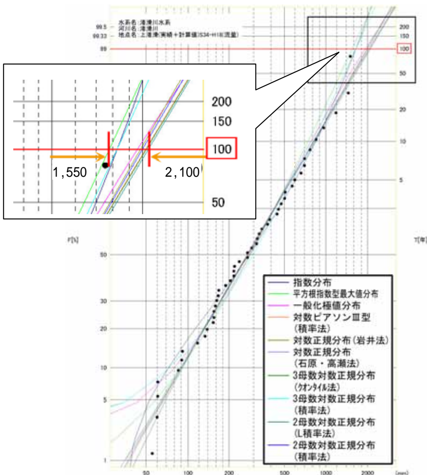
図 4-2 上渚滑地点流量確率図(S34 ~ H18:48 年間)
