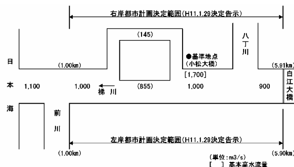
図 4-6 分水路計画流量配分図
