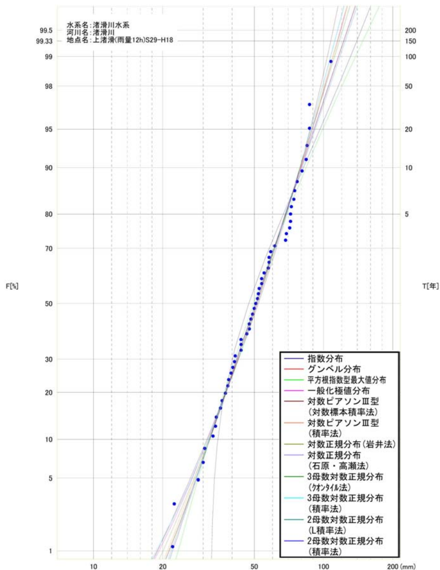
図 4-4 上渚滑地点における雨量確率評価(昭和 29 年～平成 18 年:53 カ年)
