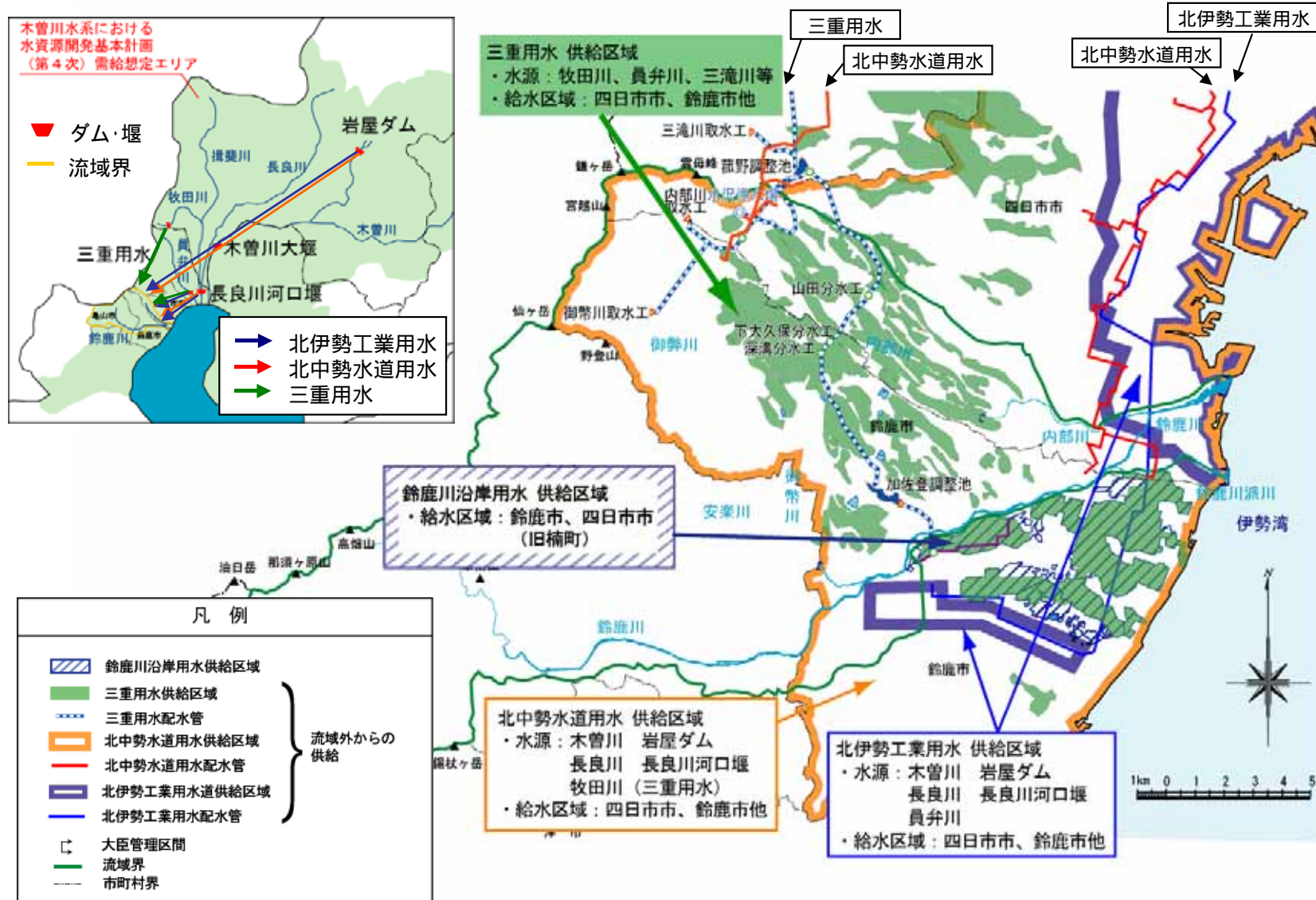
図 3-2 鈴鹿川流域の水資源供給区域
