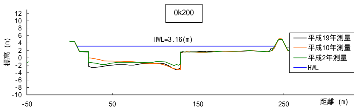
図 3-2 河口部 横断変遷図 (Ok200)
