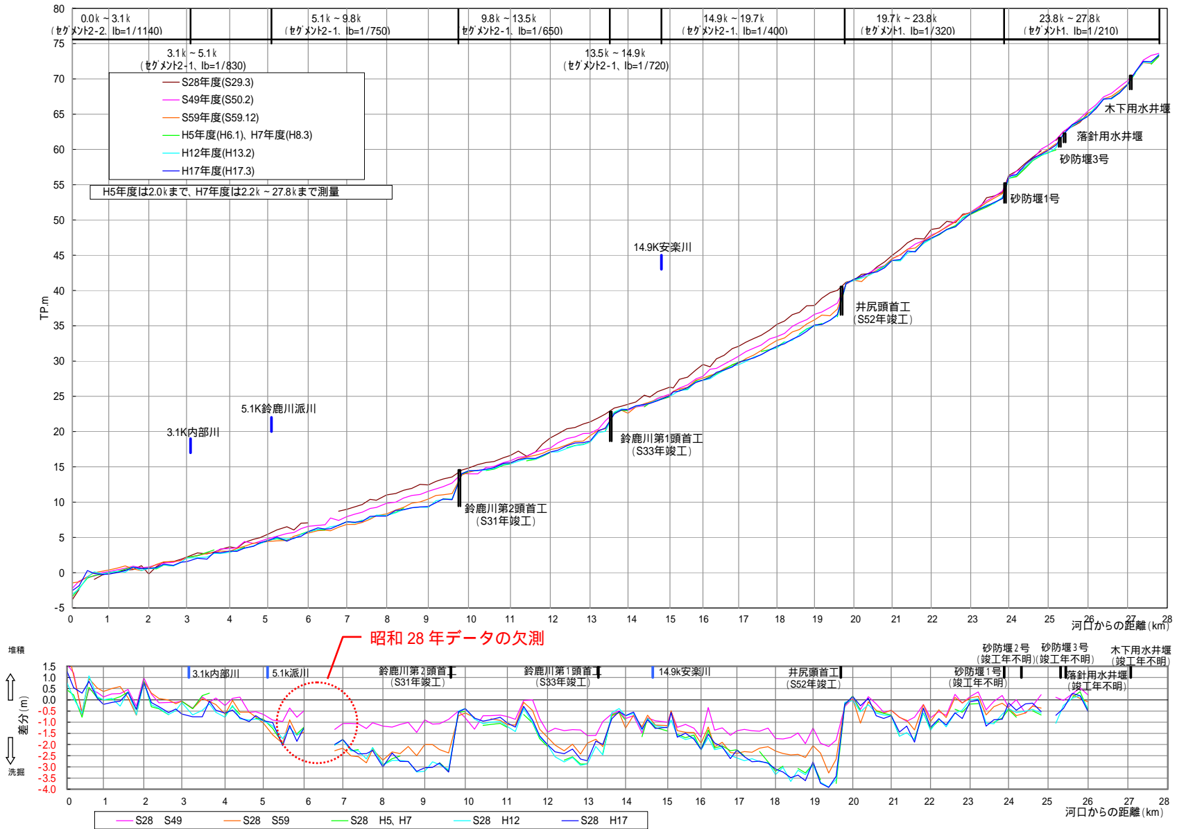
図 2-7 鈴鹿川低水路平均河床高縦断図
