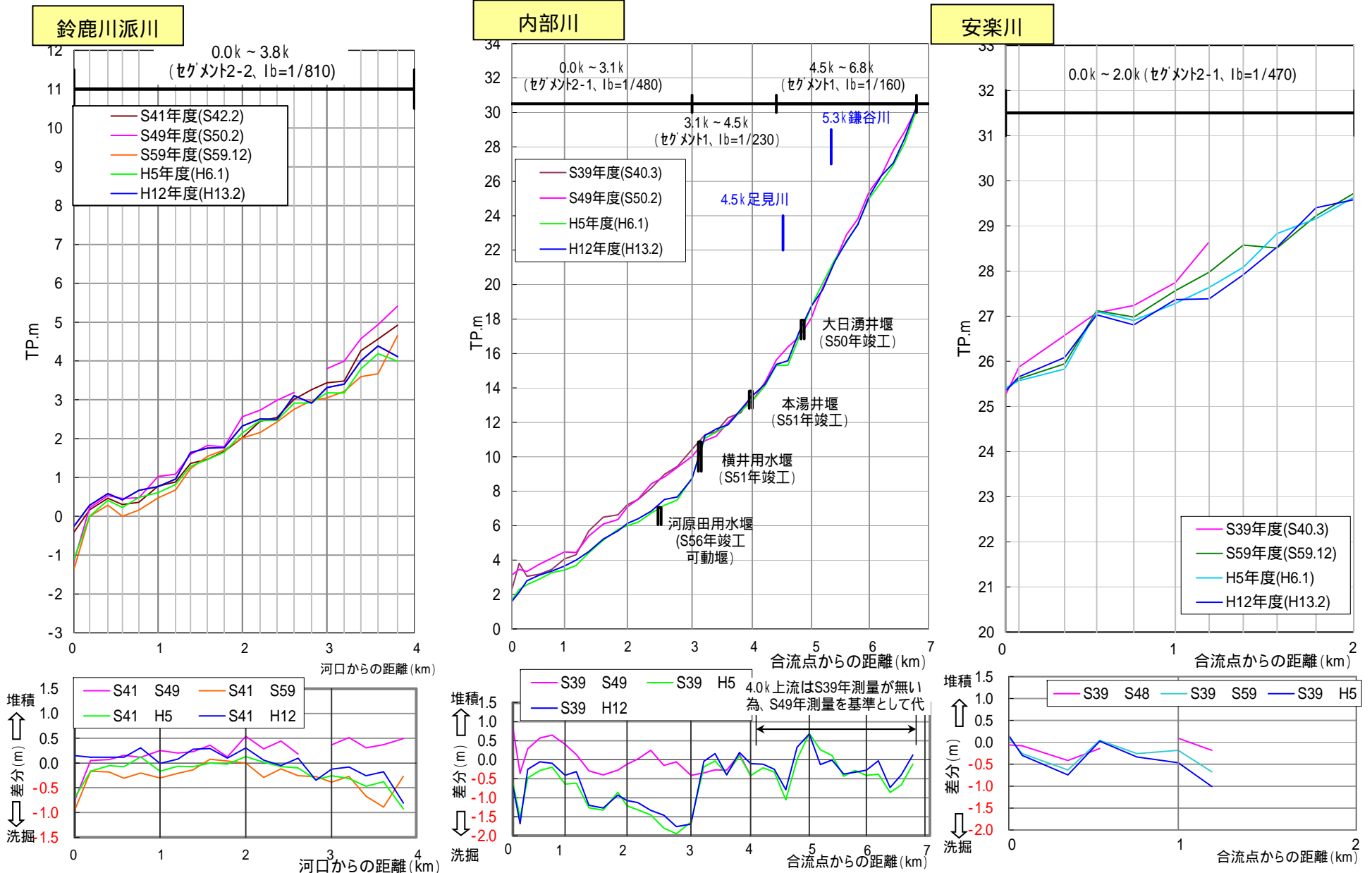
図 2-8 支派川平均河床高縦断面図
