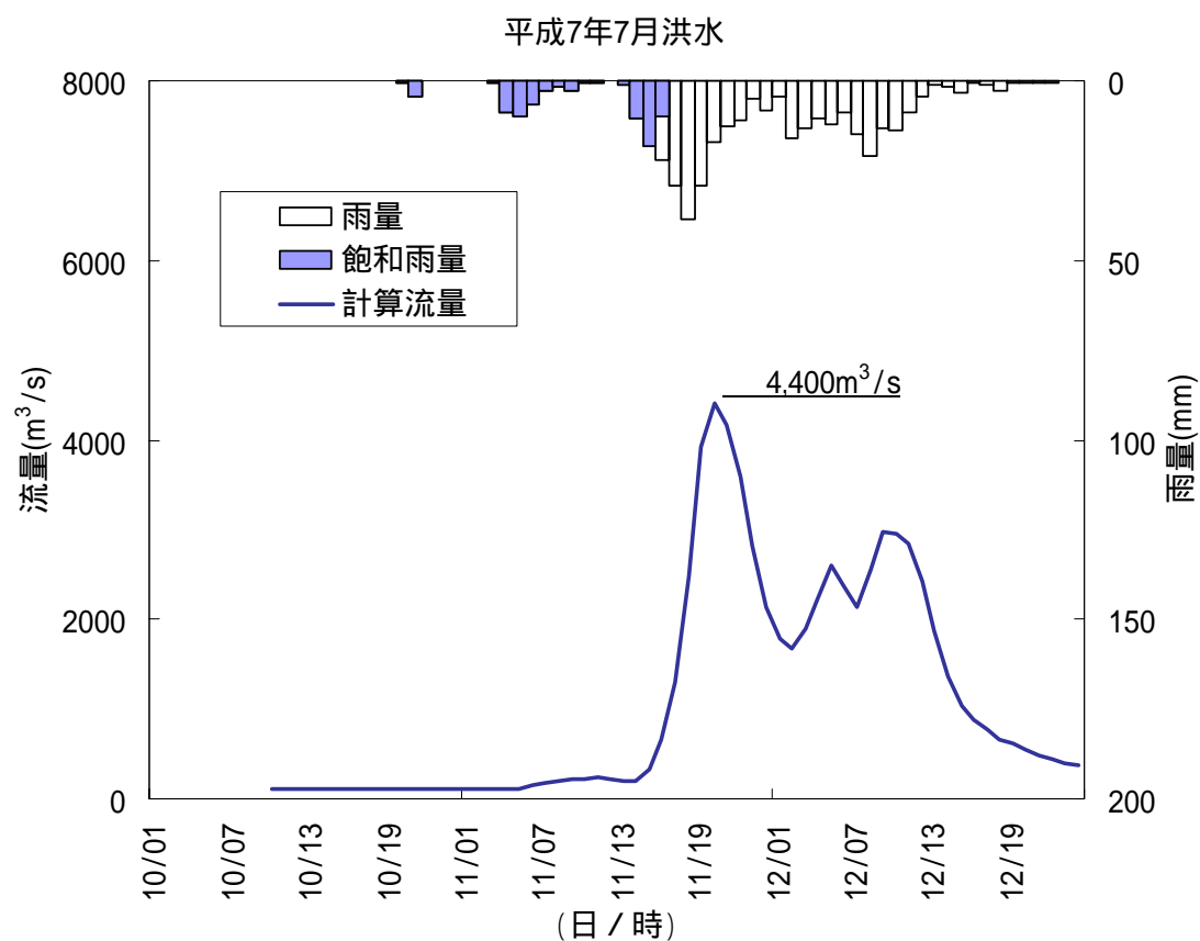
図4 - 9 山本地点における流出計算結果
