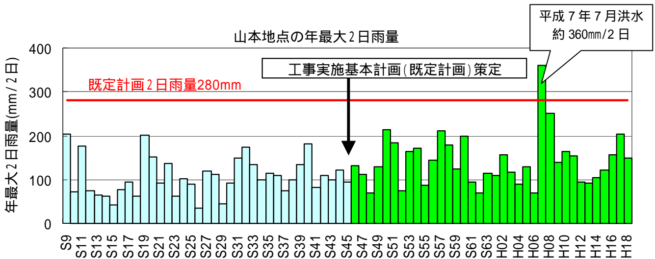
図4 - 2 年最大2日雨量 (山本地点上流域平均)
