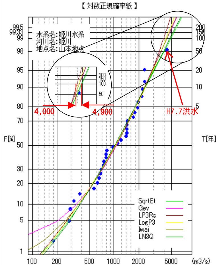
図4 - 10 基準地点山本における流量確率図（S34～H18, N=48ヶ年）
