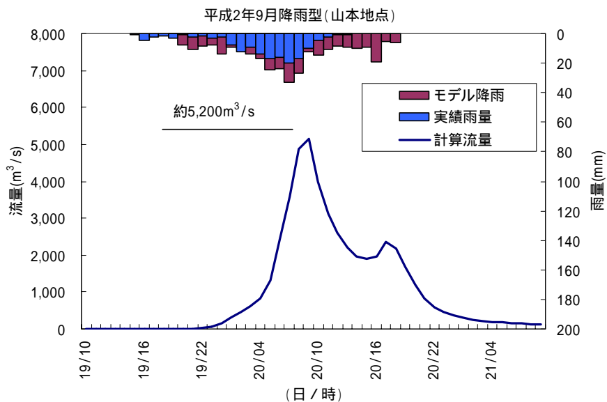
図4 - 7 1/100モデル降雨による検証ハイドログラフ(平成2年9月型洪水)
