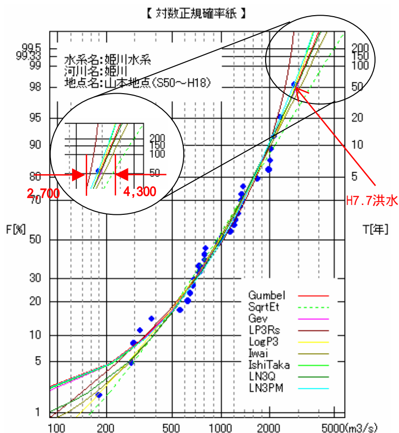
図4-3 基準地点山本における流量確率図（S34～H18, N=48ヶ年）
