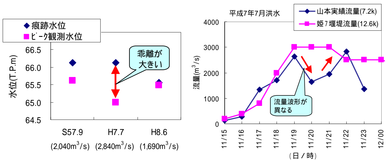
図4-8 痕跡水位および姫川第七堰堤の流況との比較
