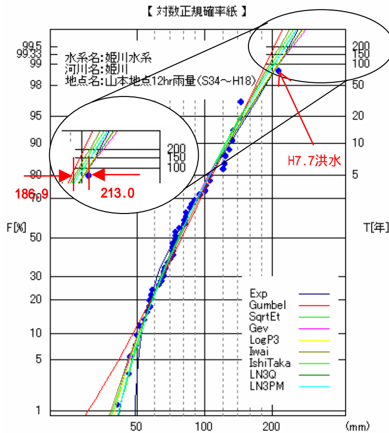
図 4 - 4 基準地点山本における雨量確率図 ( S34 ~ H18, N=48 ヶ年 )
