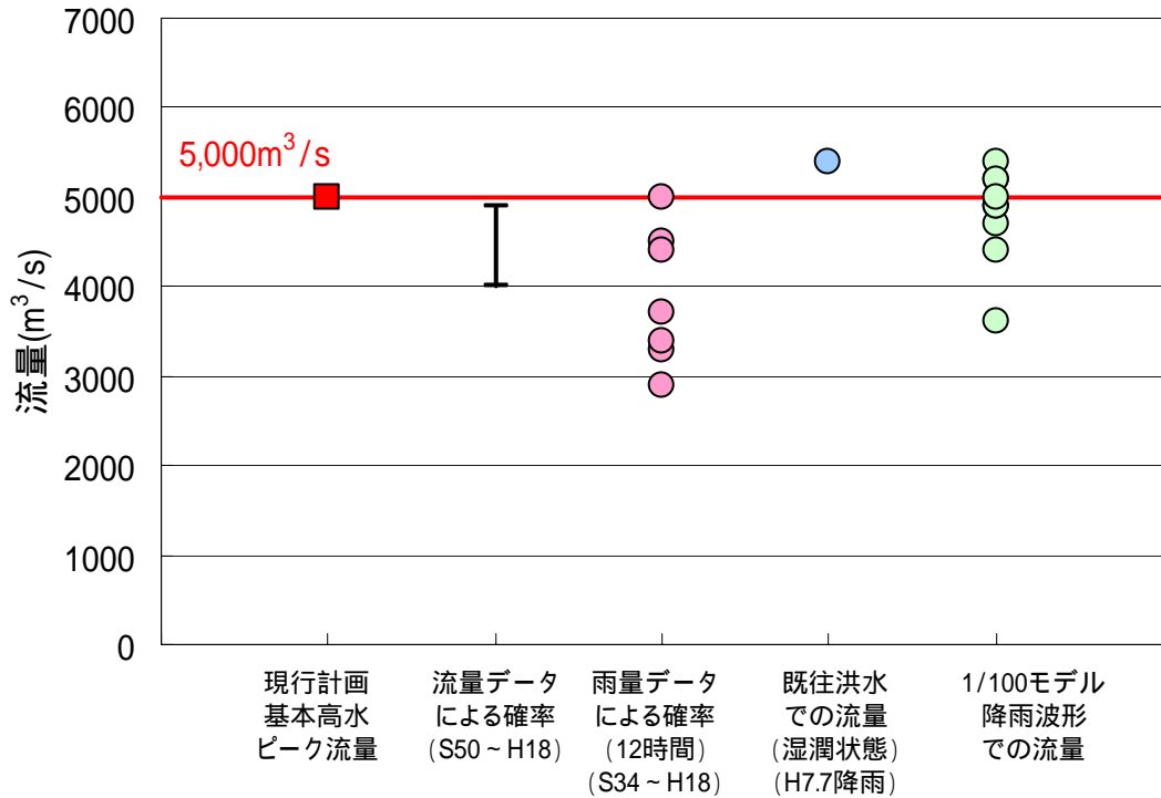
図4 - 1 1 各手法における基本高水のピーク流量算定結果
