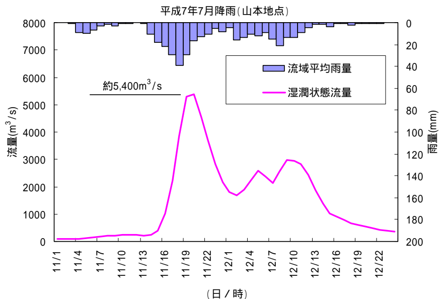
図4 - 6 湿潤状態での計算流量(平成7年7月型洪水)
