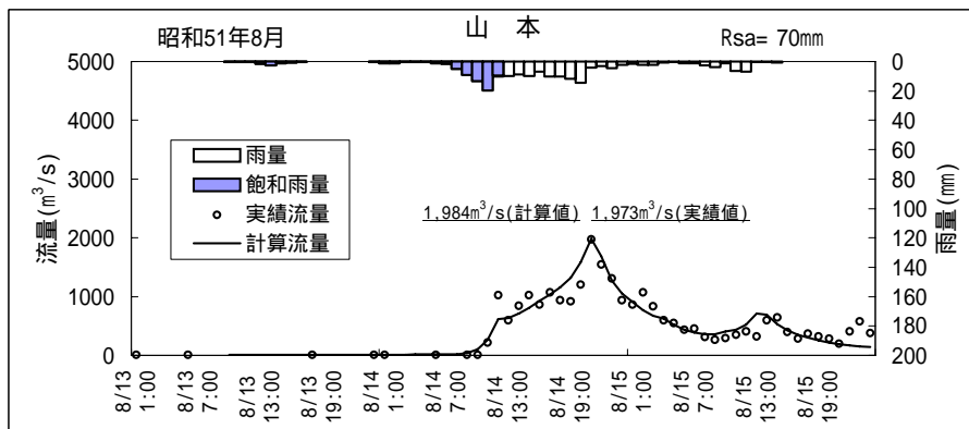
図 4 - 5 昭和 51 年 8 月洪水再現計算結果（山本地点）
