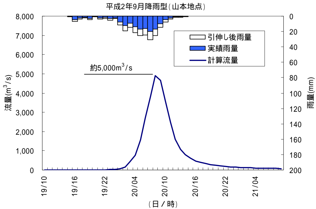
図4 - 1 2 基本高水のハイドログラフ (山本地点、平成2年9月型)
