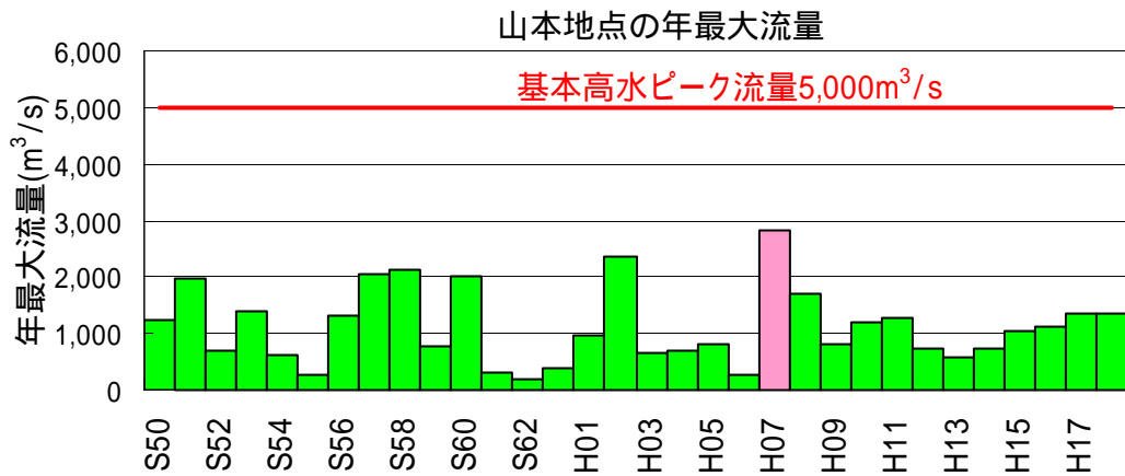
図4 - 1 年最大流量 (計算流量：山本地点)
