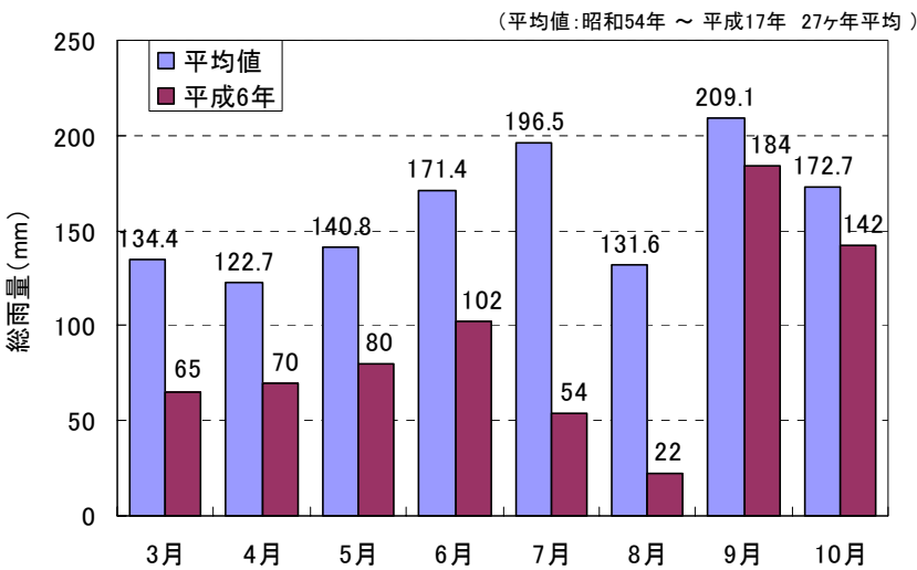
図 5-6 小松雨量観測所における平成6年(1994年)と27ヶ年平均の月別総雨量の比較
