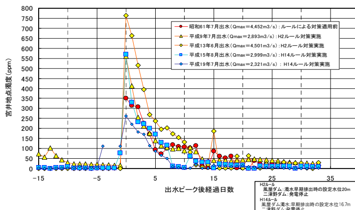
図 7-2 宮井地点における出水後の濁度時系列
