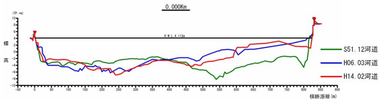
図 5-2 熊野川河口部（0.0k）の横断面図
