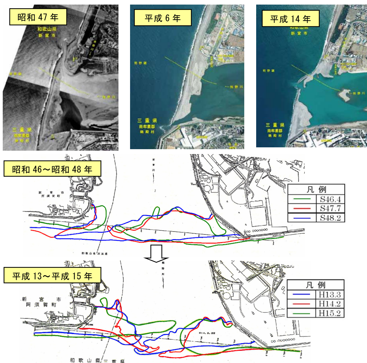
図 5-1 熊野川河口部経年変化
