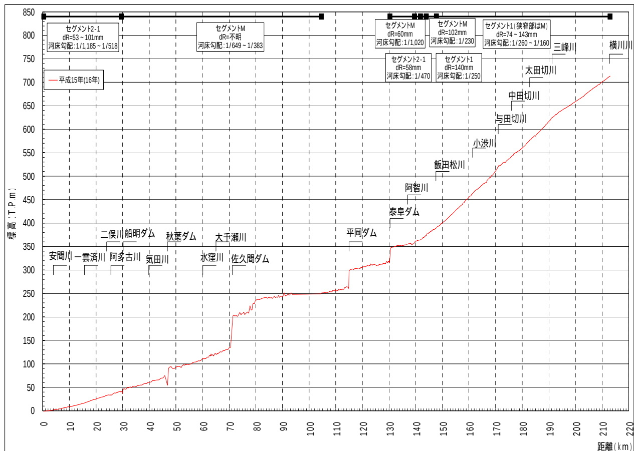
図 8 - 1 天竜川の河床勾配
