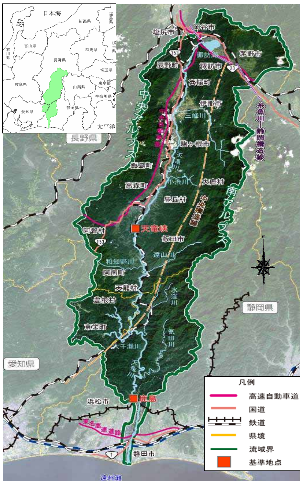
図 1-1 流域図
