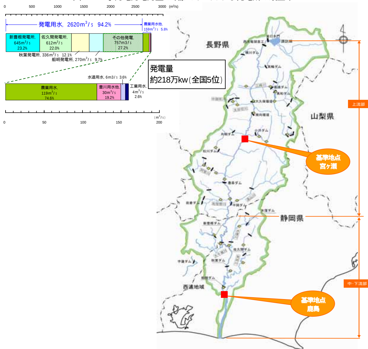
図 5.3 ダム位置図
