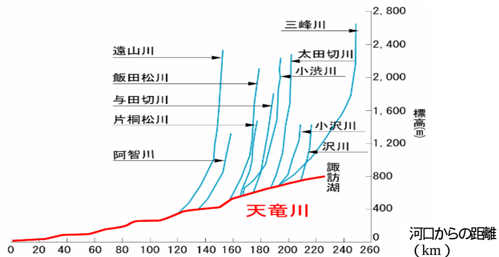
図 1 - 4 河床勾配図
