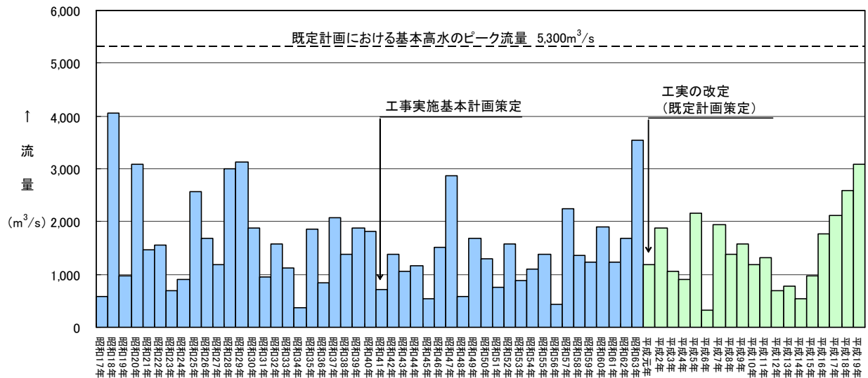
図 4-1 年最大流量(基準地点城南)
