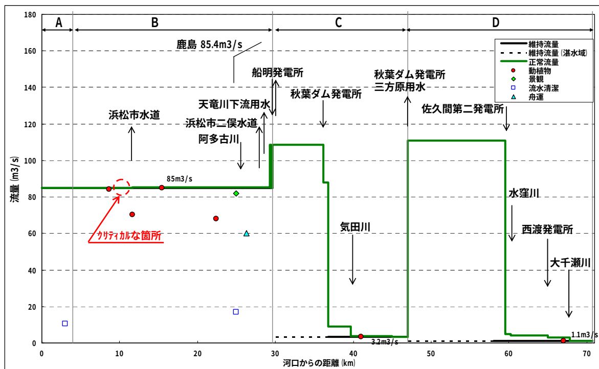
図 6-8 天竜川正常流量縦断図 (中・下流) (4/5)
