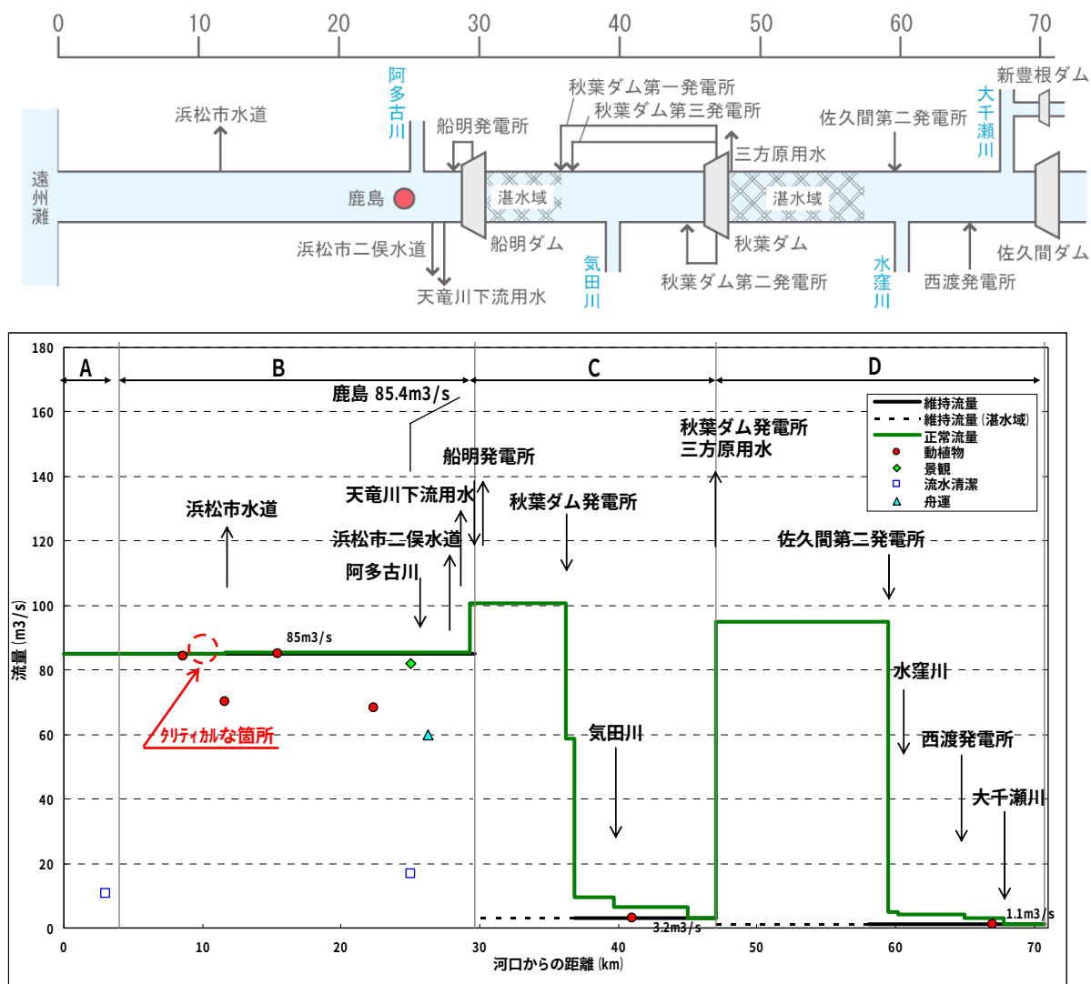
図 6-9 天竜川正常流量縦断図 (中・下流) (5/5)
