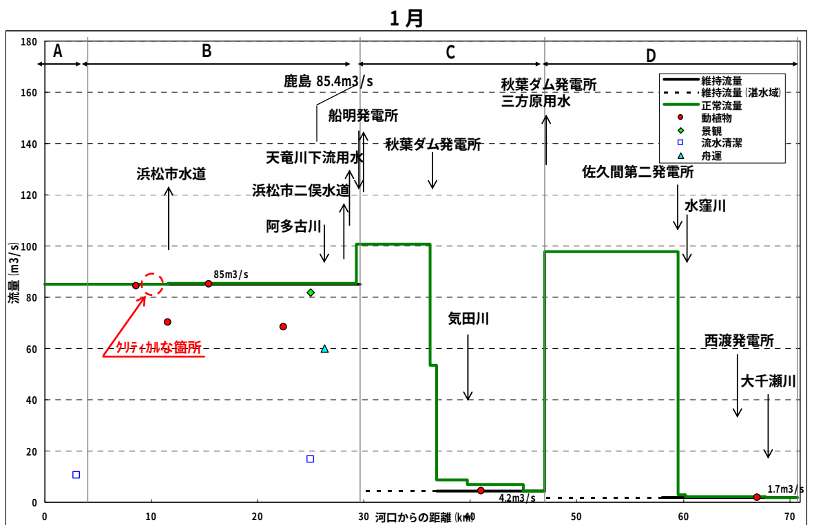
2~3月 * B区間における動植物からの維持流量は既定計画等に基づく検証値 図 6-5 天竜川正常流量縦断面図 (中・下流) (1/5)
