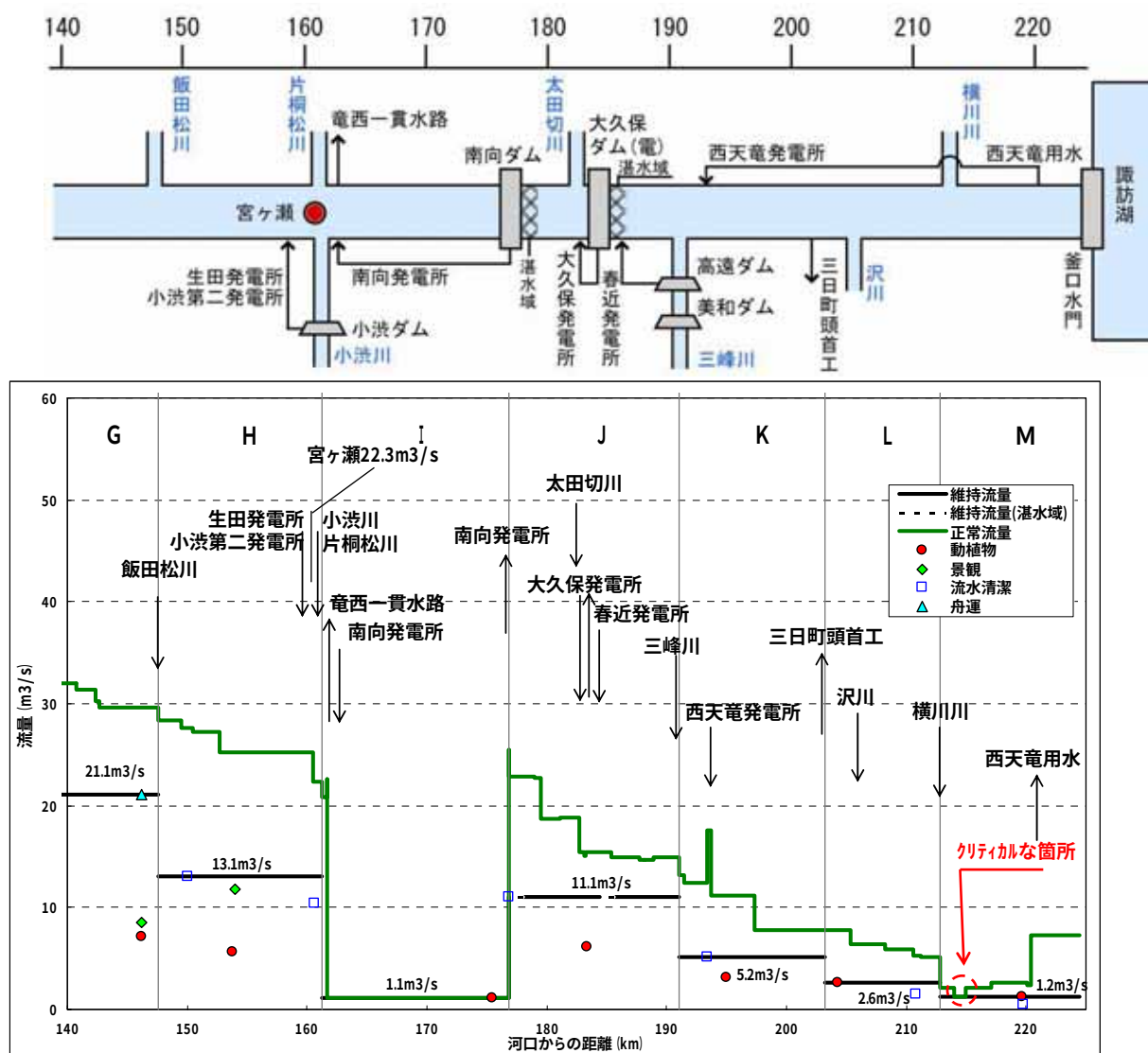
図 6-4 天竜川正常流量縦断図(上流) (4/4)
