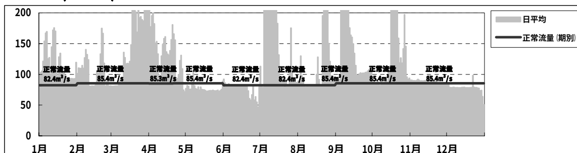
図 6-13 日平均流量図(鹿島地点:平成13年~平成17年)
