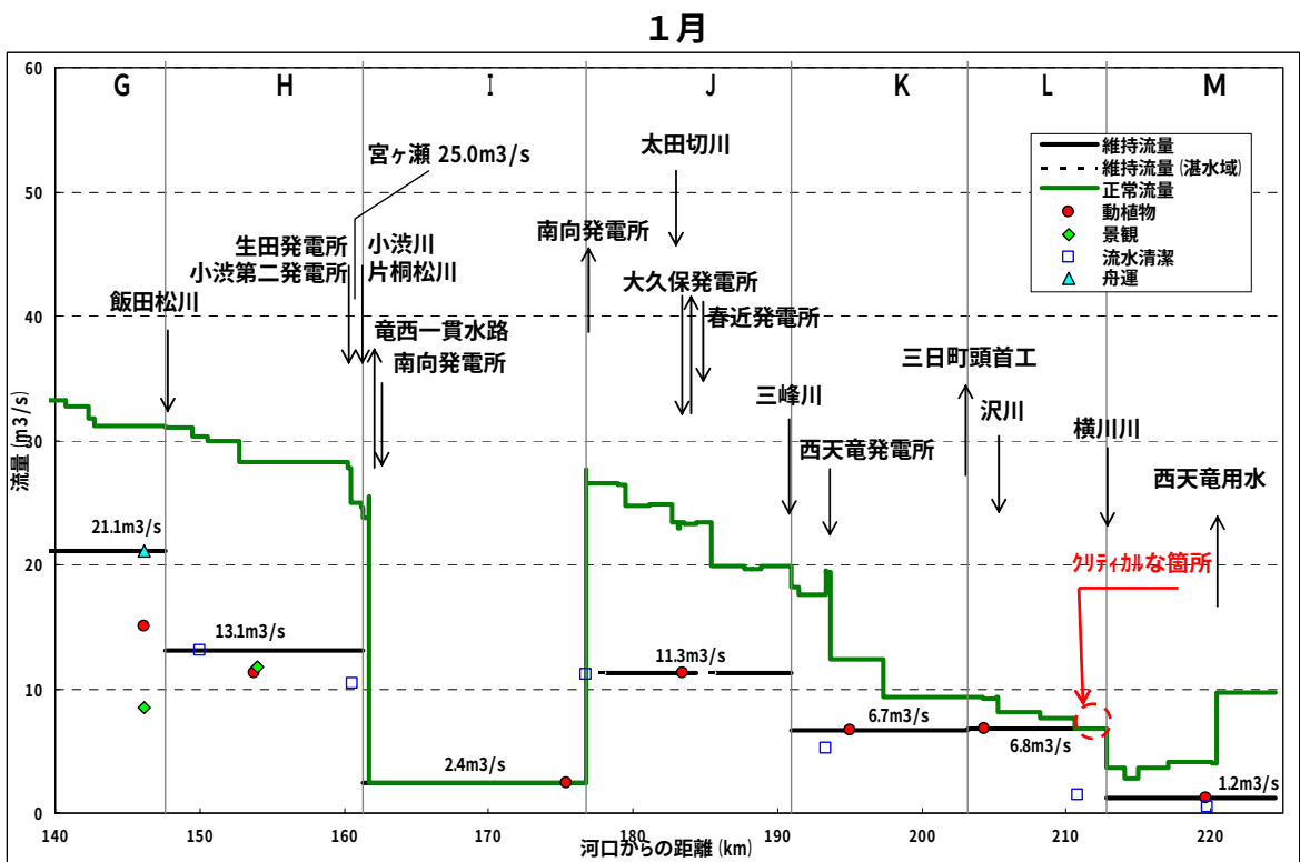
図 6-1 天竜川正常流量縦断面図 (上流) (1/4)
