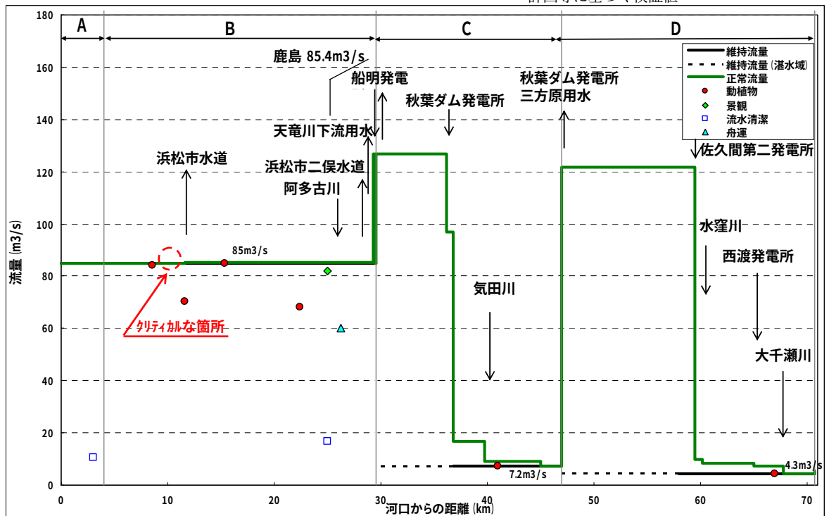
図 6-6 天竜川正常流量縦断図 (中・下流) (2/5)
