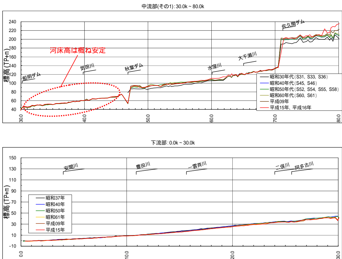
図 3-6 : 天竜川平均河床高縦断面図(佐久間ダム下流河道)
