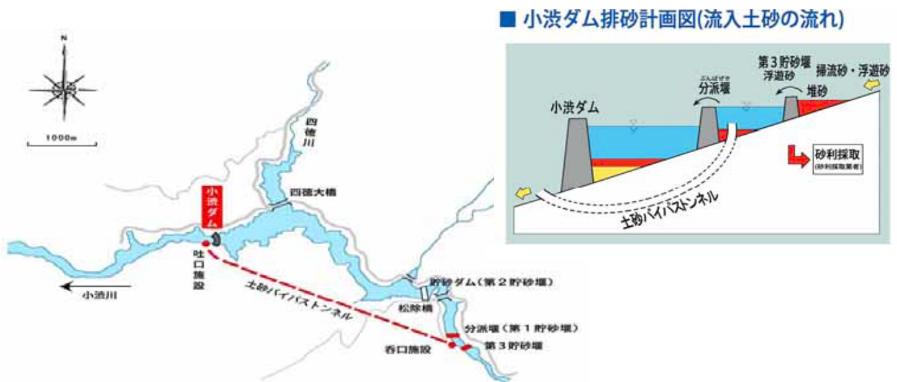
図 4-21：小渋ダム洪水バイパストンネルイメージ図
