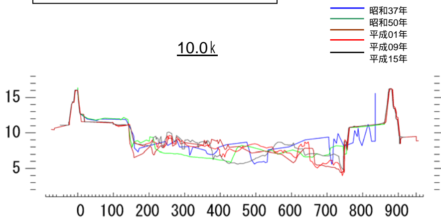
図 4-11：河床形態の変化（澁筋固定箇所と動的平衡箇所）
