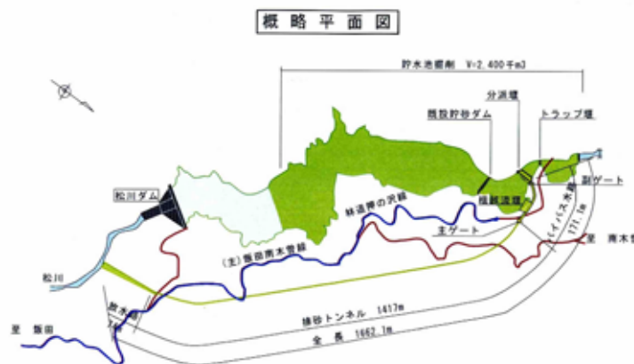
4-22：松川ダム洪水バイパスの概要
