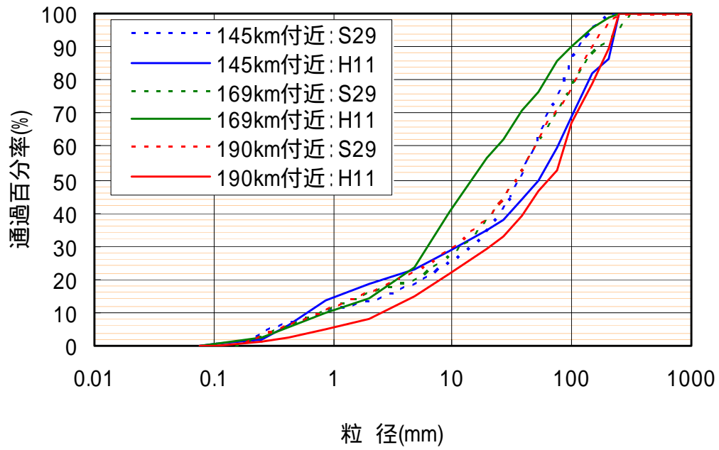
図 4-4 : 上流部の粒度分布
