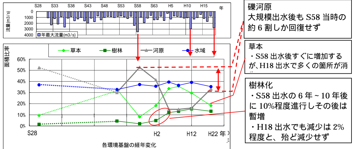
図 4-5 : 河原及び樹林の割合経年変化(139.6 k ~ 191.2 k)
