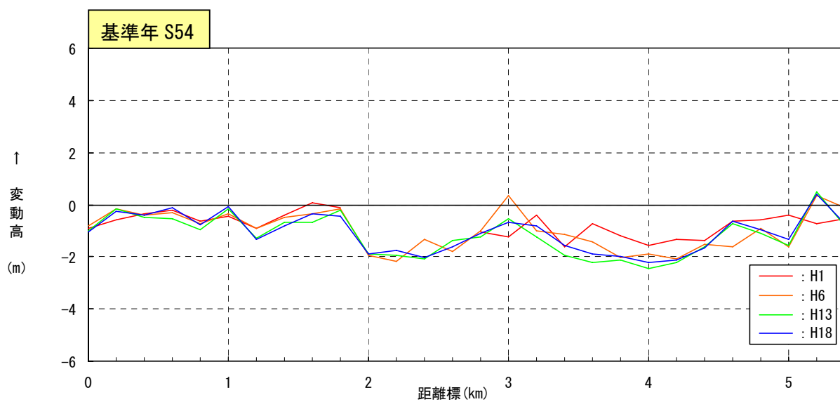
図 2-3 (1) 浜戸川低水路平均河床高縦断面図
