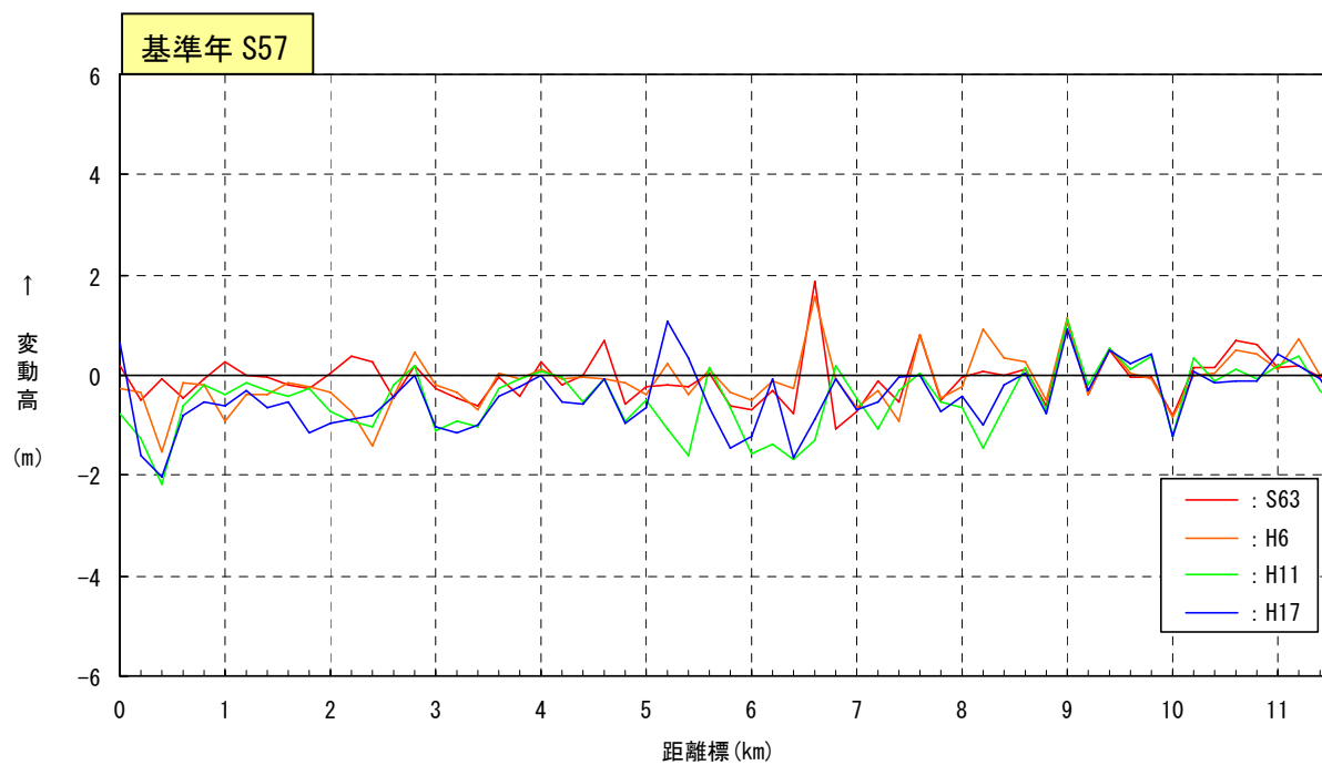
図 2-4 (1) 加勢川低水路平均河床高縦断面図
