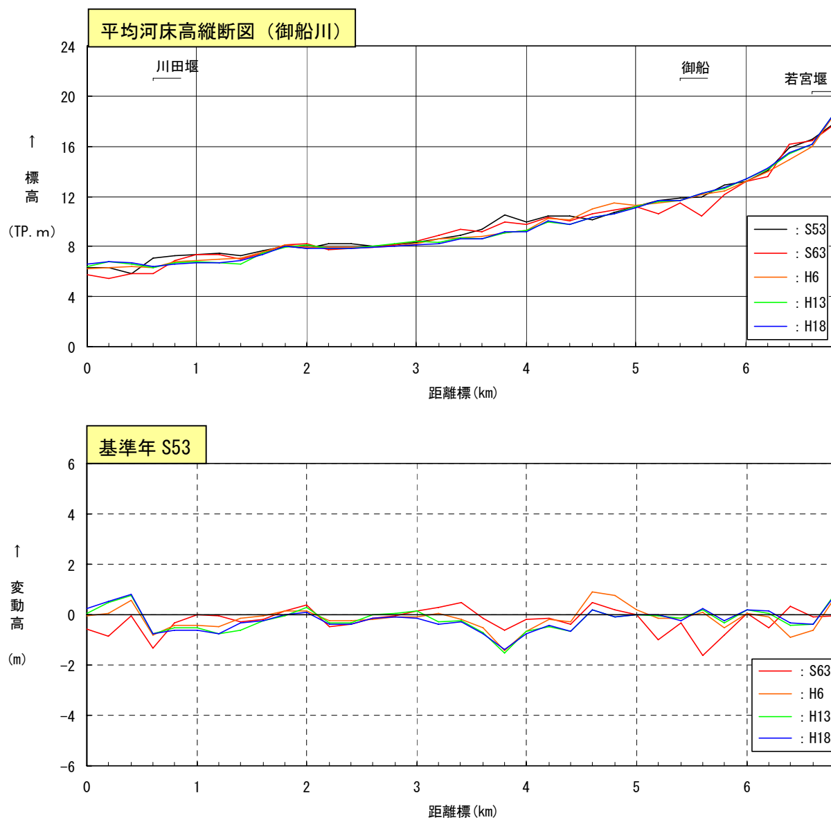
図 2-5 (1) 御船川低水路平均河床高縦断図
