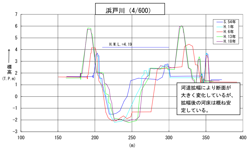
図 2-7 (2) 代表断面における横断形状の経年変化
