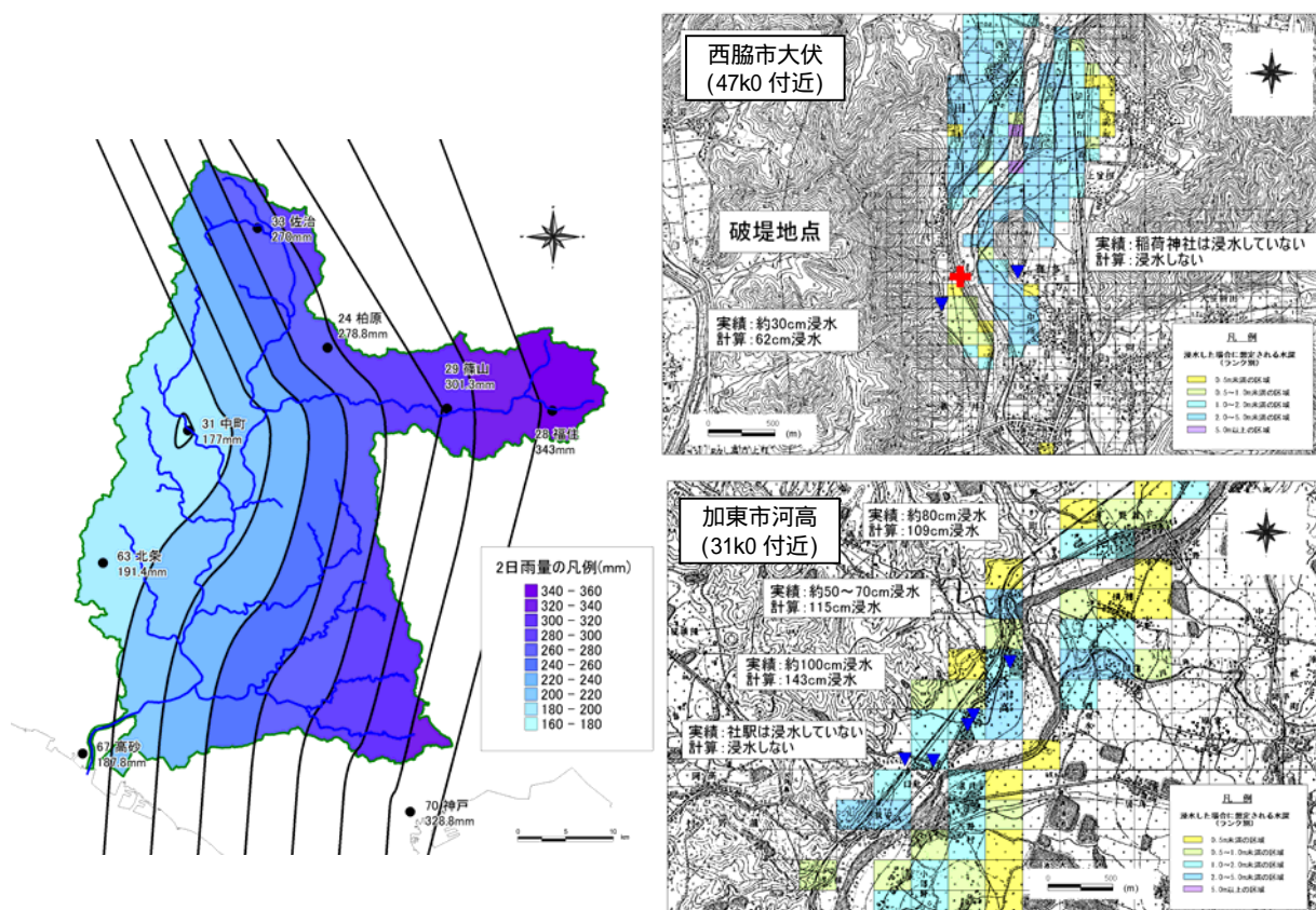
昭和 20 年 10 月洪水 等雨量線図および浸水範囲図
