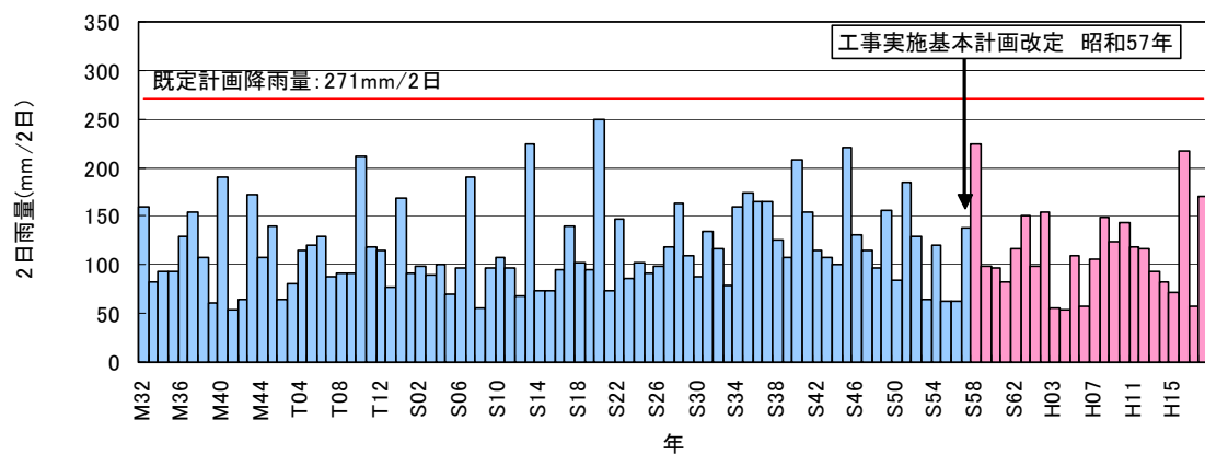
図 4-5 国包地点上流年最大 2 日雨量
