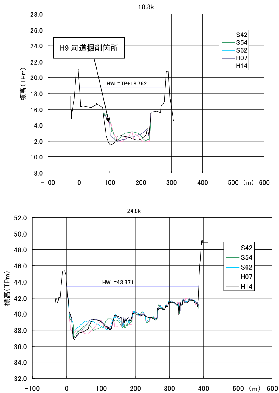
図 8-5 (2) 河道形状の変動特性
