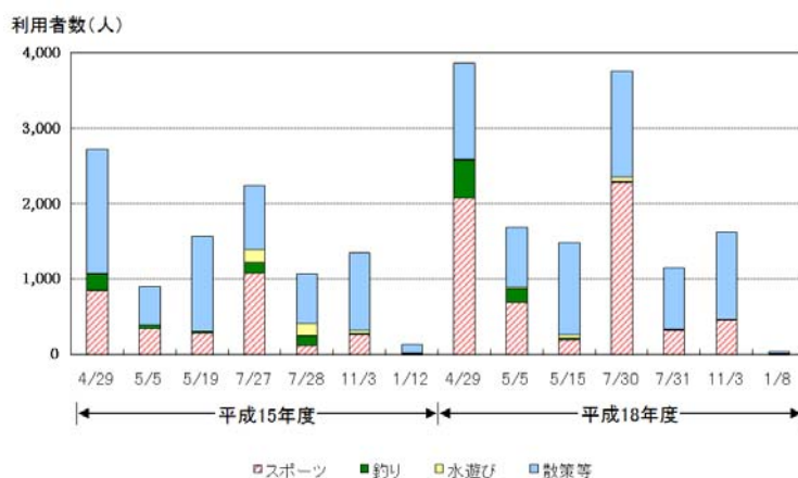
図 7-1 河川利用目的の傾向
