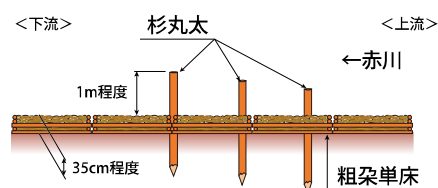
水制工の構造図
