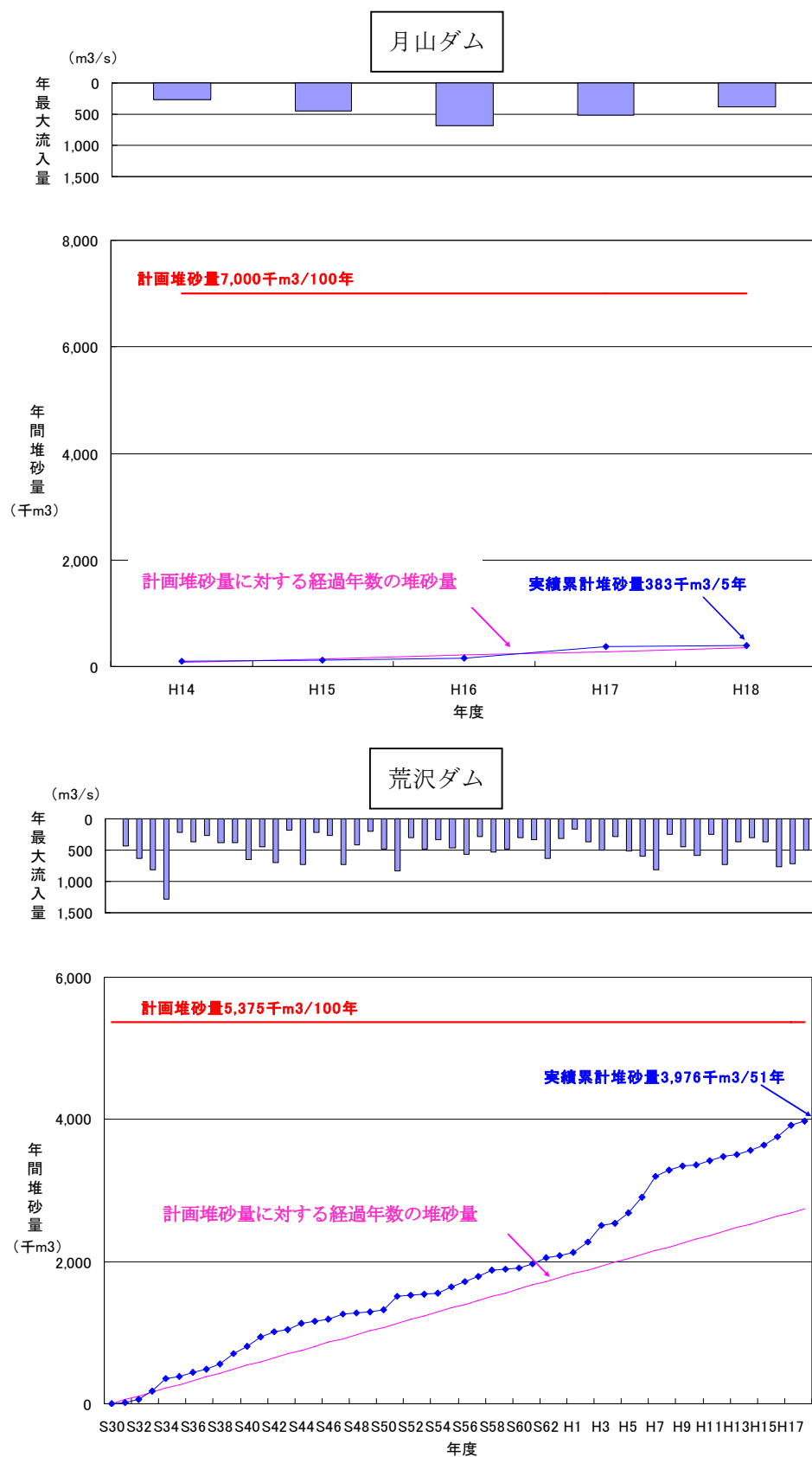
図 8-4 ダムの堆砂状況
