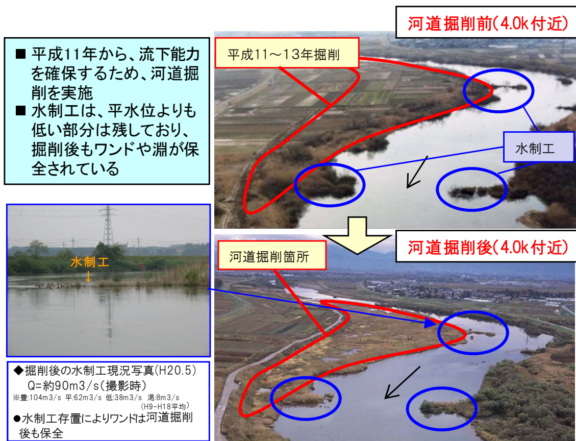
河道掘削の水制工の状況（実施済み）
