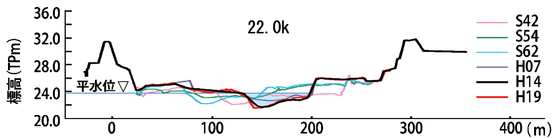
図 2-6 河道形状の変動特性
