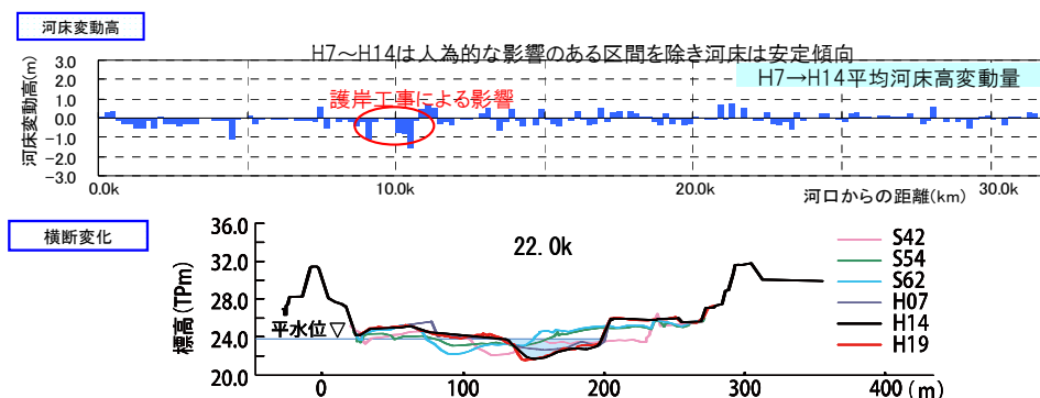
図 6-1 河床変動高 (H7-H14) 及び横断形年変化
