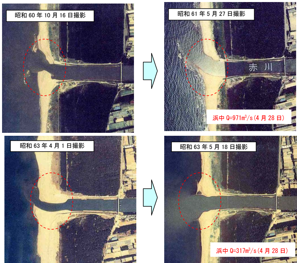
図 4-1 (2) 赤川河口の空中写真 (融雪後の河口状況)
