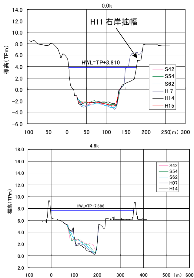
図 2-5 河道形状の変動特性
