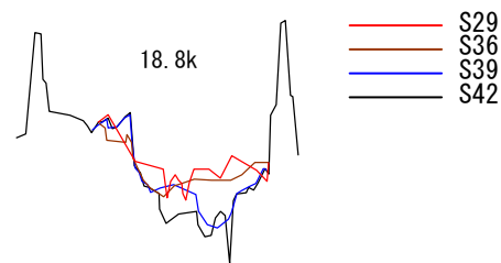
図 2-4 砂利採取の盛んな昭和 30 年代の横断変化
