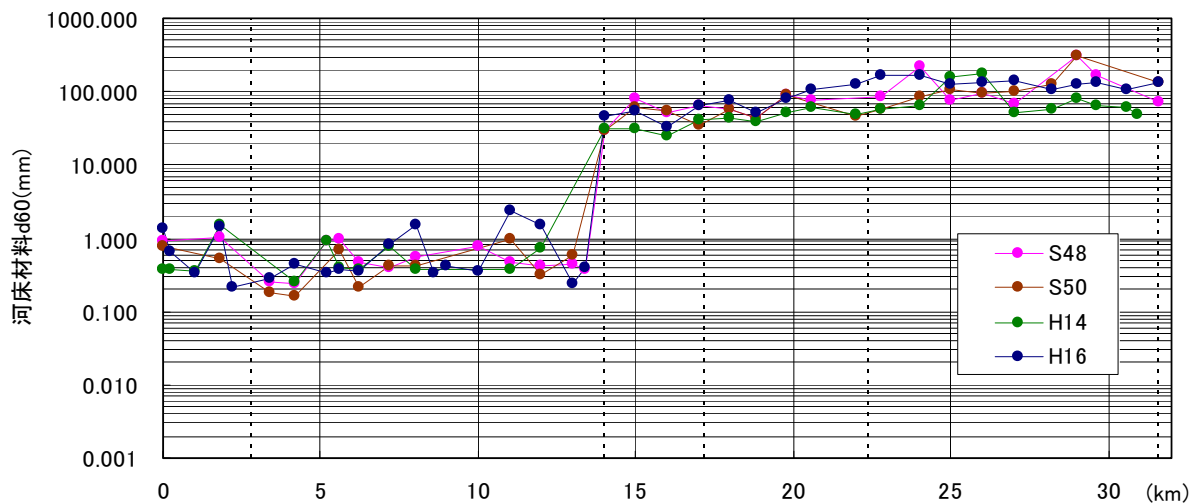
図 2-9 代表粒径の縦断分布の経年変化 (S48~H16)
