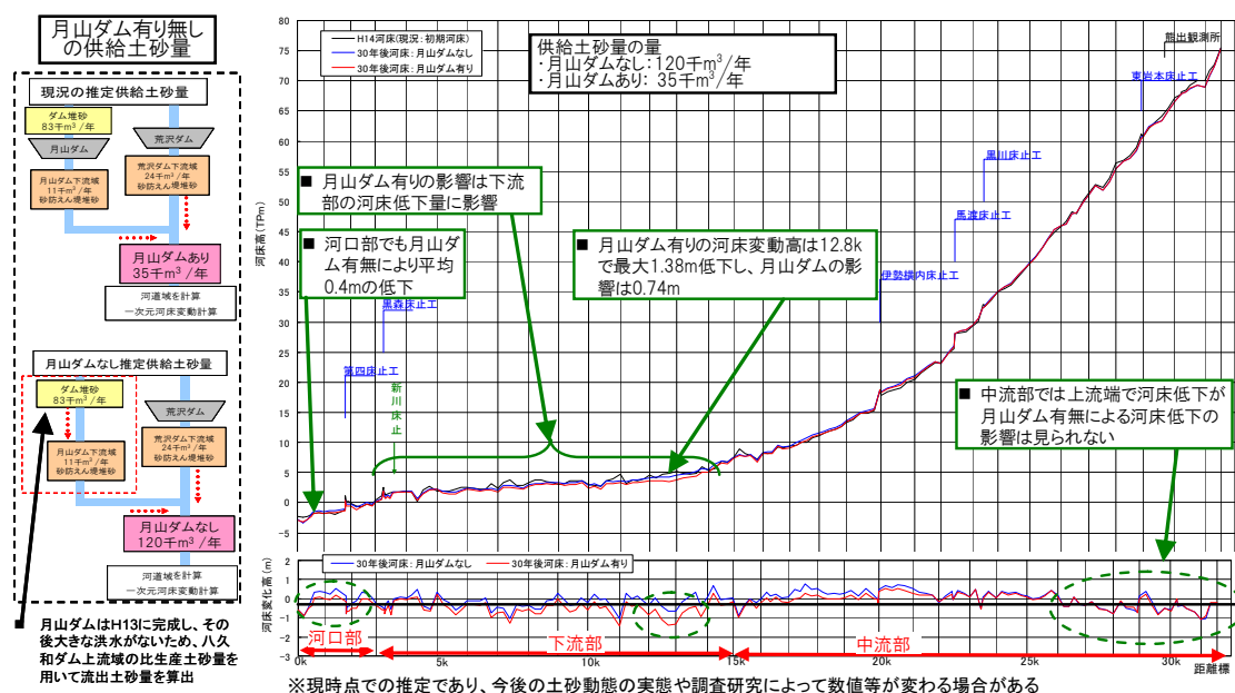
図 6-2 河床変動計算結果 (月山ダム有・無)
