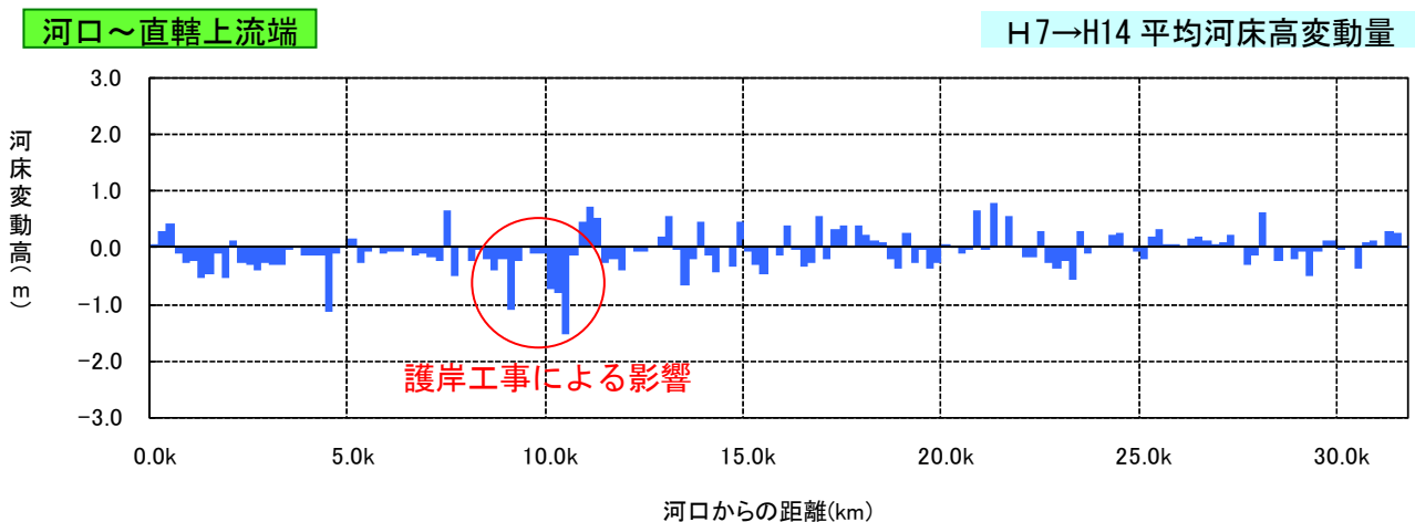
図 2-3 河床変動量の経年変化（赤川）
