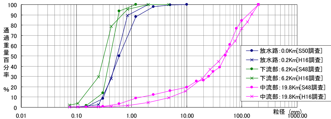
図 2-8 河床材料の経年変化 (S48~H16)
