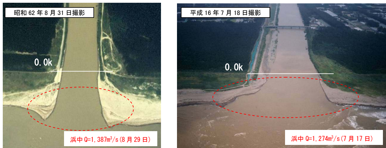
図 4-1 (1) 赤川河口の空中写真 (中小洪水直後の河口状況)
