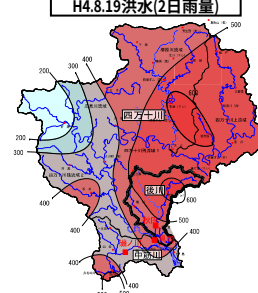
後川 戦後最大洪水 H4.8.19洪水(2日雨量)
