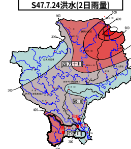
中筋川 戦後最大洪水 S47.7.24洪水(2日雨量)
