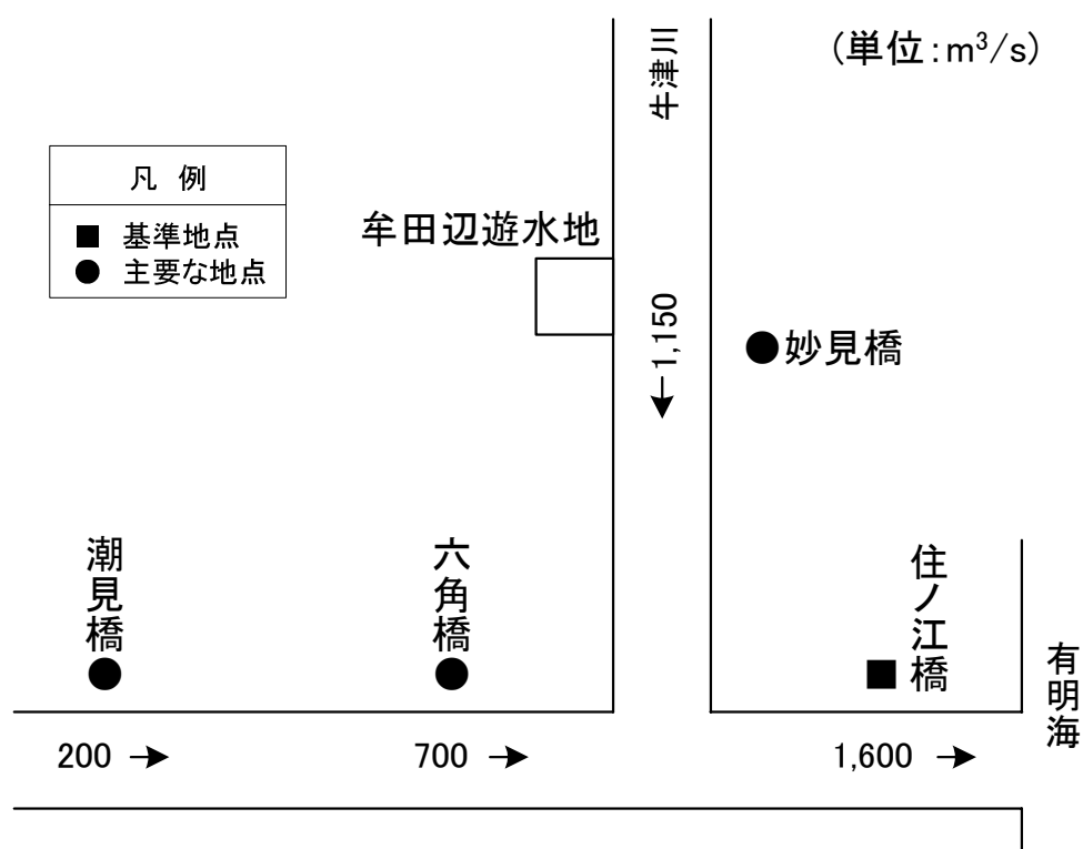
図 6-1 六角川計画高水流量図
