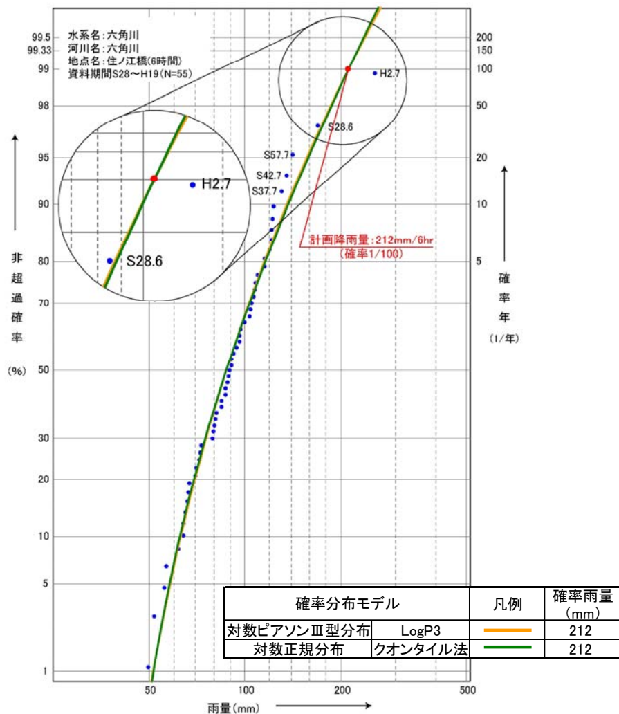
図 4-4 住ノ江橋地点における雨量確率評価（昭和 28 年～平成 19 年：55 カ年）
