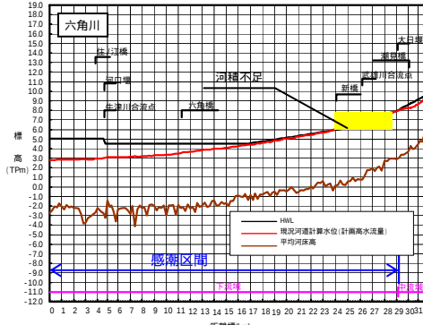
六角川現況流下能力(水位縦断面図)
