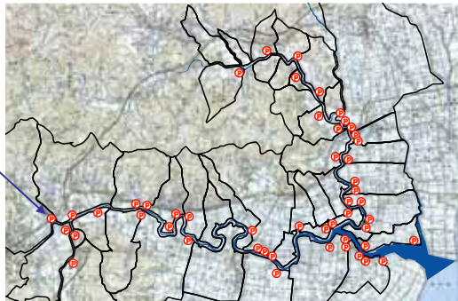
〔既設ポンプ位置図〕
