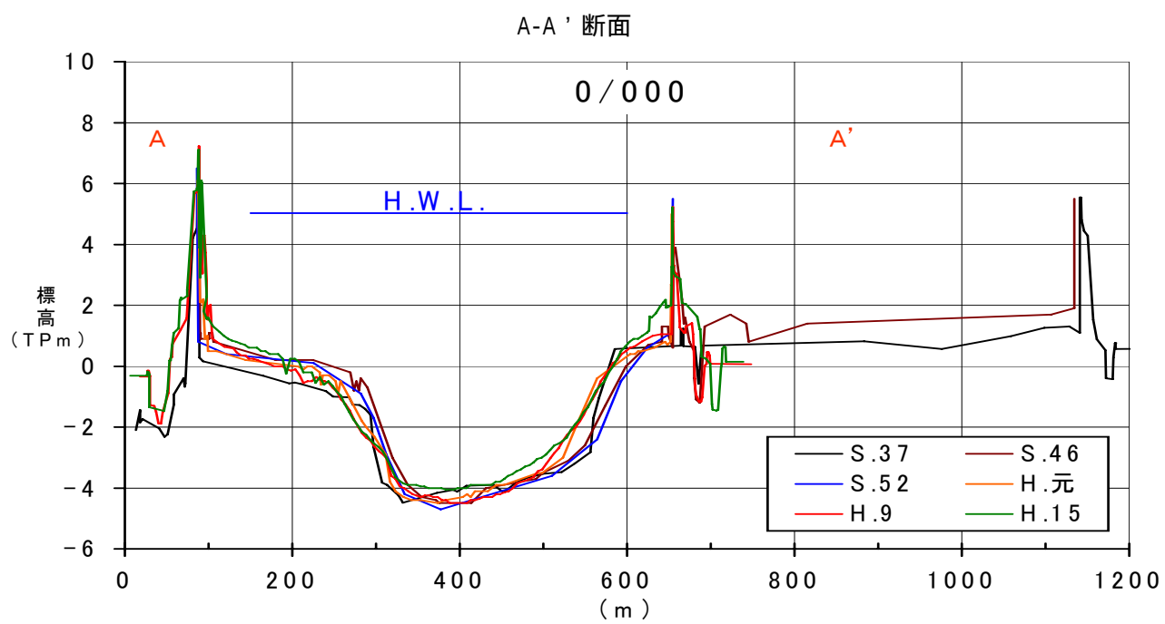
图 3-2 河口部横断变迁图
