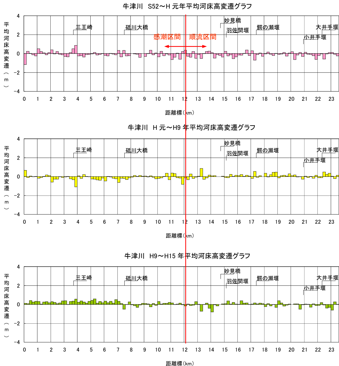
図 2-2 (2) 牛津川の河床変動傾向 (低水路平均河床高)
