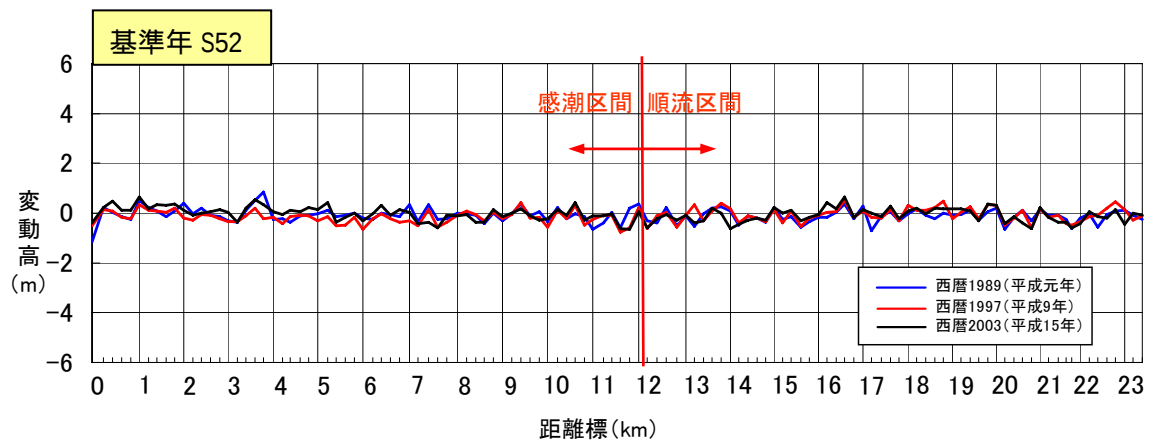
図 2-2 ( 1 ) 六角川低水路平均河床高縦断面図
