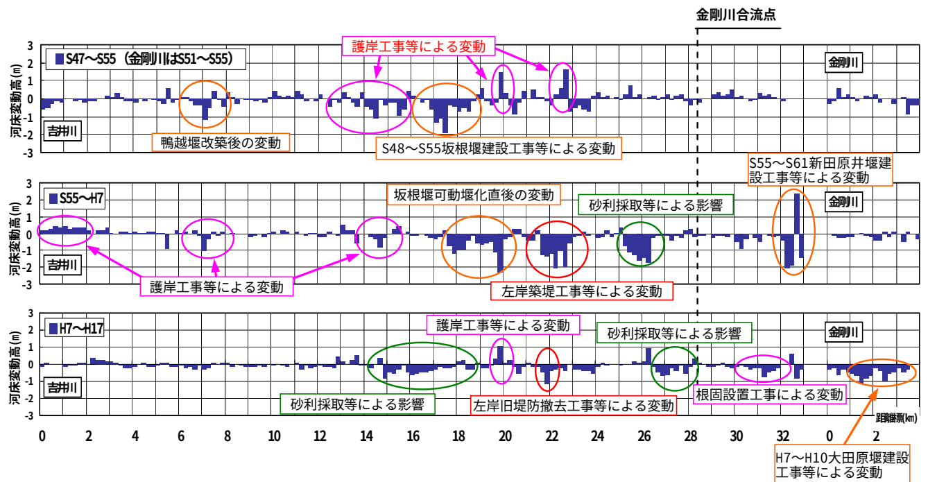
図-8.2.1(1) 吉井川・金剛川 低水路内河床変動量経年変化図
