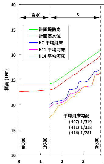
図-8.1.1(2) 吉井川水系平均河床高縦断図(金剛川 0K0~3K8)
