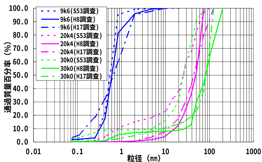
図-8.2.3 粒径加積曲線の経年変化
