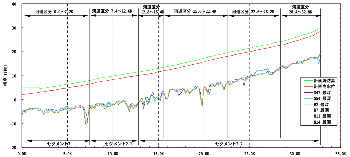
図-8.1.1(1) 吉井川水系平均河床高縦断図(吉井川 0K0~32K8)
