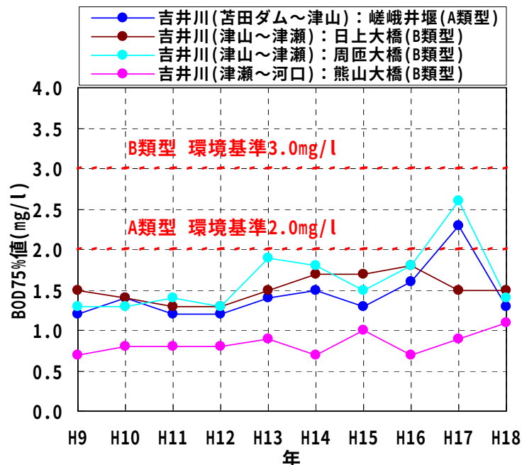
図-6.2.1 主要地点の水質(BOD75%値)経年変化図
