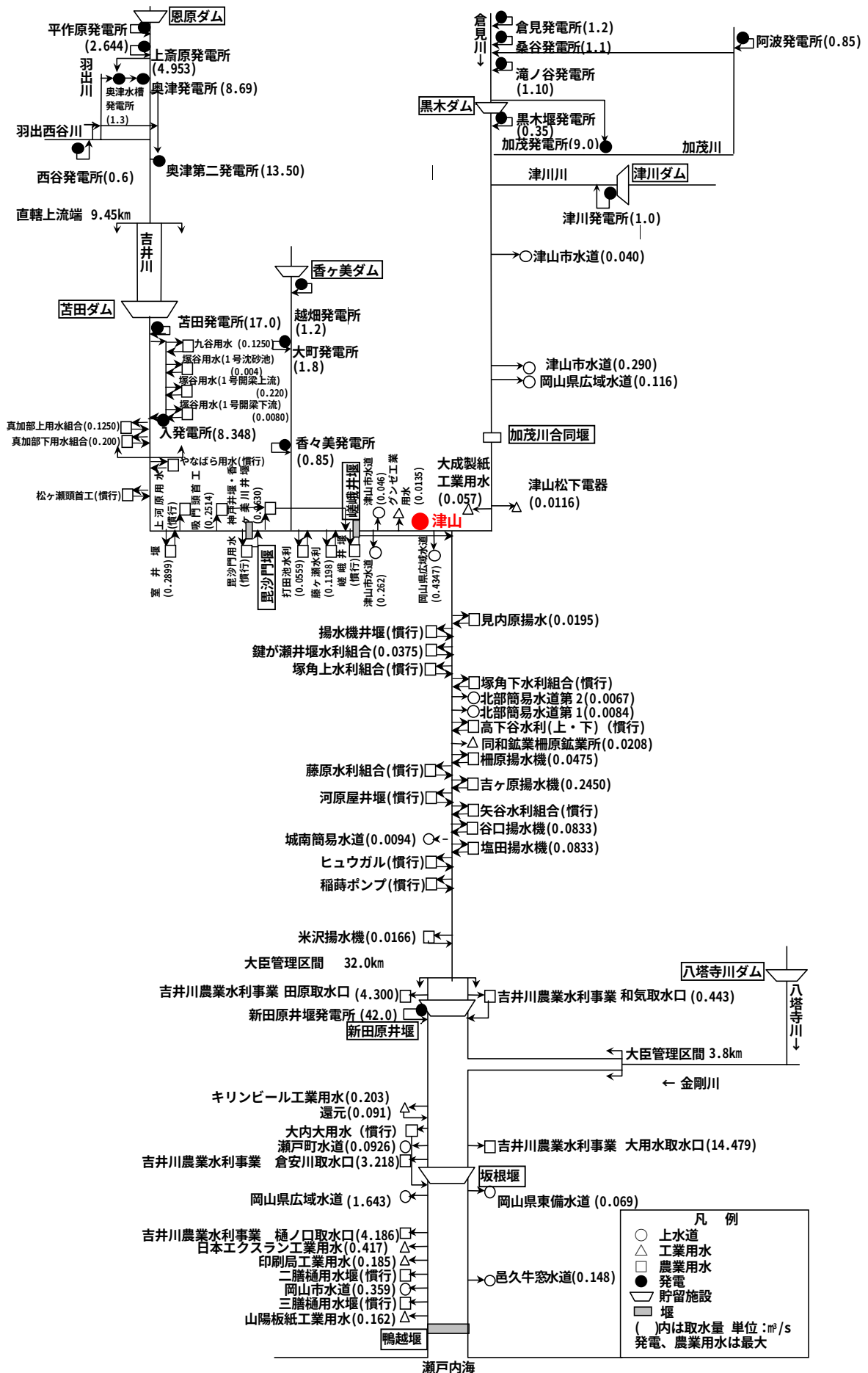
図-5.1.6 水利模式図
