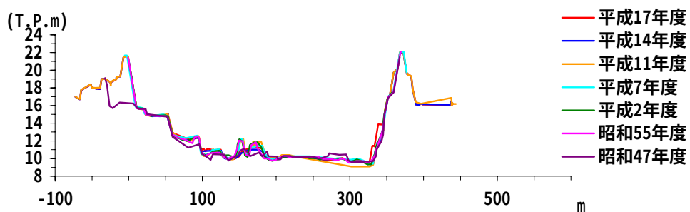
図-8.2.2(2) 河床横断面経年変化図(吉井川：24K800)
