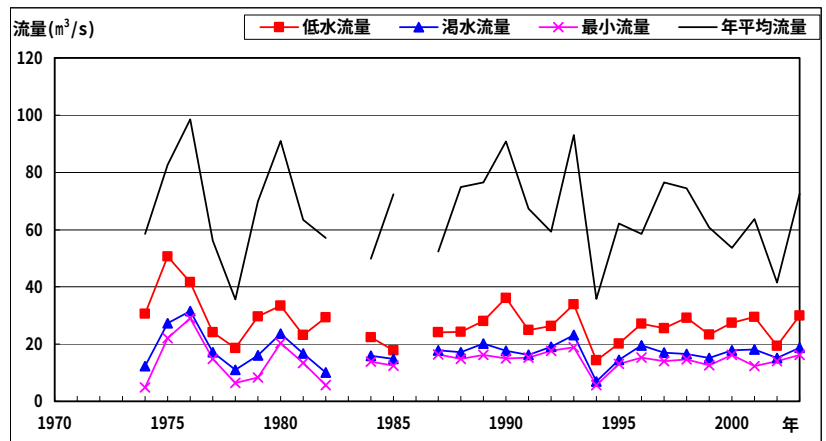
図-5.2.1 津瀬観測所における流況の経年変化
