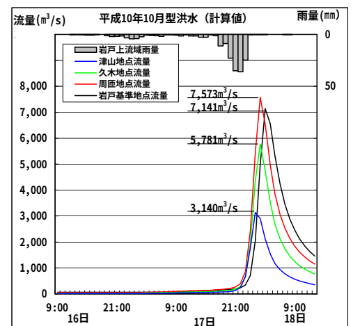
図-4.1.1 平成 10 年 10 月洪水 ハイドロハイトグラフ
