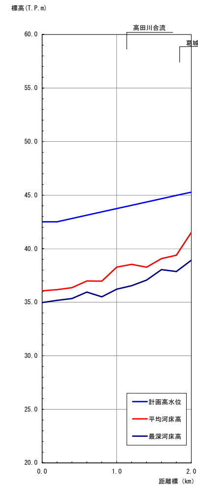
図 7 - 2 佐保川、曾我川、石川計画縦断面図
