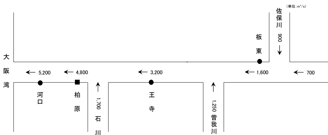
図 6 - 1 大和川計画高水流量図
