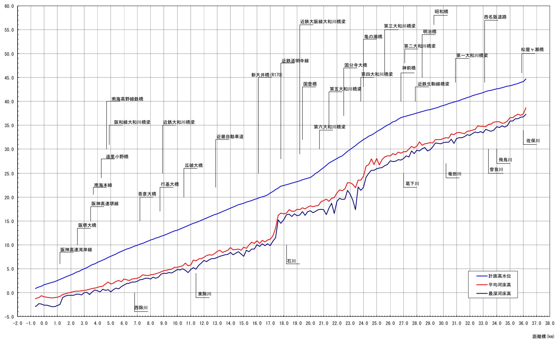
図 7 - 1 大和川計画縦断面図
