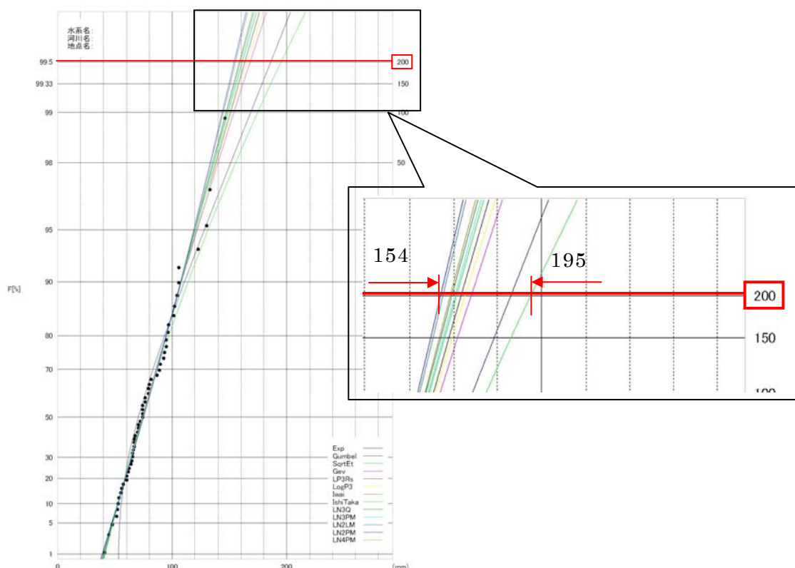
図 4 - 5 柏原地点上流における雨量確率評価（昭和28年～平成19年：55ヵ年）
