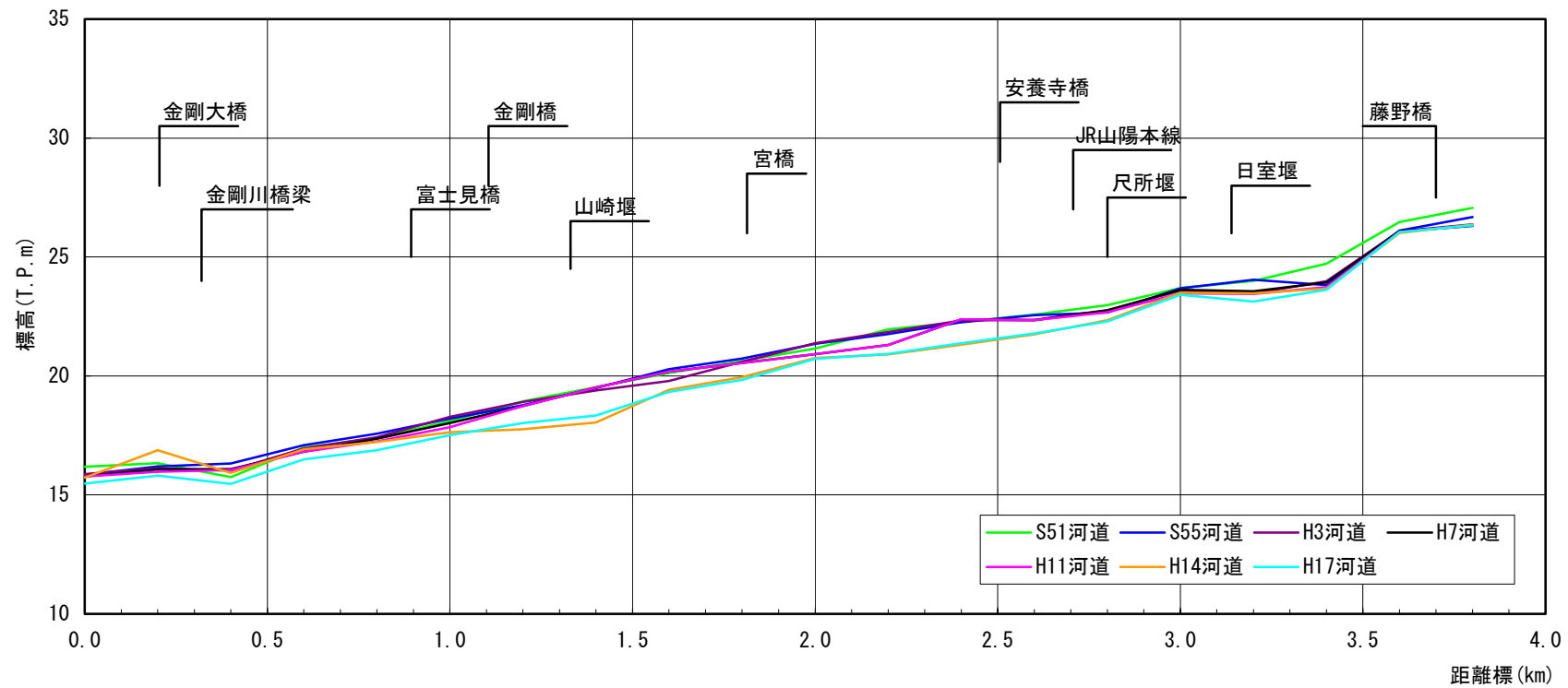
図 2-3 低水路平均河床高縦断図(金剛川)
