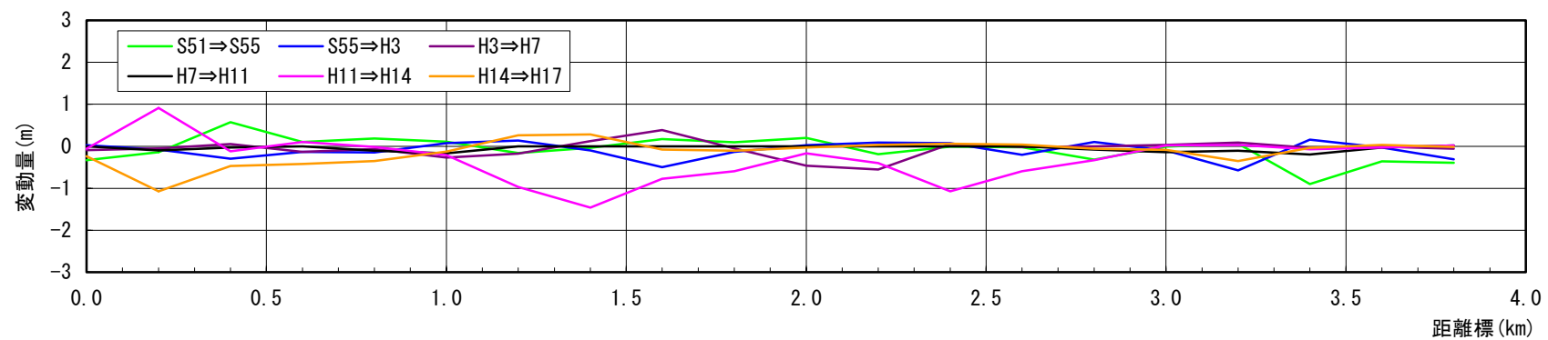
図 2-4 平均河床変動量縦断図(金剛川)
