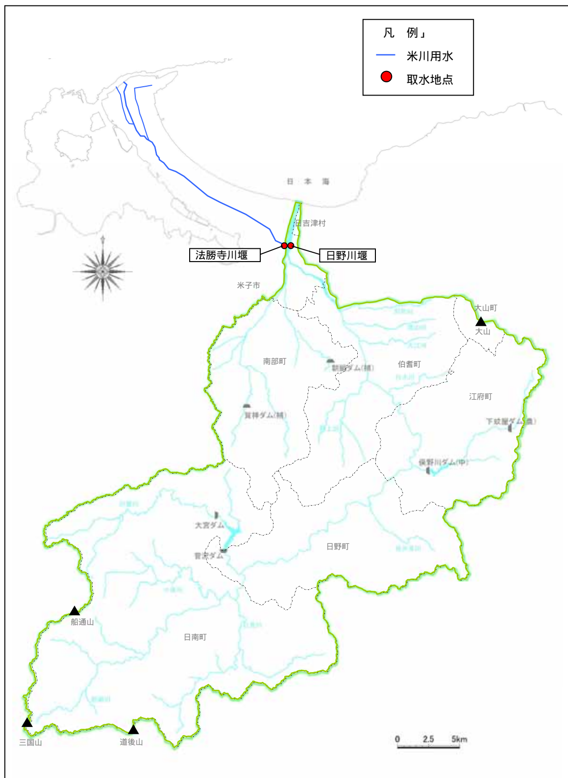
図 5.1.5 米川用水
