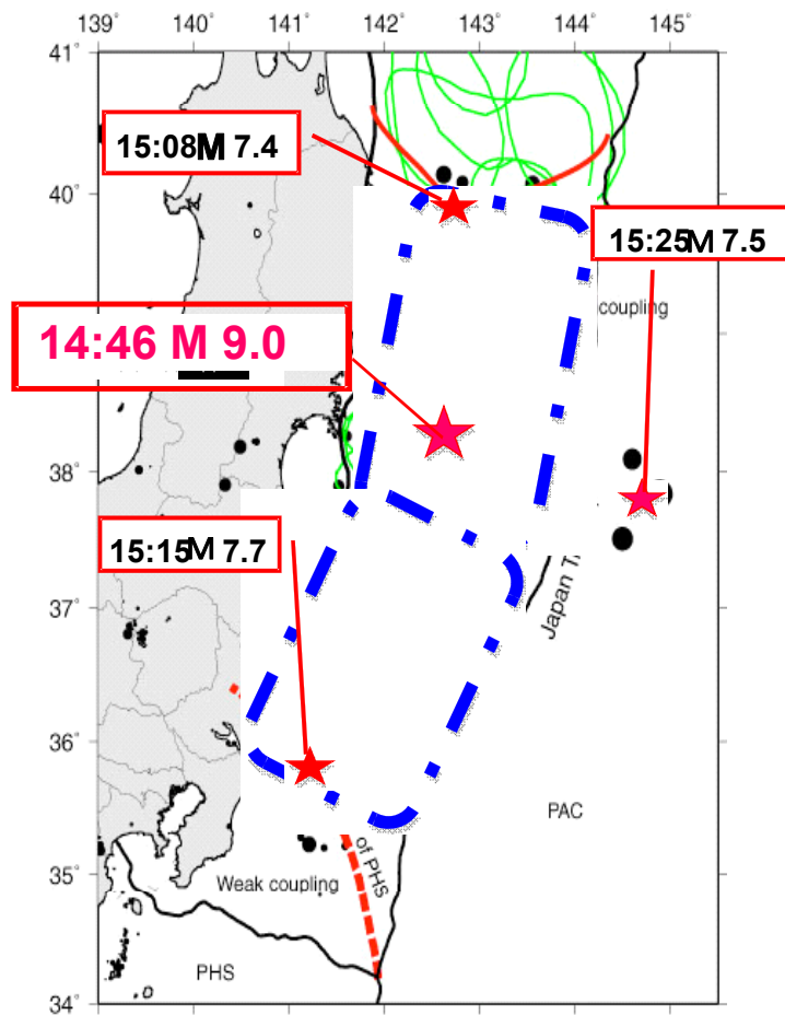
震源分布とそのマグニチュード
