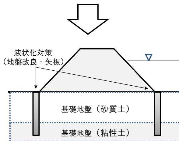
地盤改良・矢板による 耐震・液状化対策
