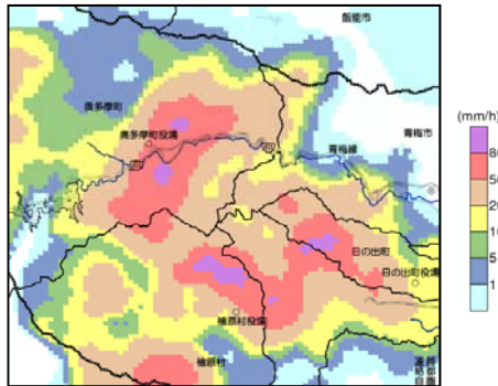
XバンドMPLレーダによる雨量観測
