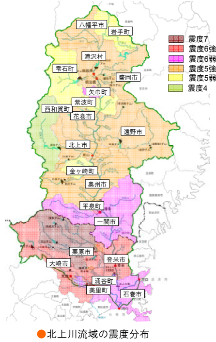
●北上川流域の震度分布
