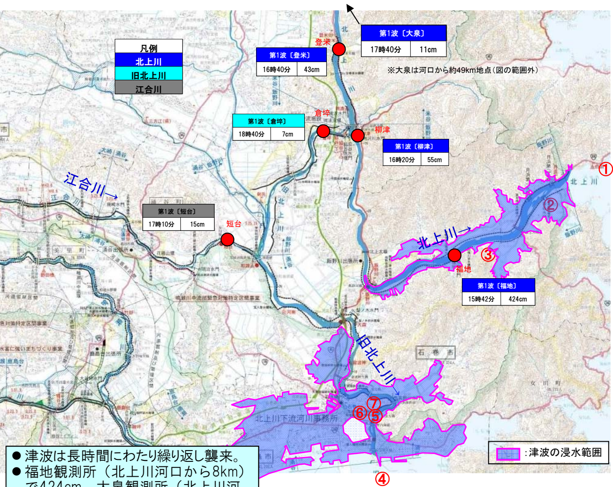
津波の浸水及び遡上範囲
