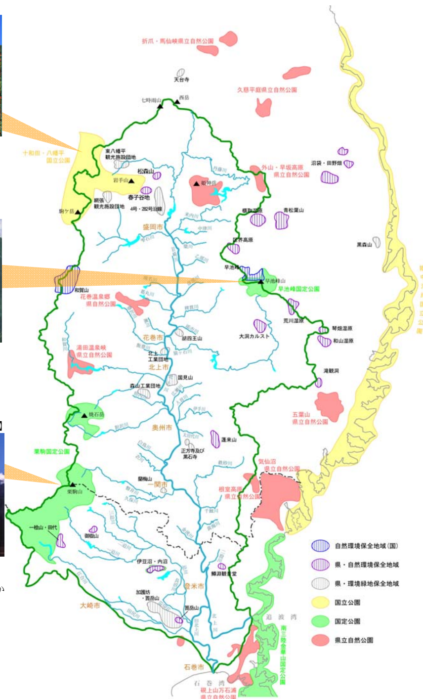
図 2-7 北上川流域の自然公園
