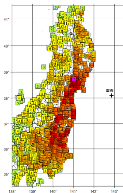
図 4-18 震度分布図
