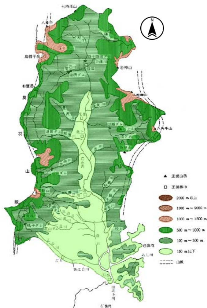
図 1-3 北上川流域 地形図
