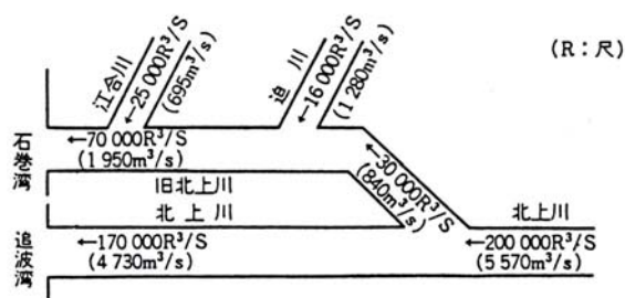
図 4-3 北上川下流部当初計画 流量配分図
