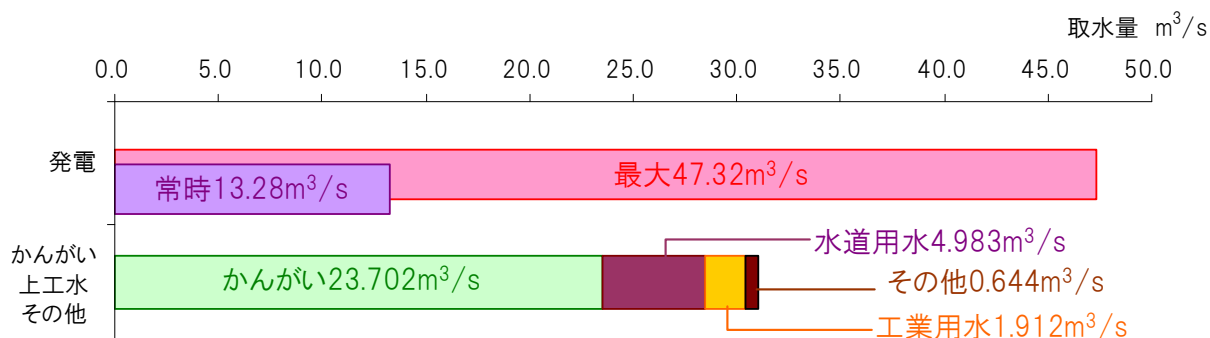
図 5-1-3 名取川水系における目的別水利流量
