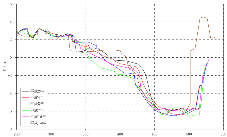
図 8-3-5 名取川河口部（-0.6k）の横断図
