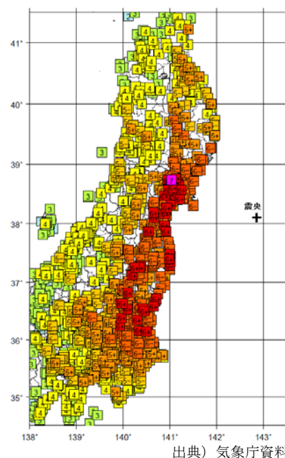
図 4-3-1 震度分布図
