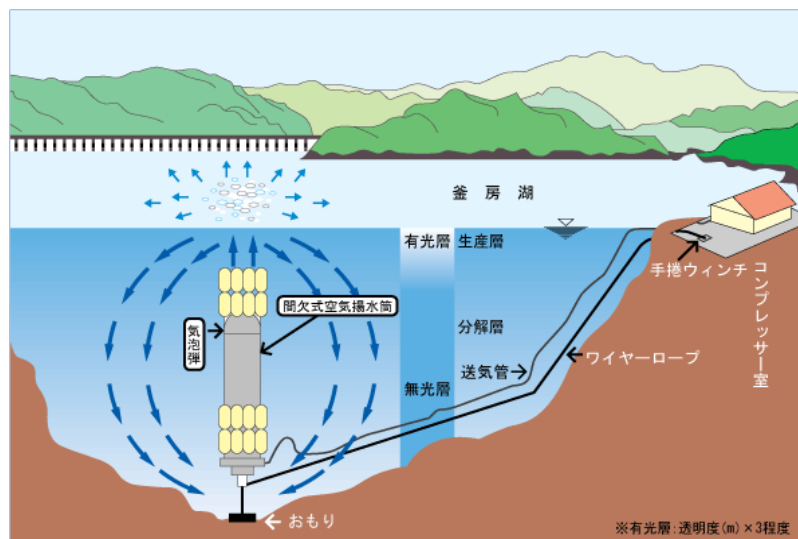
▲釜房ダムの曝気循環システム
