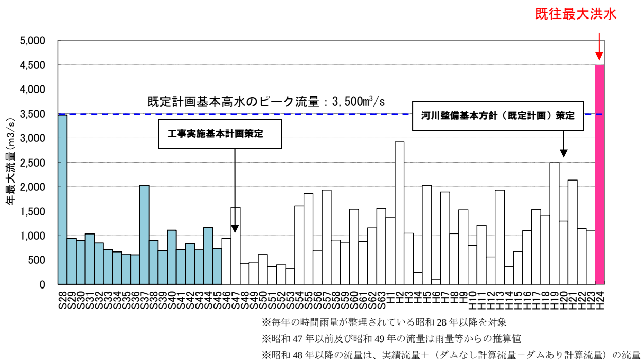
図 4-1 年最大流量（基準地点船小屋）
