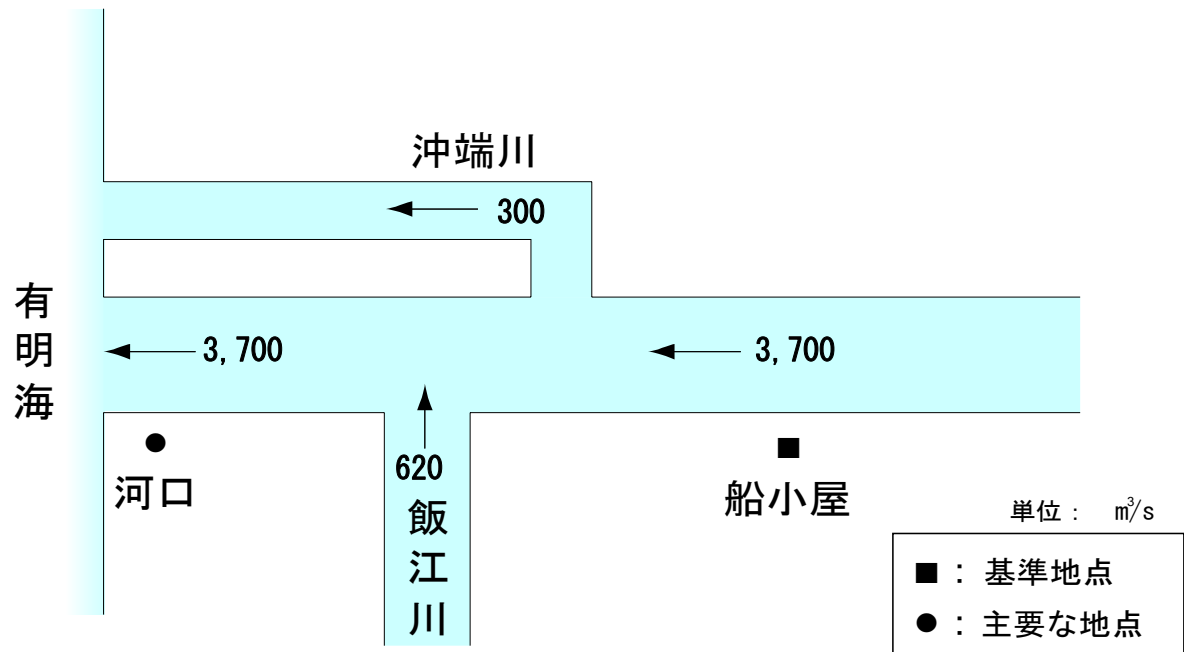
図 6-1 矢部川計画高水流量図 基本方針（案）
