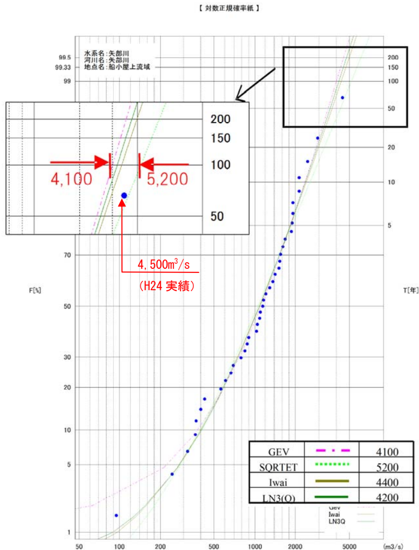
図 4-3 船小屋地点における流量確率評価 (昭和 48 年～平成 24 年：40 年間)
