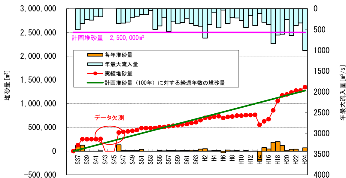
図 3-1 日向神ダムの堆砂状況
