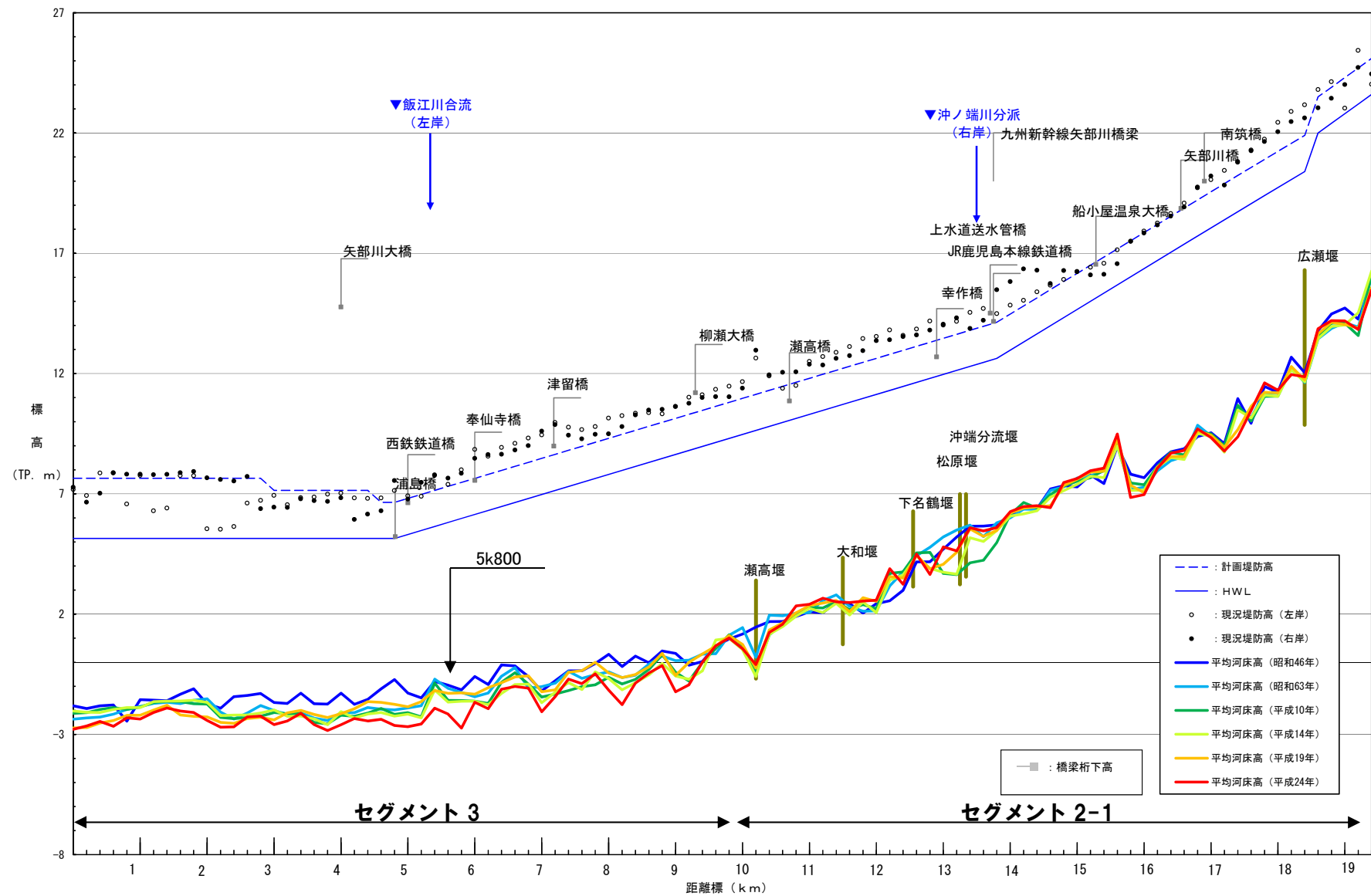
図 2-2 (1) 矢部川平均河床高縦断図 (昭和 46 年～平成 24 年)
