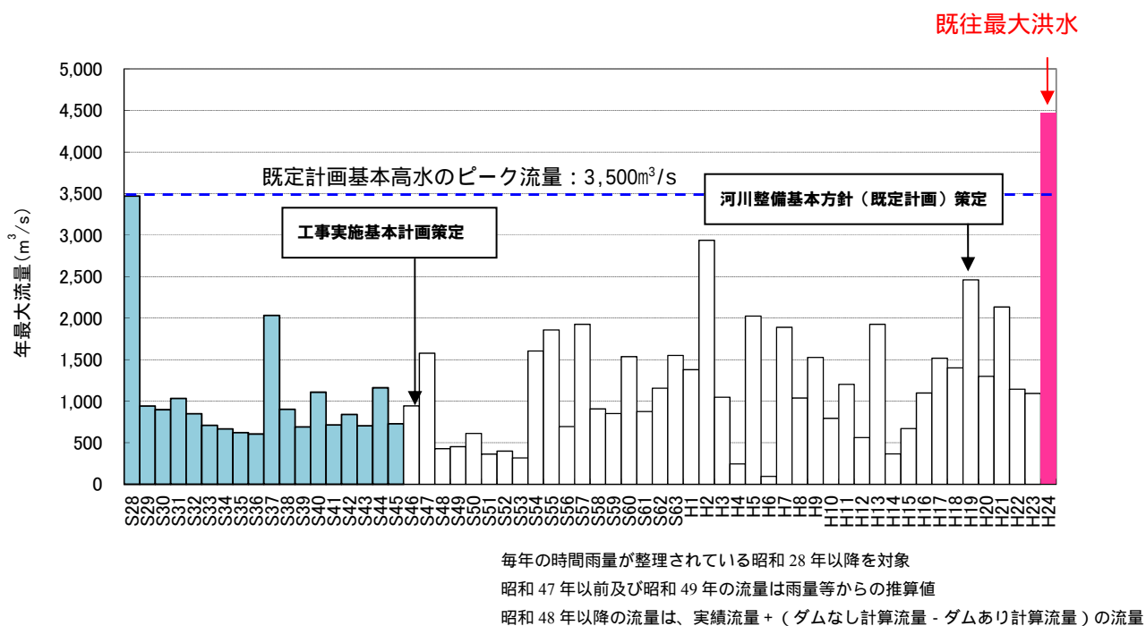
図 4-1 年最大流量（基準地点船小屋）
