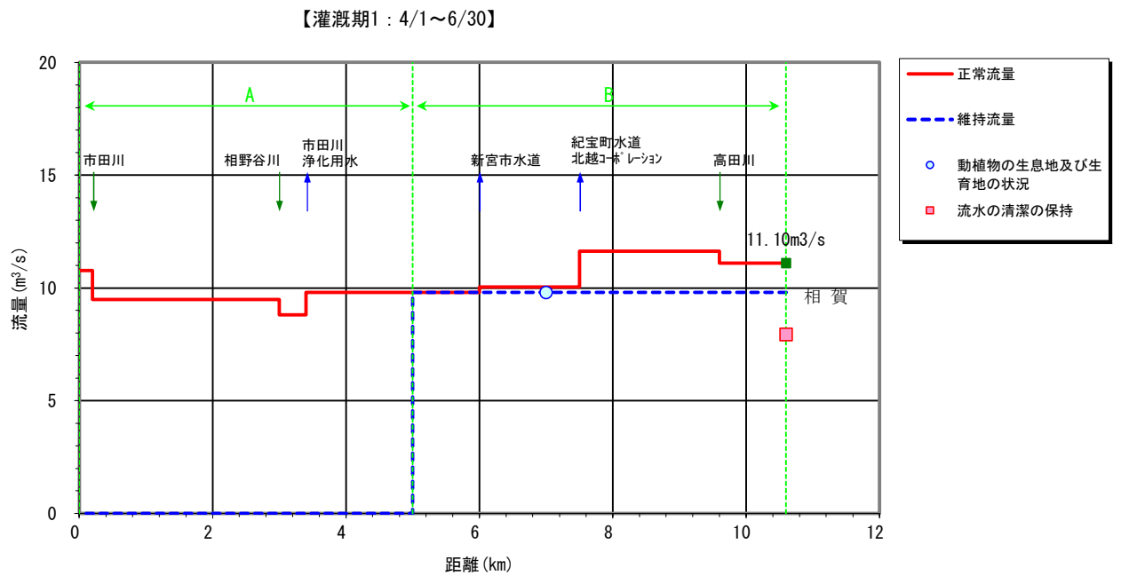
図 6-1 (2) 熊野川の正常流量(灌漑期 : 4/1~6/30 (期間 2) )
