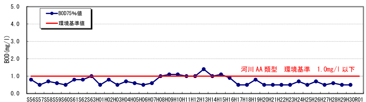
BOD の経年変化(四滝) 河川 A A 類型
