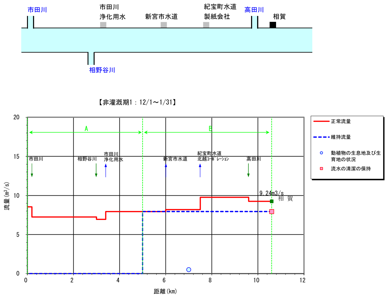
図 6-1 (7) 熊野川の正常流量(非灌漑期：12/1～1/31 (期間 7) )
