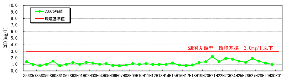
COD の経年変化(坂本ダム湖取水口) 湖沼A類型
