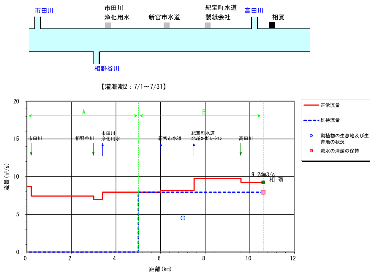
図 6-1 (3) 熊野川の正常流量(灌漑期 : 7/1~7/31 (期間 3) )
