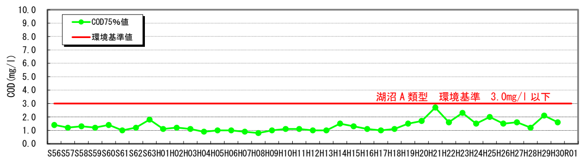
COD の経年変化(池原ダム湖取水口) 湖沼A類型
