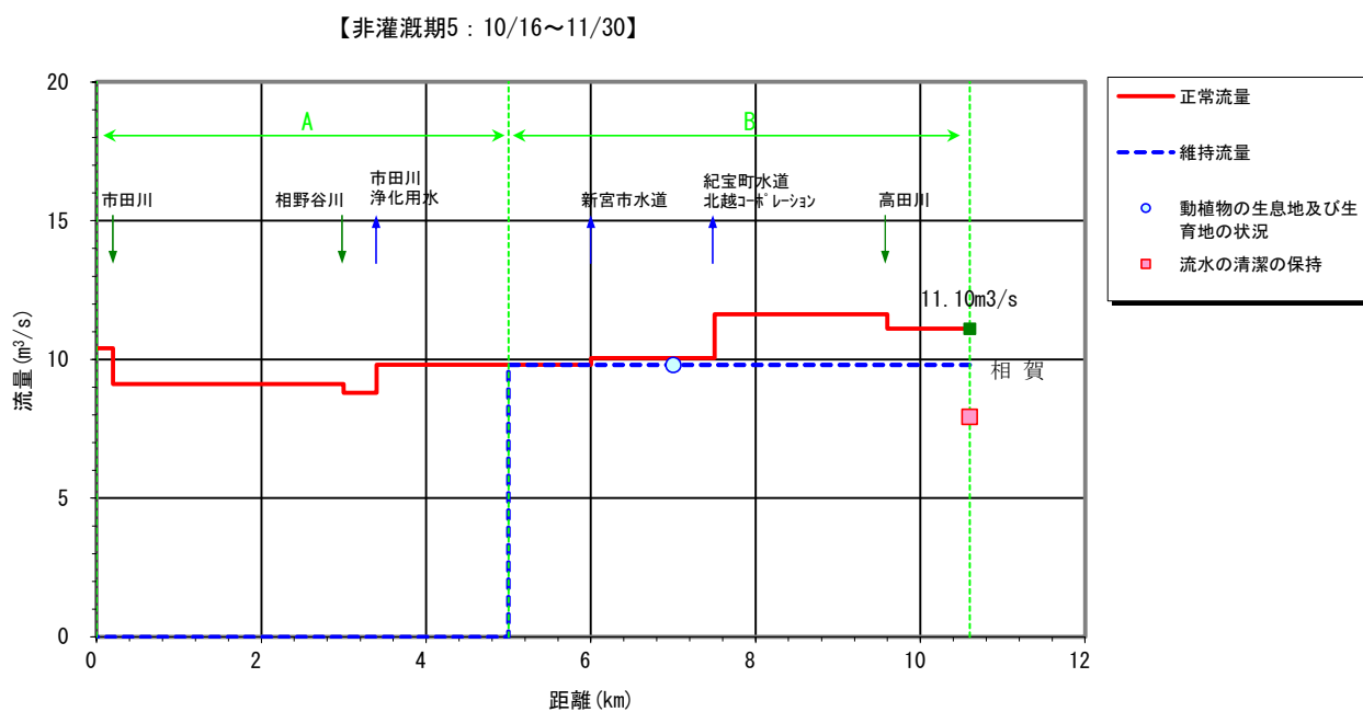
図 6-1 (6) 熊野川の正常流量(非灌漑期 : 10/16~11/30 (期間 6) )
