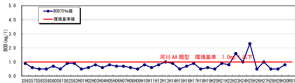
BOD の経年変化(北山大橋) 河川 A A 類型
