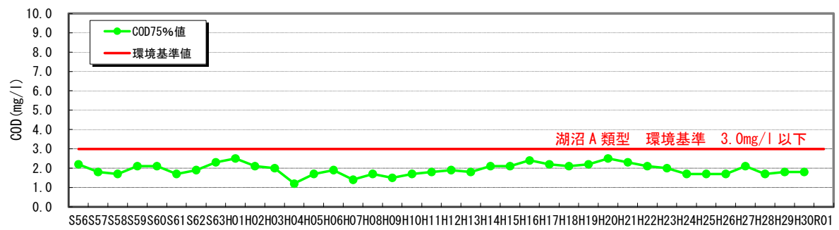
COD の経年変化(猿谷ダム湖取水口) 湖沼A類型
