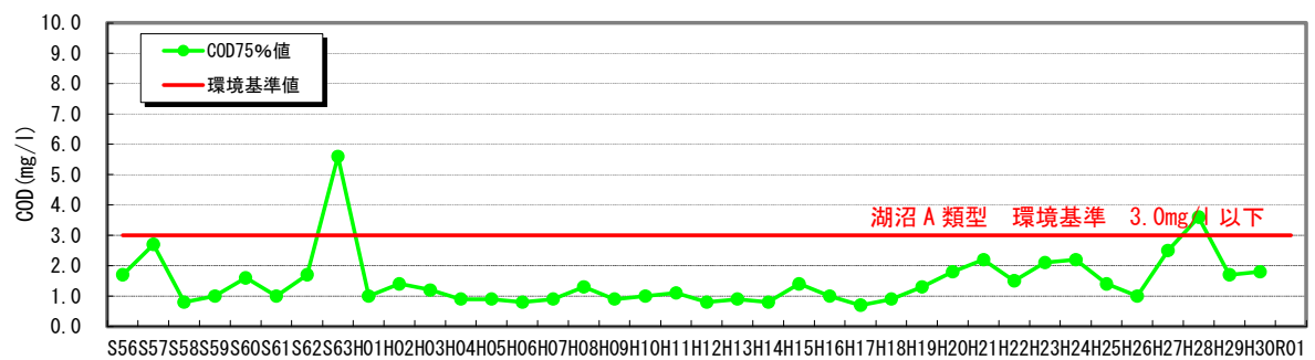
COD の経年変化(風屋ダム湖取水口) 湖沼A類型
