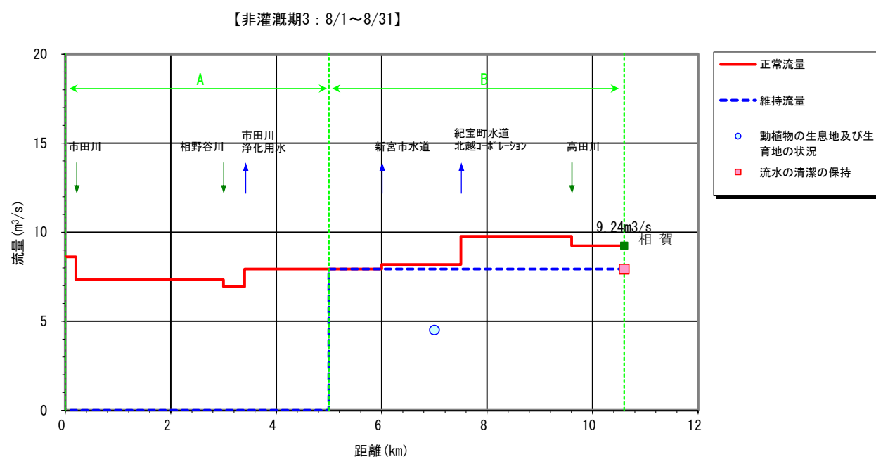
図 6-1 (4) 熊野川の正常流量 (非灌漑期 : 8/1~8/31 (期間 4) )
