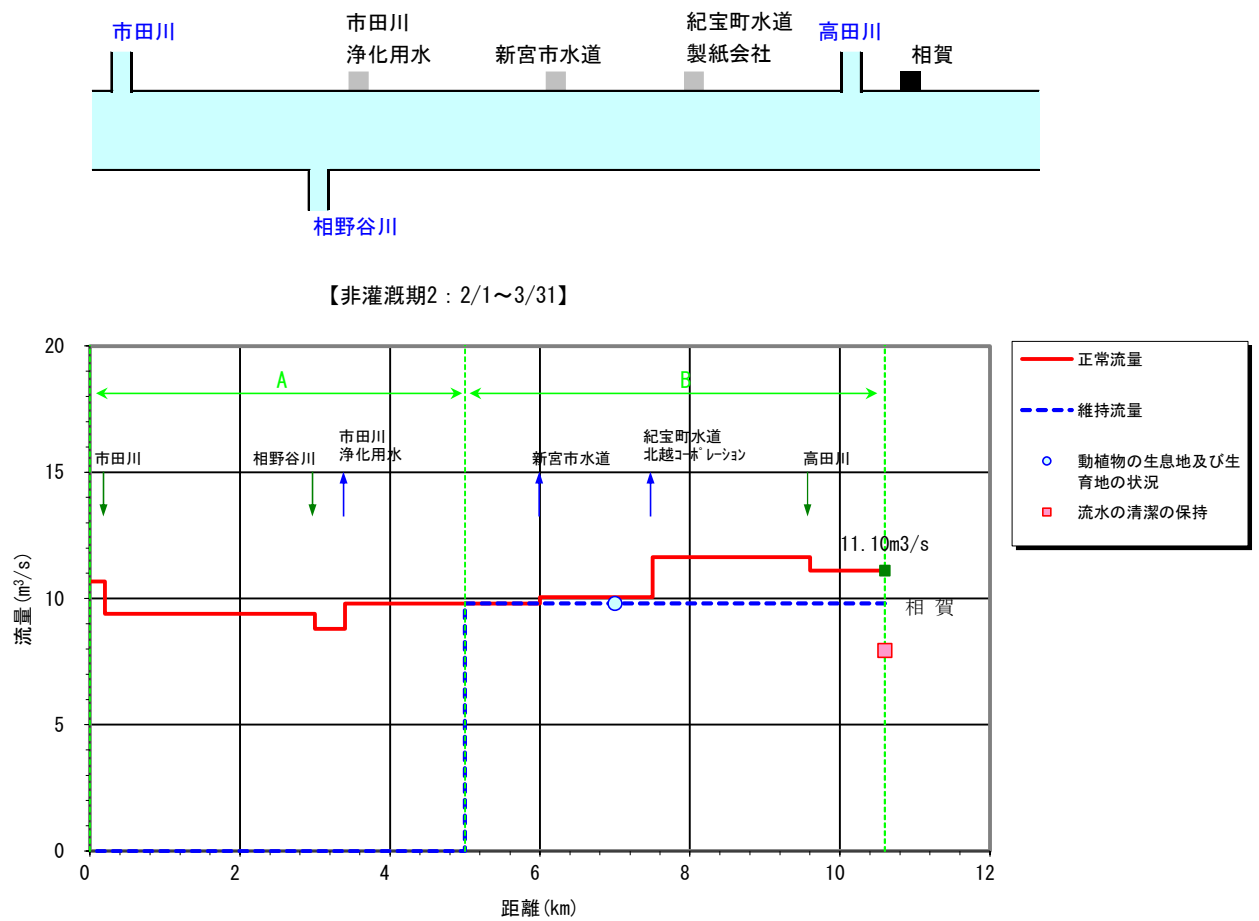
図 6-1 (1) 熊野川の正常流量(非灌漑期 : 2/1~3/31 (期間 1) )
