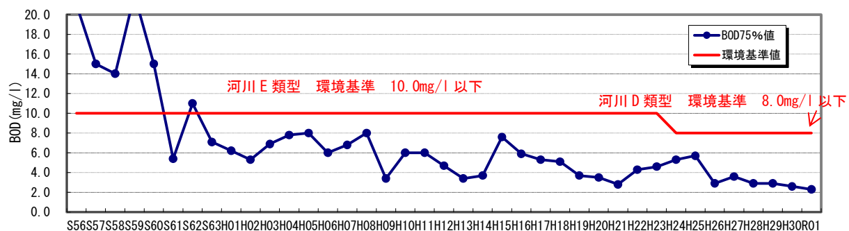
BOD の経年変化(貯木橋) 河川 D 類型
