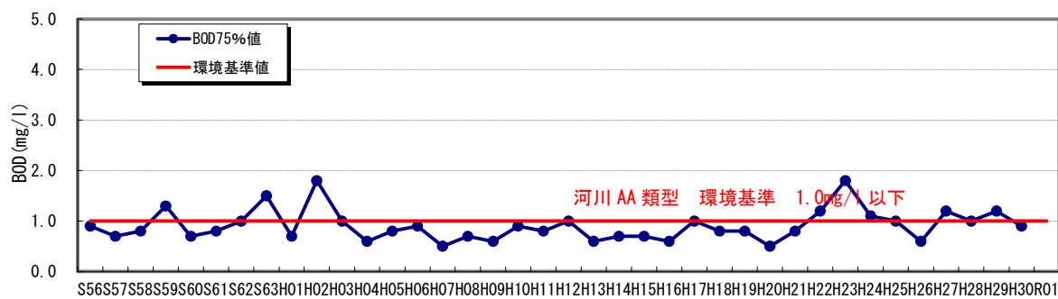
BOD の経年変化(小口橋) 河川 A A 類型
