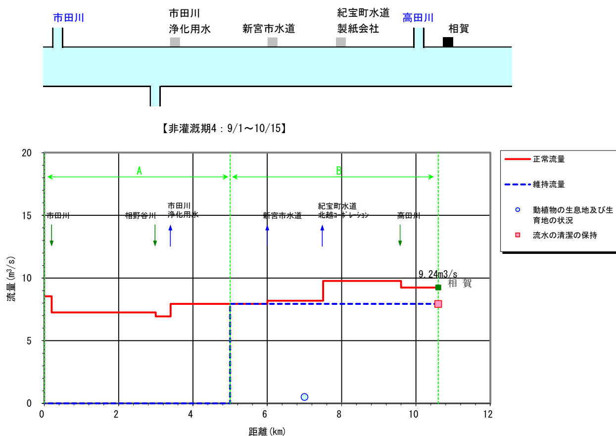
図 6-1 (5) 熊野川の正常流量(非灌漑期 : 9/1~10/15 (期間 5) )
