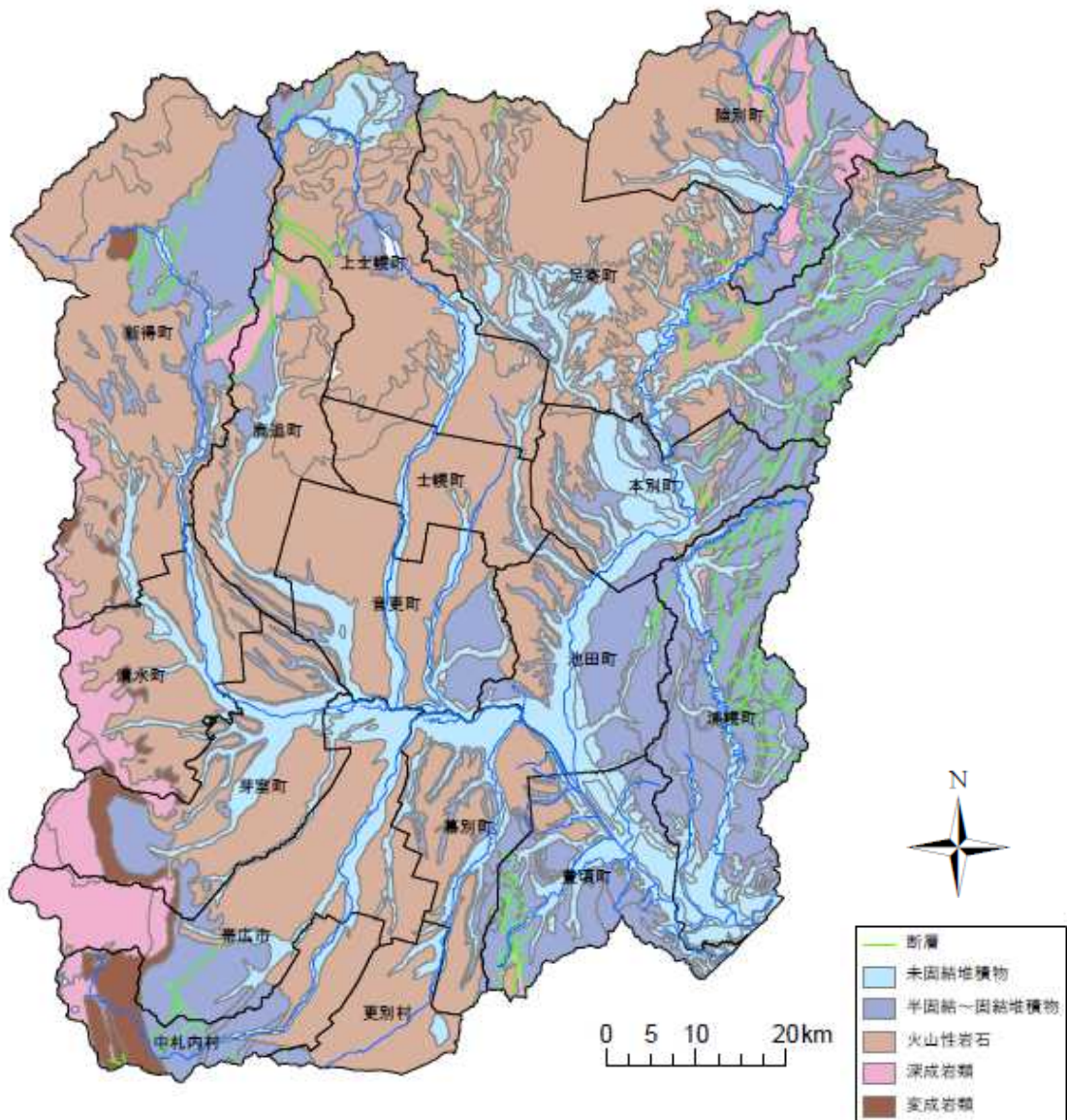
図 1-3 表層地質図
