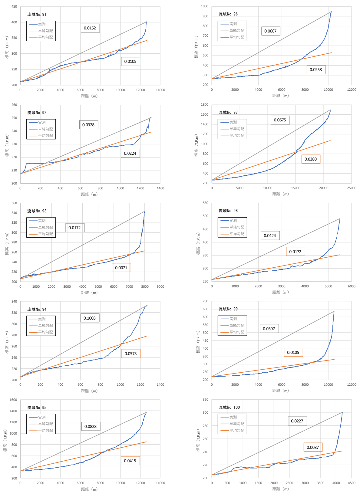
图 1-28 (10) 流域流路勾配
