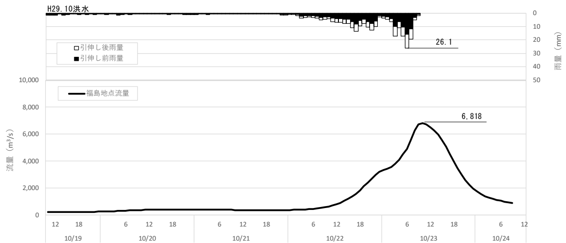
図 1-46 (22) 対象降雨の降雨 36hr 拡大による流出計算結果 (H29.10 洪水、福島地点)
