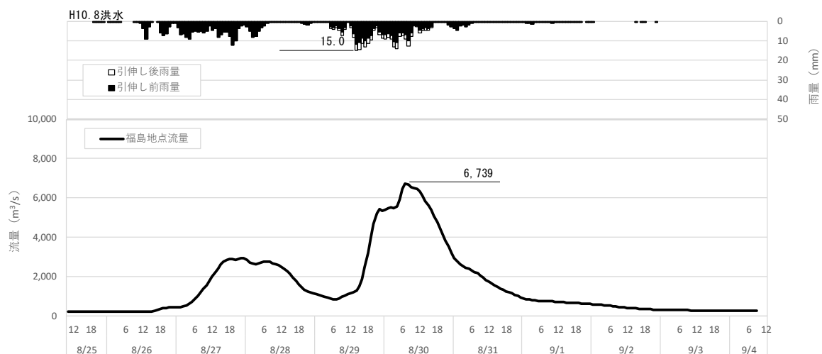
図 1-46 (13) 対象降雨の降雨 36hr 拡大による流出計算結果 (H10.8 洪水、福島地点)
