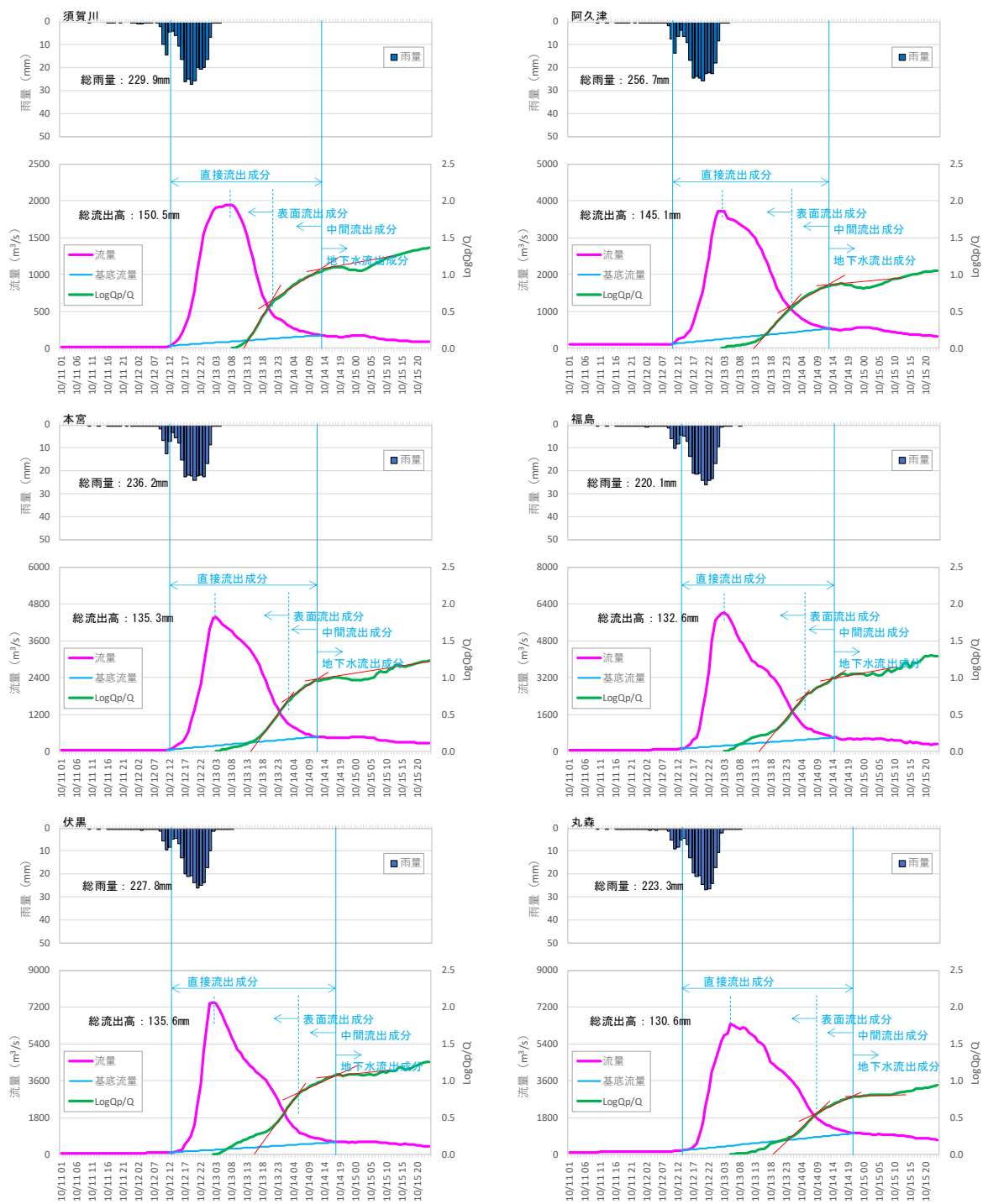
図 1-17 (1) 成分分離の事例 (R1.10 洪水)
