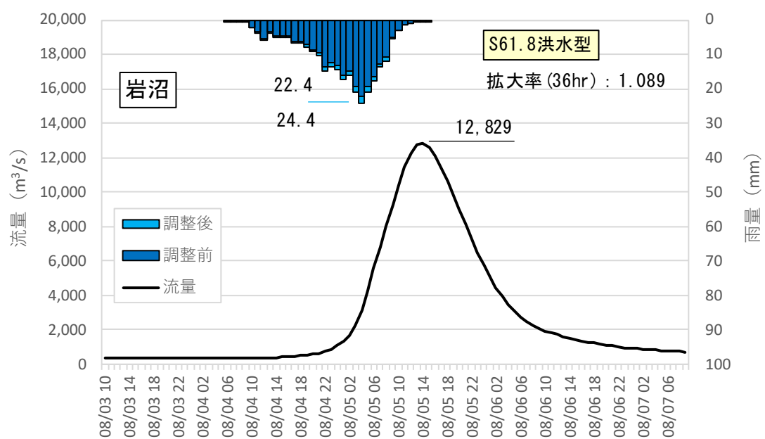
図 1-57 基本高水決定 基準地点流量波形
