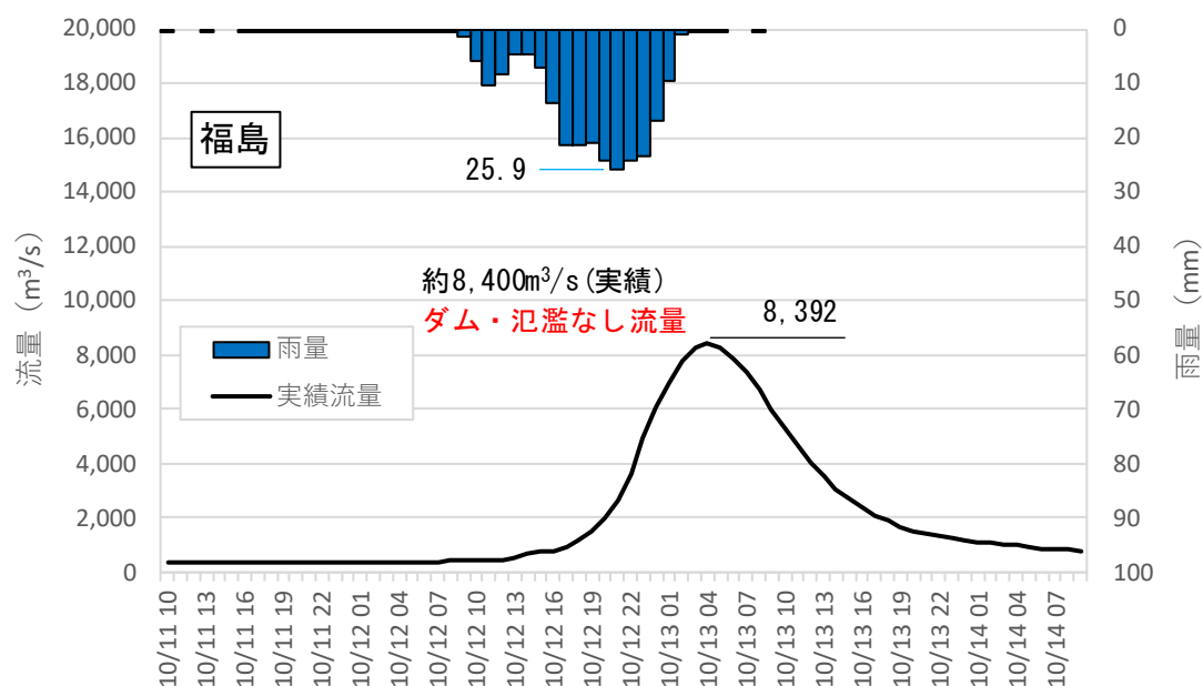
図 1-53 (1) 令和元年 10 月洪水実績流量（基準地点福島）
