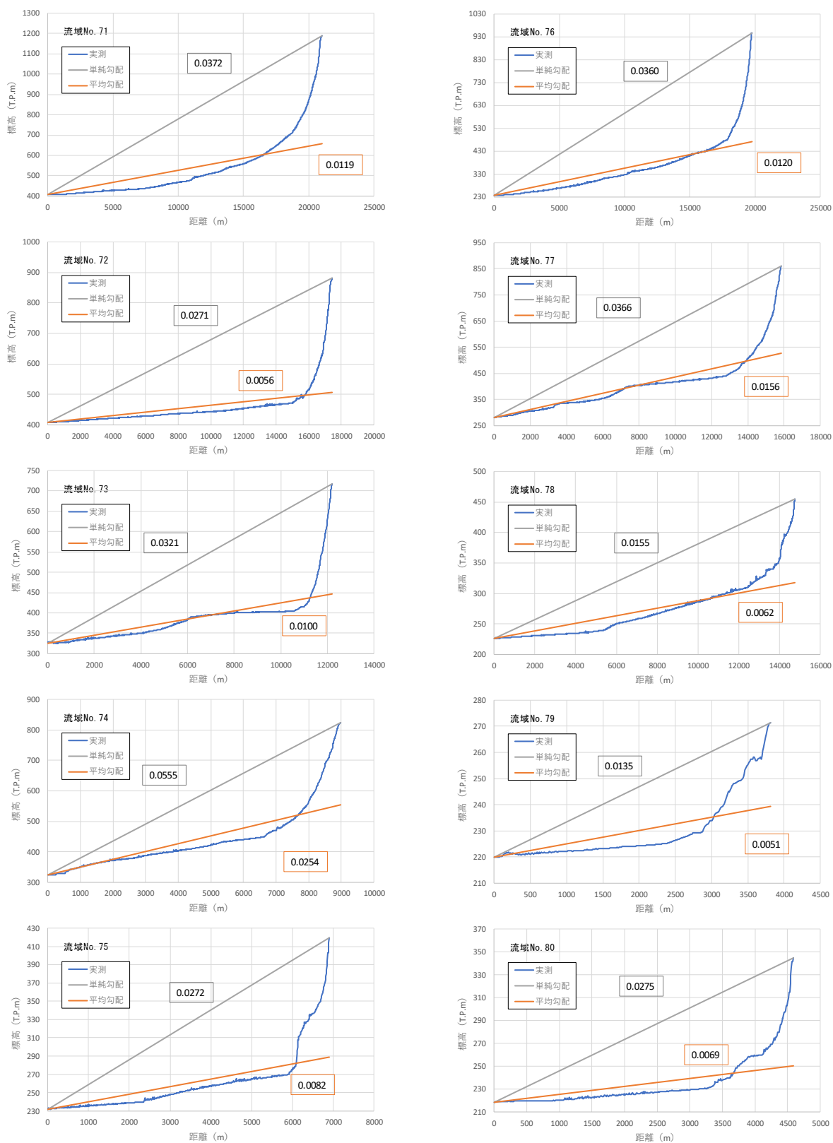
图 1-28 (8) 流域流路勾配
