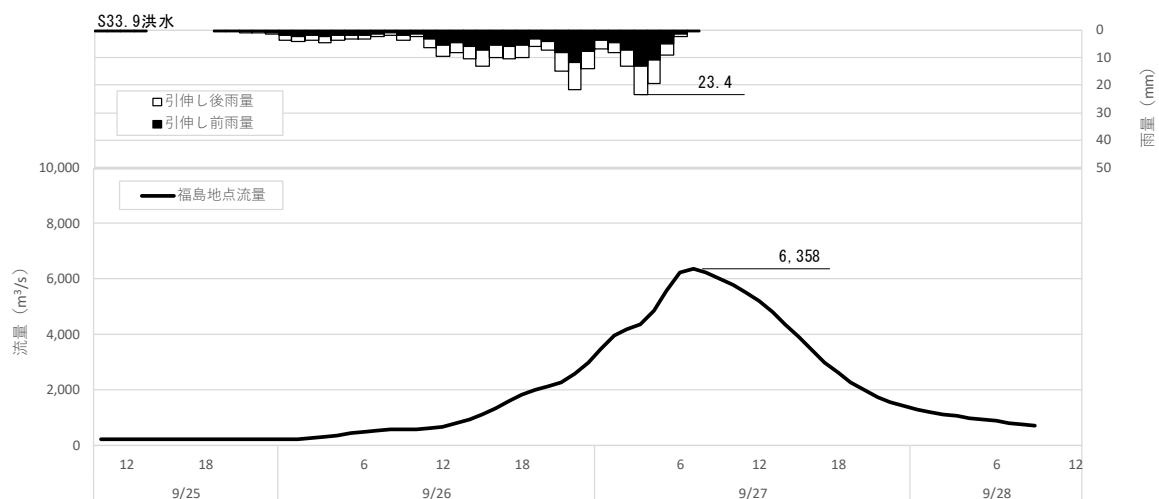
図 1-46 (1) 対象降雨の降雨 36hr 拡大による流出計算結果 (S33.9 洪水、福島地点)
