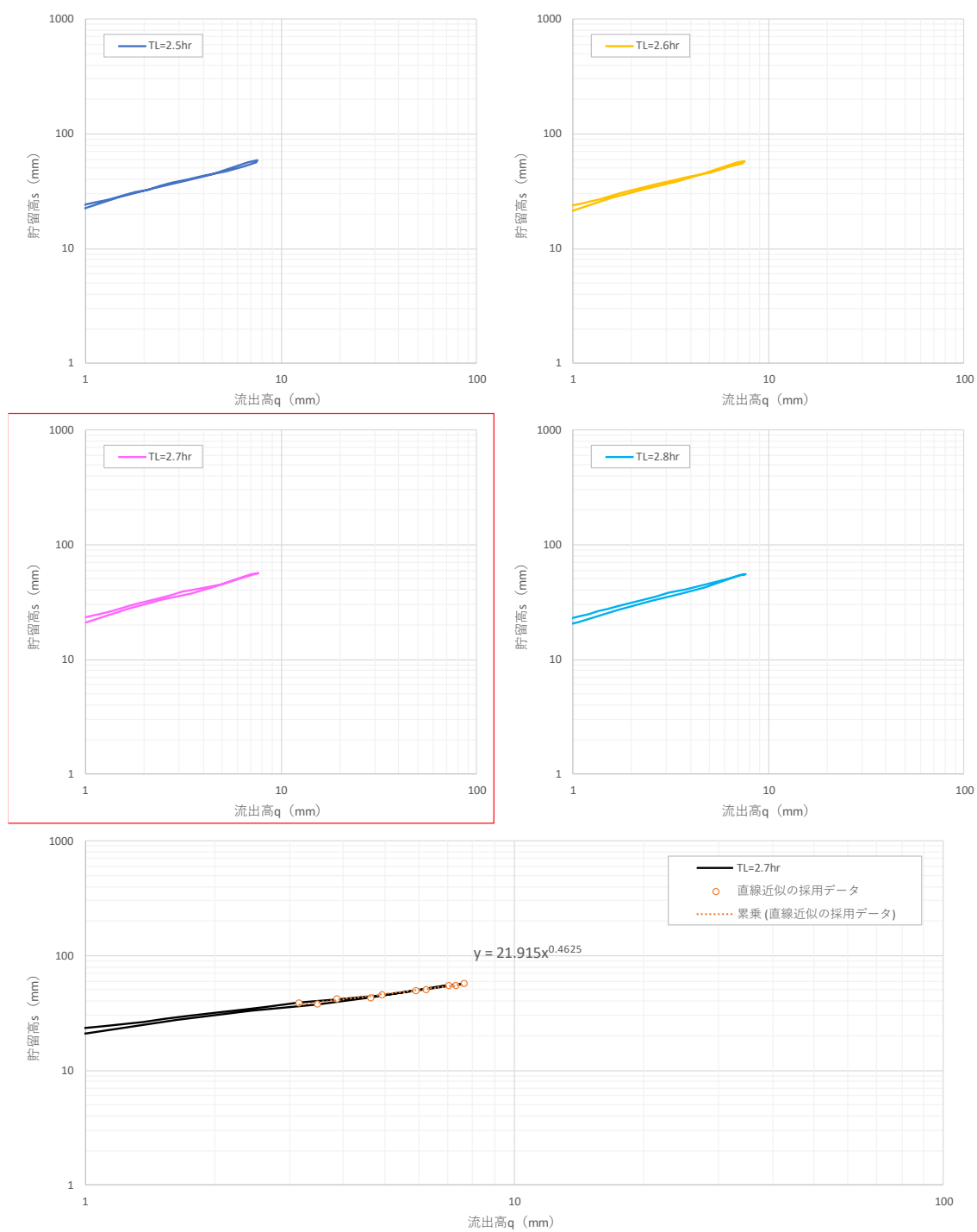
図 1-21 (3) 貯留高－流出高関係図（七ヶ宿ダム地点：R1.10 洪水）
