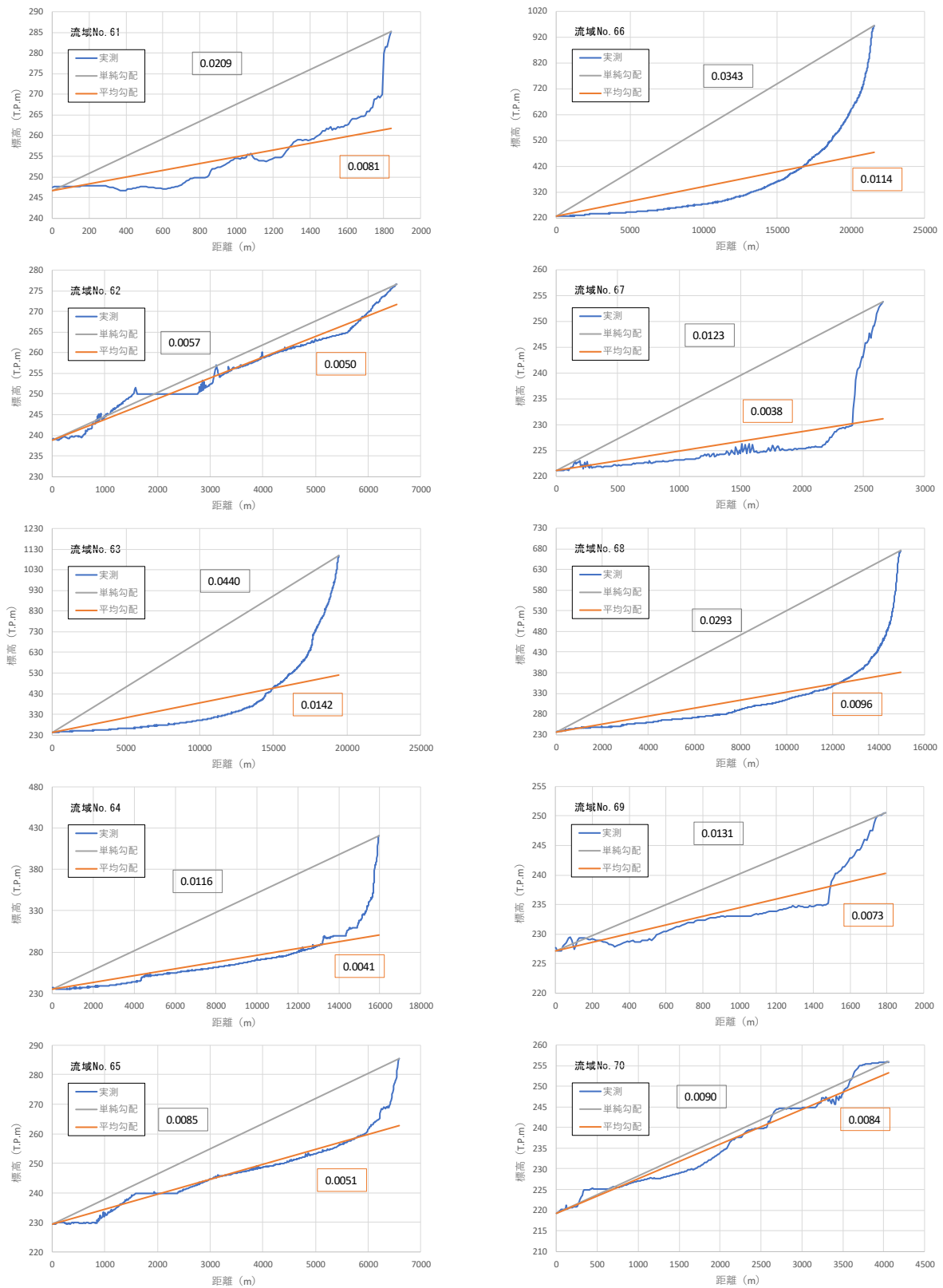
图 1-28 (7) 流域流路勾配
