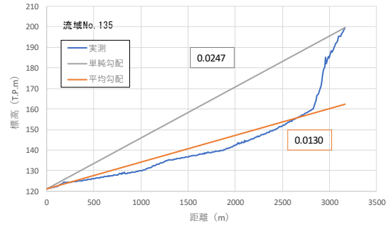
图 1-28 (14) 流域流路勾配
