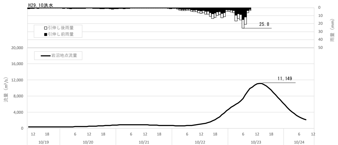
図 1-46 (23) 対象降雨の降雨 36hr 拡大による流出計算結果 (H29.10 洪水、岩沼地点)
