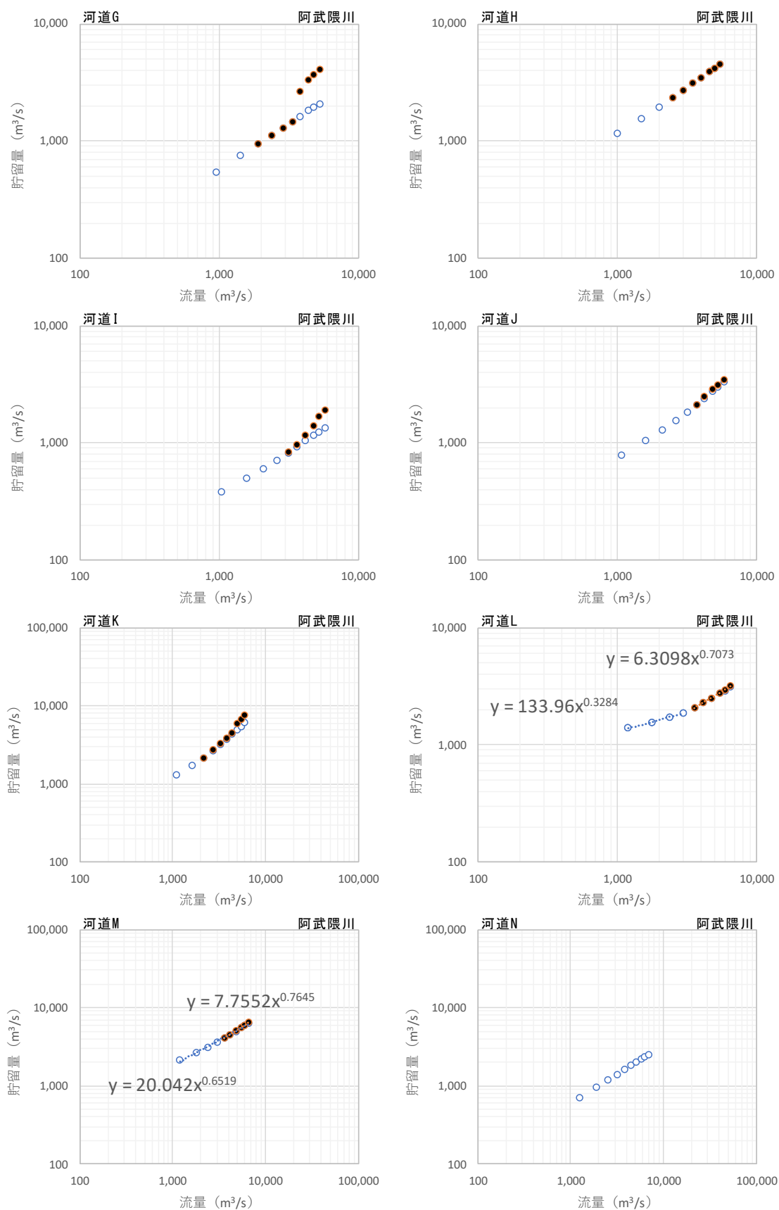
図 1-29 (3) S-Q 関係図
