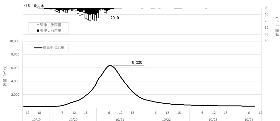
図 1-46 (18) 対象降雨の降雨 36hr 拡大による流出計算結果 (H16.10 洪水、福島地点)
