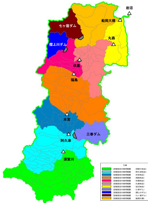
図 1-15 f1、Rsa 検討対象流域
