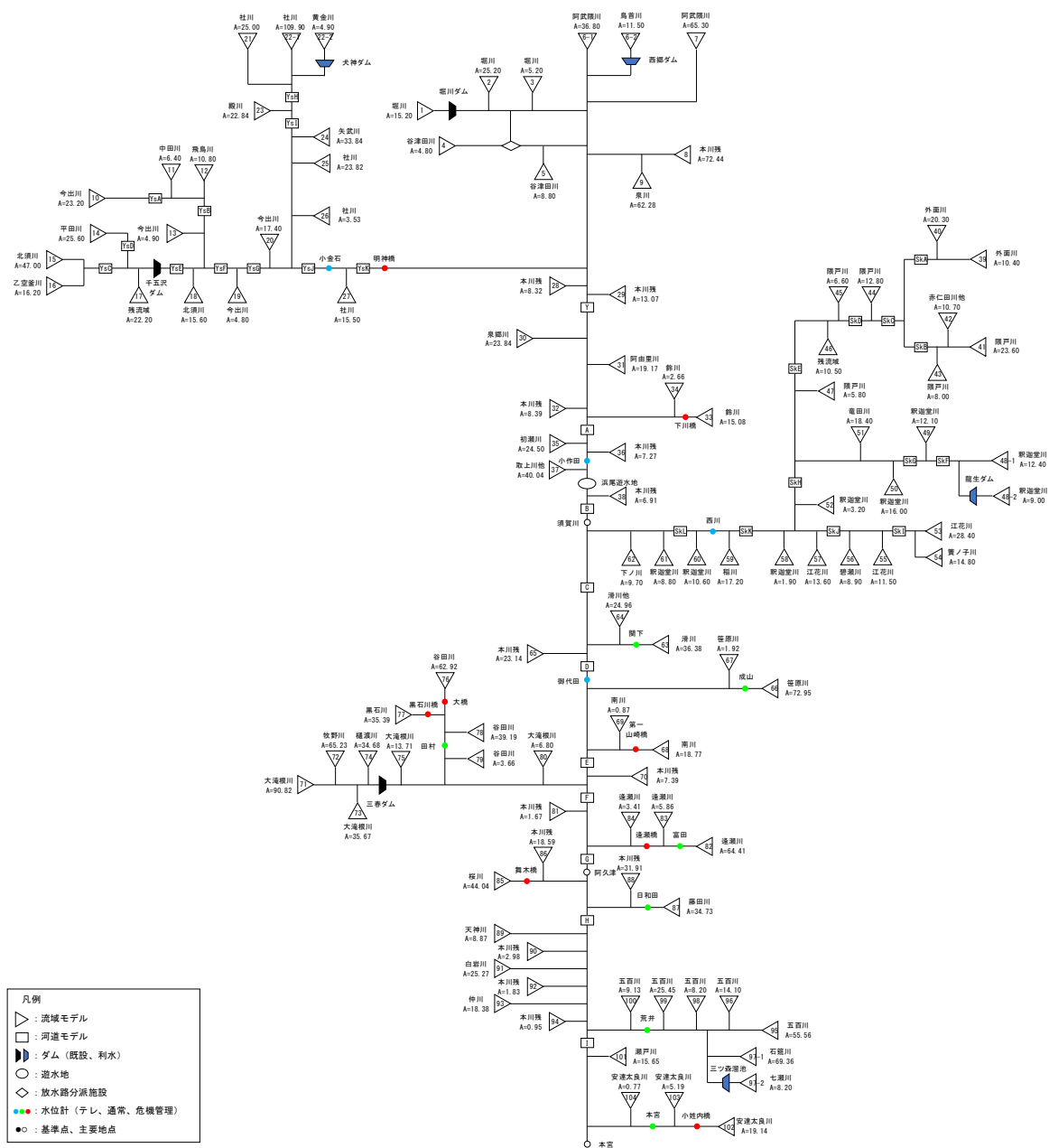
図 1-33 (1) 流出計算模式図
