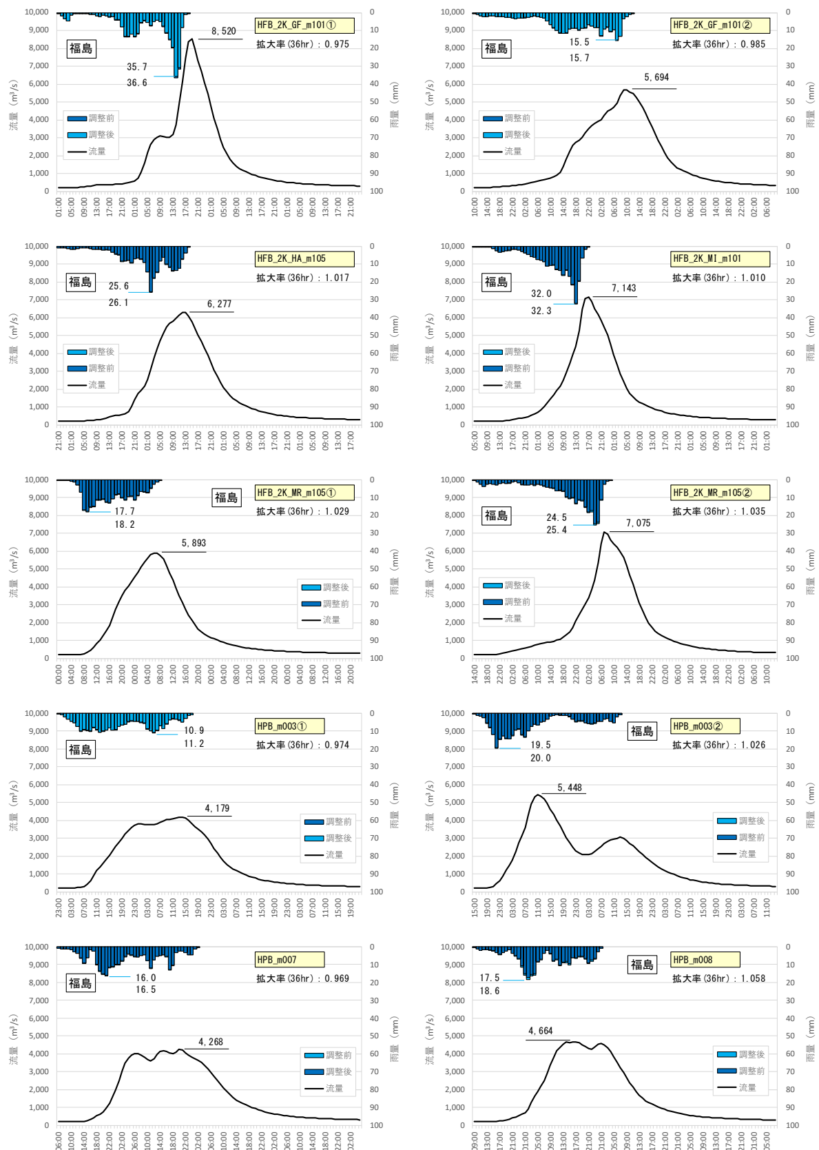
図 1-49 (1) アンサンブル予測降雨波形による流出計算結果（福島地点）
