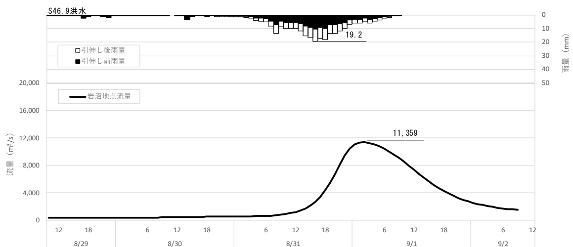
図 1-46 (5) 対象降雨の降雨 36hr 拡大による流出計算結果 (S46.9 洪水、岩沼地点)
