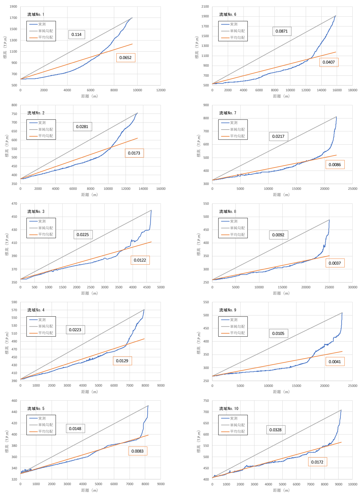
图 1-28 (1) 流域流路勾配
