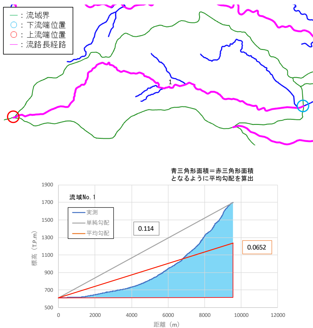
図 1-27 流域 1 の流域平均勾配算出例
