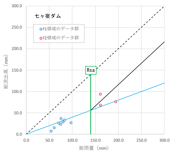
図 1-19 (2) 総降水量と総流出高の関係
