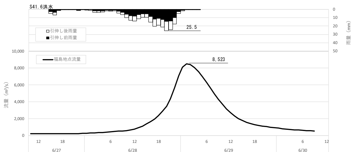
図 1-46 (3) 対象降雨の降雨 36hr 拡大による流出計算結果 (S41.6 洪水、福島地点)
