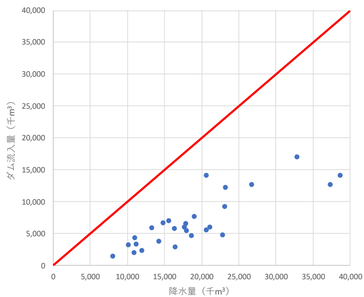
図 1-12 (2) ダム地点における流入量と降雨量の関係（摺上川ダム）
