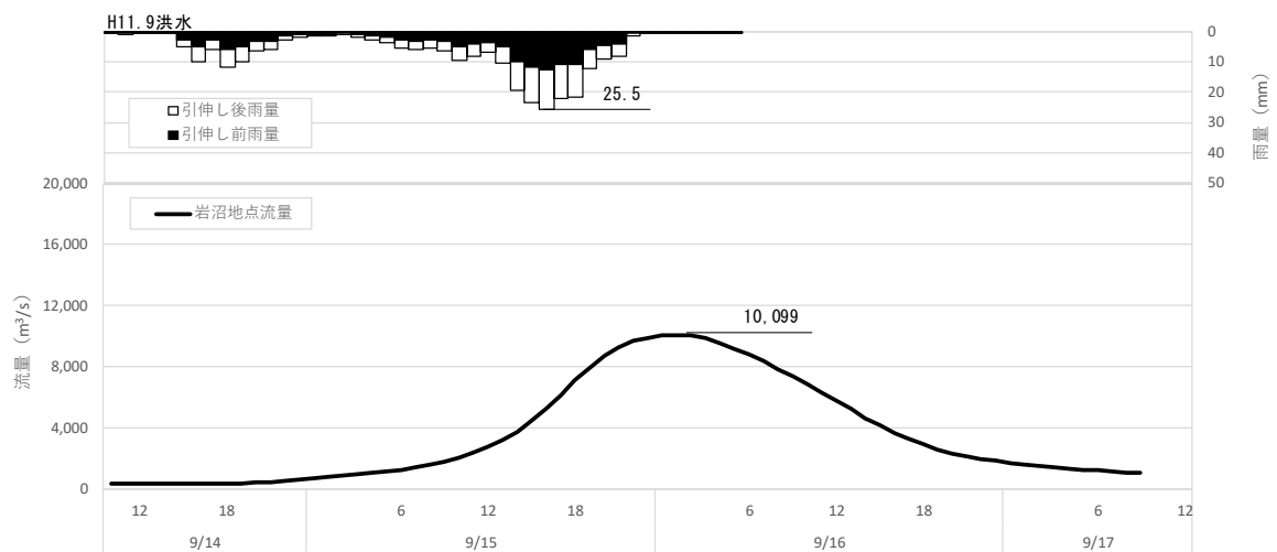
図 1-46 (15) 対象降雨の降雨 36hr 拡大による流出計算結果 (H11.9 洪水、岩沼地点)
