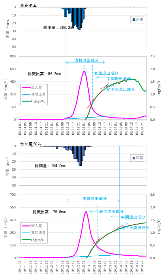
図 1-17 (2) 成分分離の事例 (R1.10 洪水)
