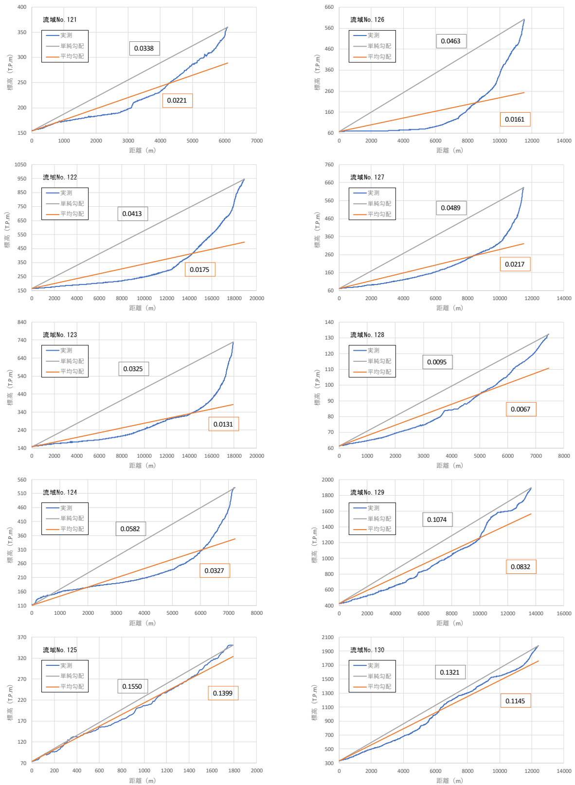
图 1-28 (13) 流域流路勾配
