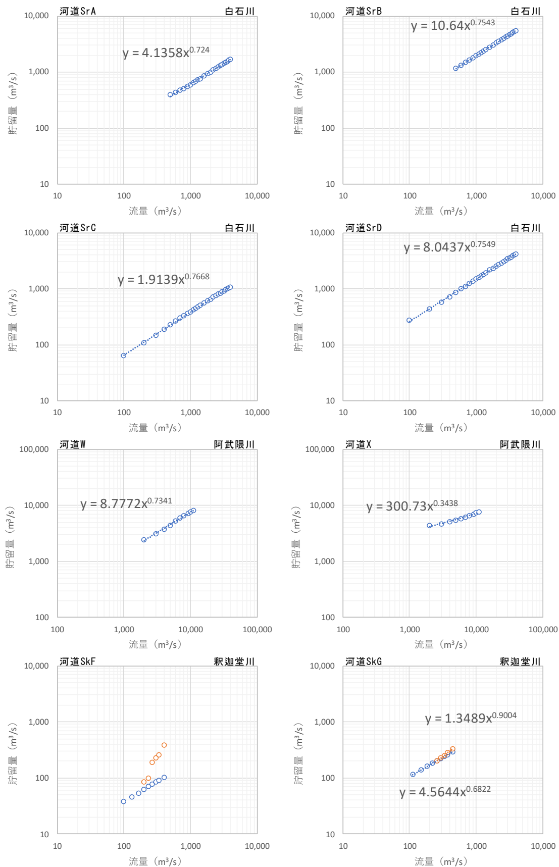
図 1-29 (5) S-Q 関係図
