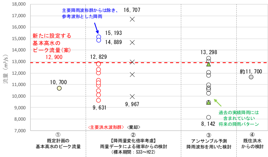
図 1-56 (1) 基本高水の設定にかかる総合判断図（福島地点）
