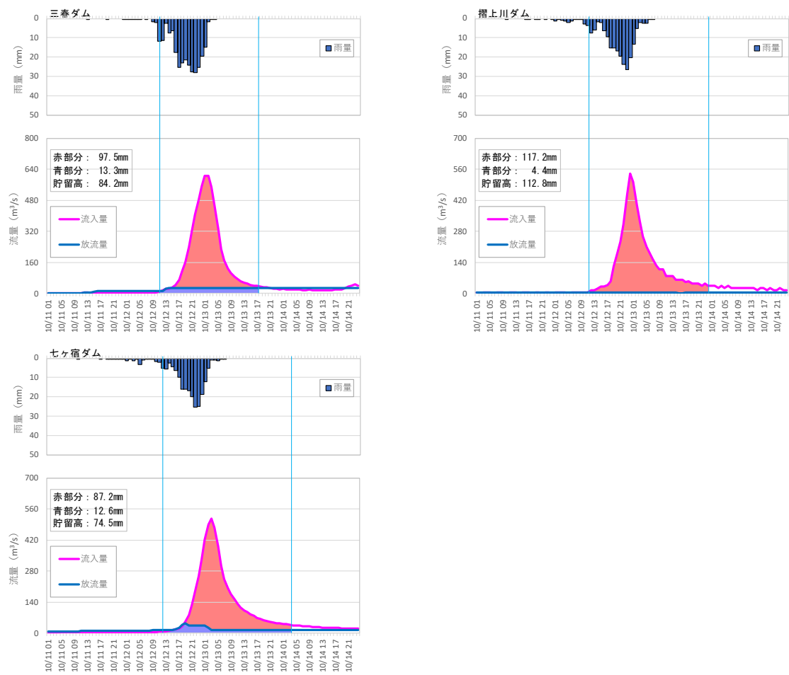
図 1-18 ダム貯留高算定事例 (R1.10 洪水)
