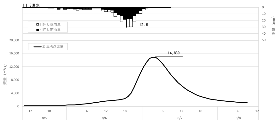
図 1-46 (12) 対象降雨の降雨 36hr 拡大による流出計算結果 (H1.8 洪水、岩沼地点)
