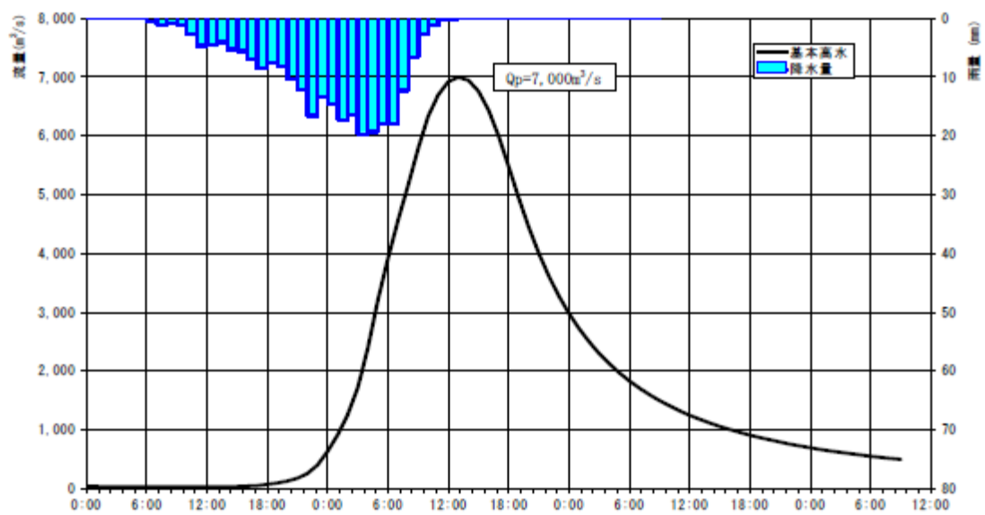
図 1-1 (1) 基本高水ハイドログラフ（福島地点：昭和 61 年 8 月型）
