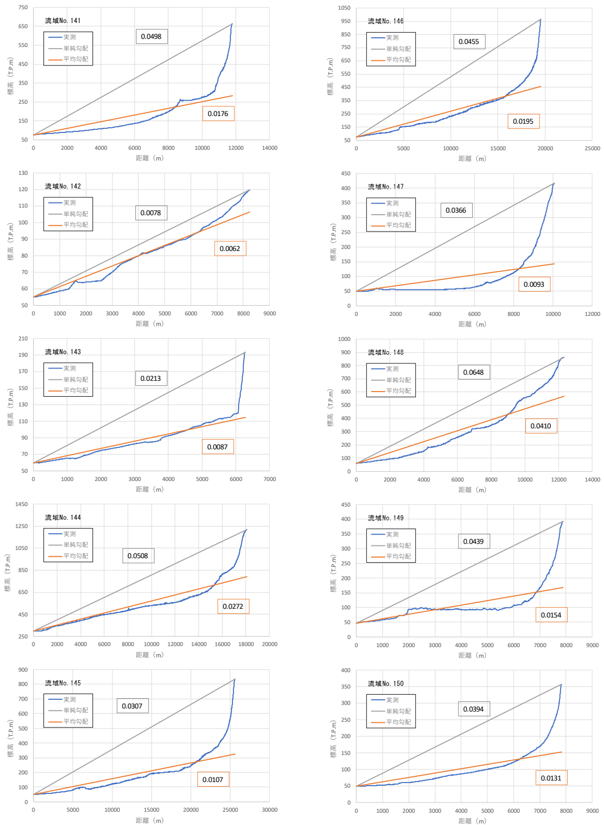
图 1-28 (15) 流域流路勾配
