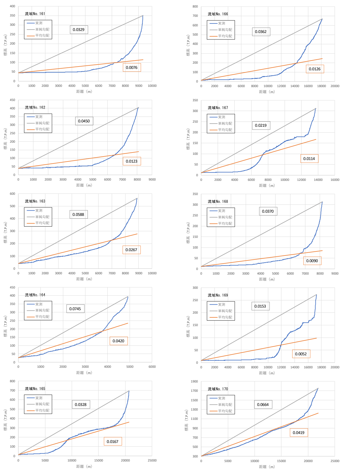
图 1-28 (17) 流域流路勾配
