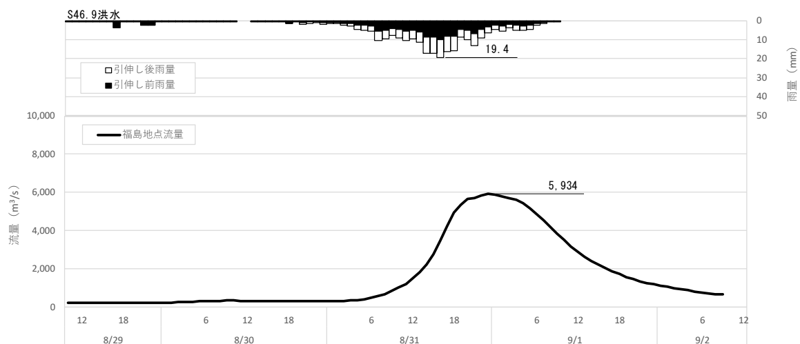
図 1-46 (4) 対象降雨の降雨 36hr 拡大による流出計算結果 (S46.9 洪水、福島地点)
