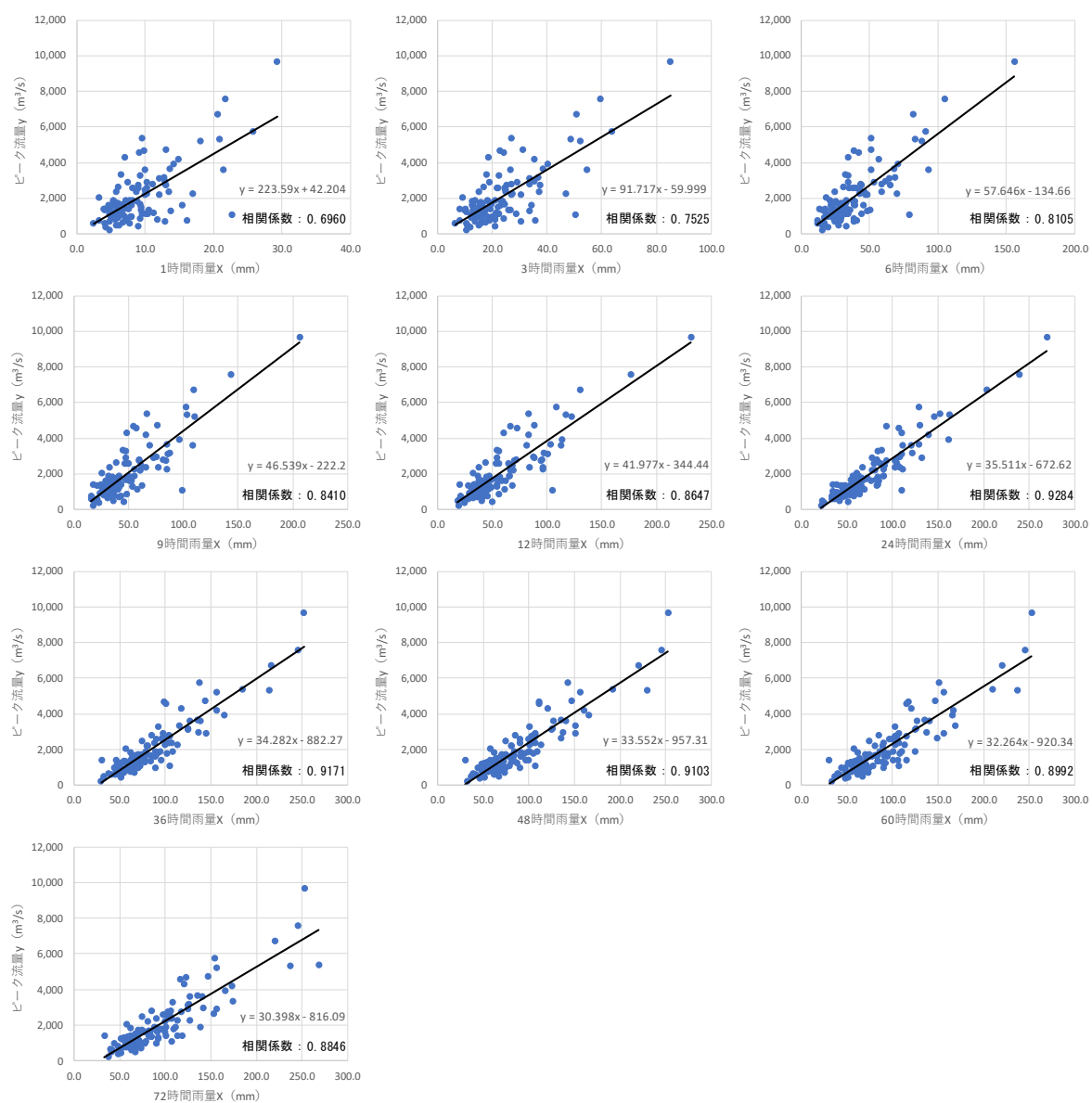
図 1-40 (4) ピーク流量と雨量との相関関係
