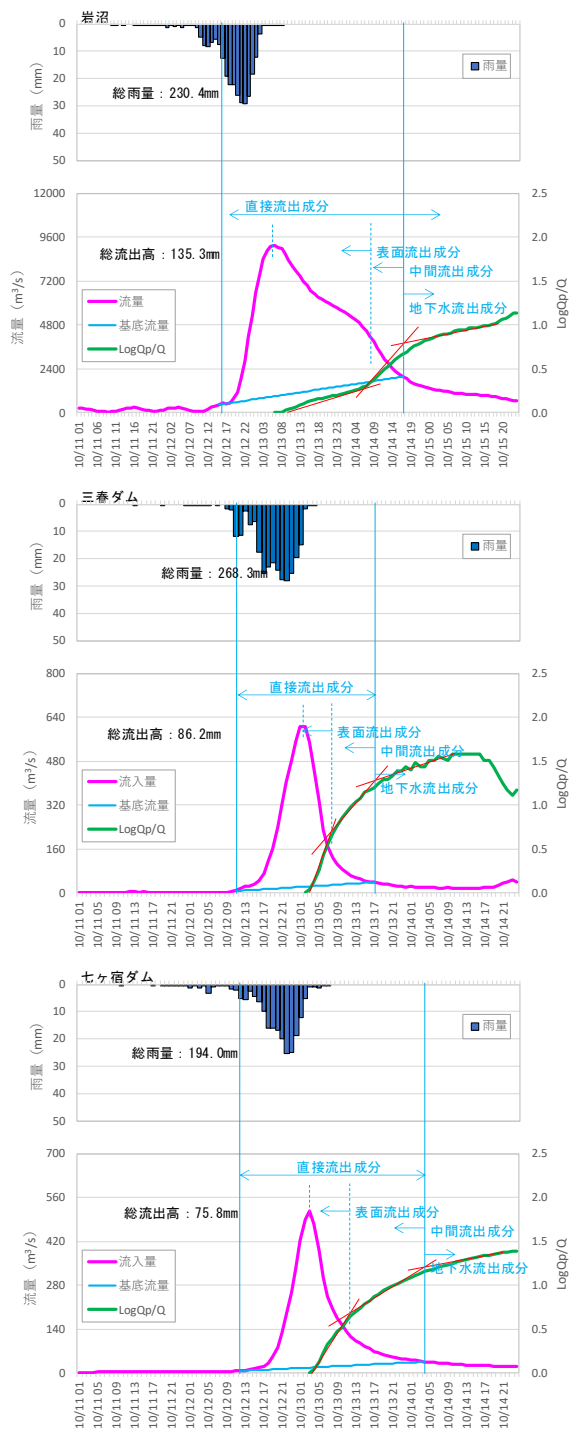
図 1-17 (2) 成分分離の事例 (R1.10 洪水)
