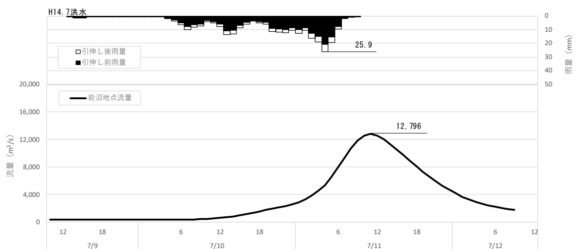
図 1-46 (17) 対象降雨の降雨 36hr 拡大による流出計算結果 (H14.7 洪水、岩沼地点)
