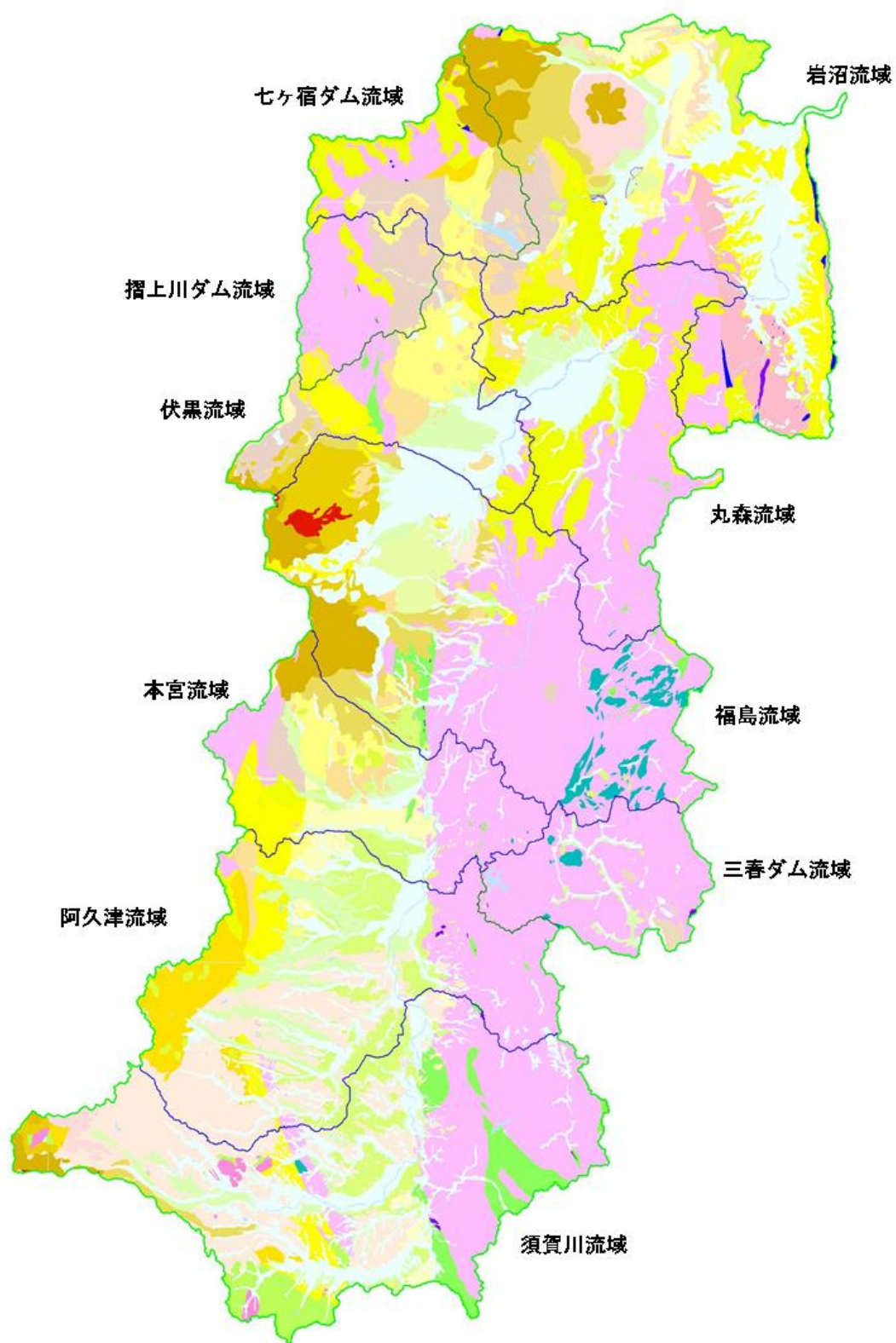
図 1-23 阿武隈川流域地質図（シームレス地質図）
