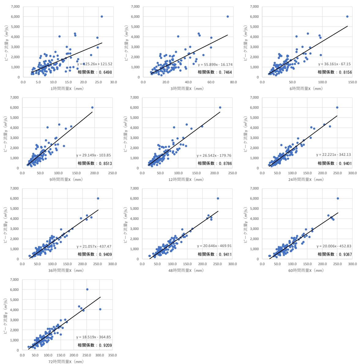
図 1-40 (2) ピーク流量と雨量との相関関係
