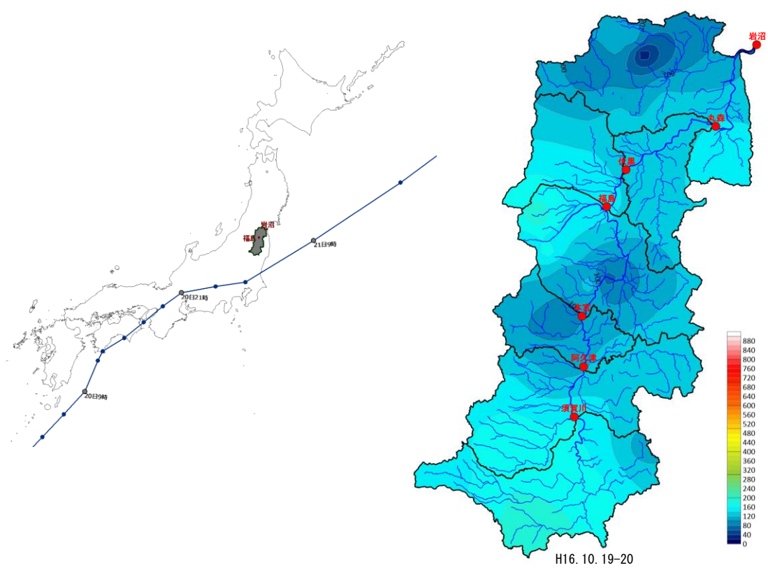
図 1-4 (9) 台風経路図及び等雨量線図 (H16.10.19-20 洪水)
