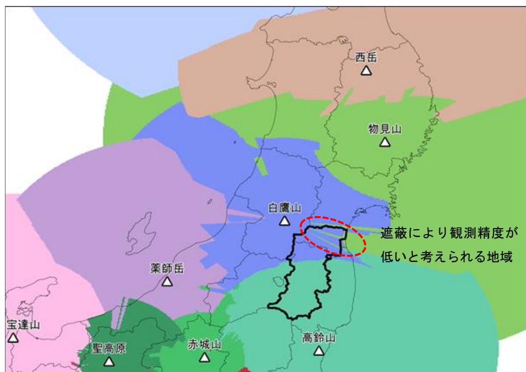
図 1-7 C バンドレーダ合成マップ
