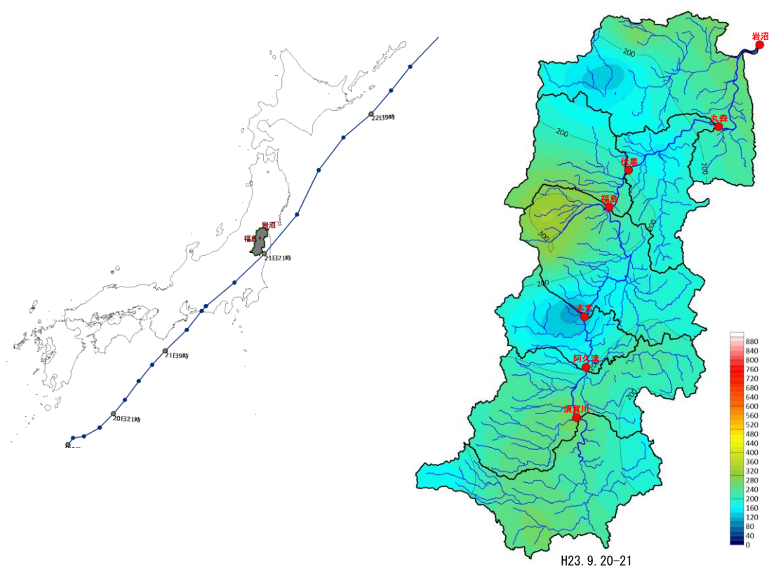
図 1-4 (11) 台風経路図及び等雨量線図 (H23.9.20-21 洪水)
