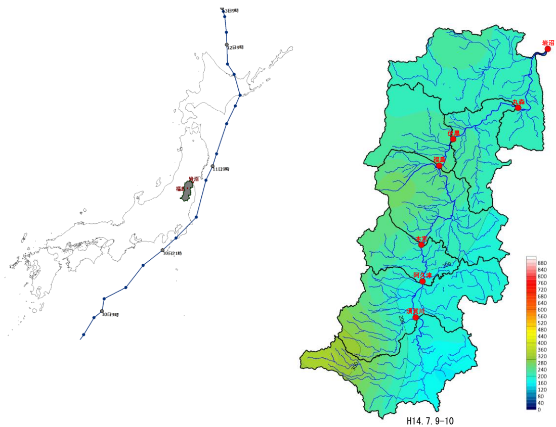
図 1-4 (8) 台風経路図及び等雨量線図 (H14.7.9-10 洪水)
