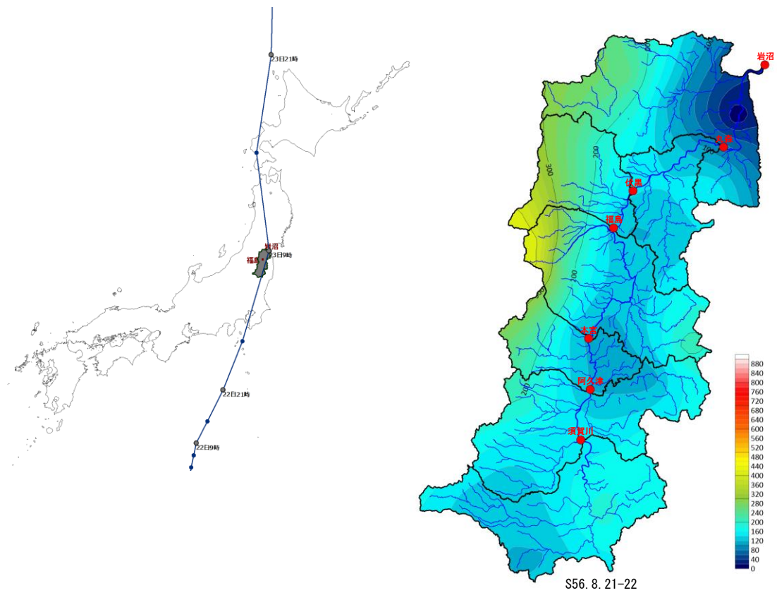
図 1-4 (2) 台風経路図及び等雨量線図 (S56.8.21-22 洪水)
