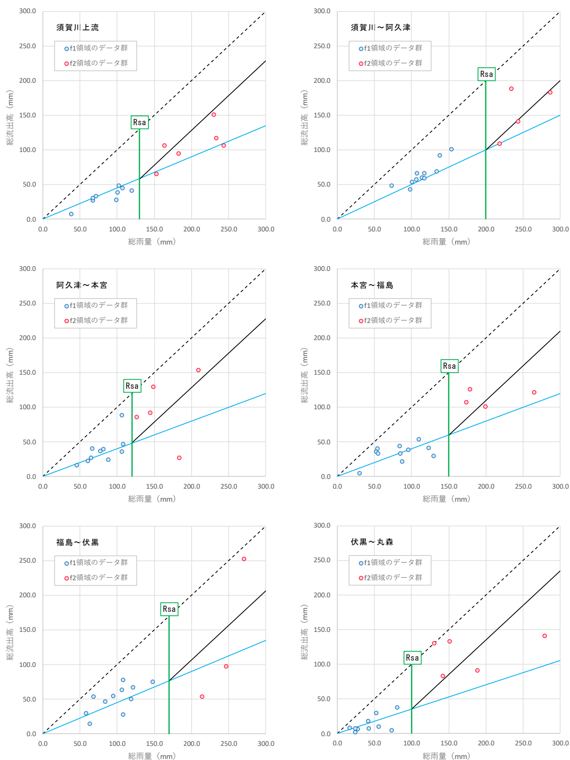
図 1-19 (1) 総降雨量と総流出高の関係
