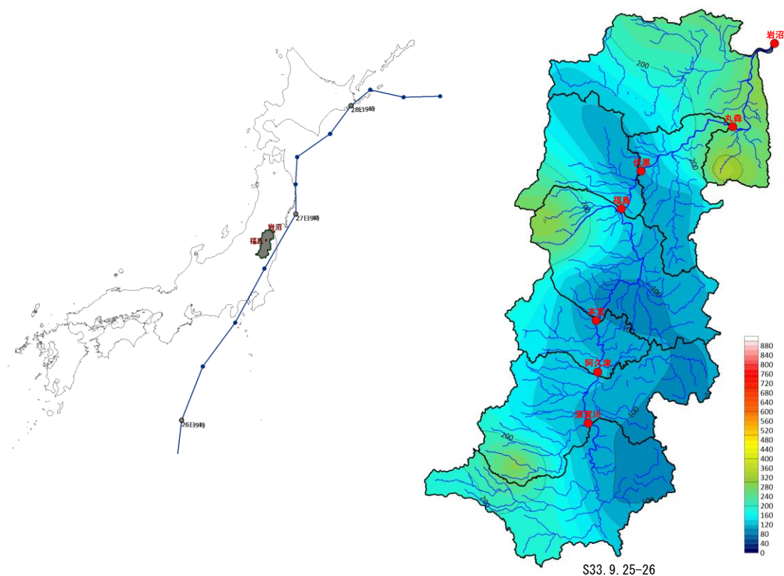
図 1-4 (1) 台風経路図及び等雨量線図 (S33.9.25-26 洪水)
