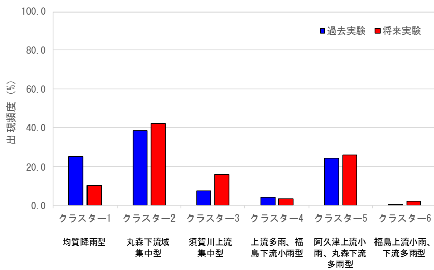
図 1-52 (2) 出現頻度 (岩沼地点)
