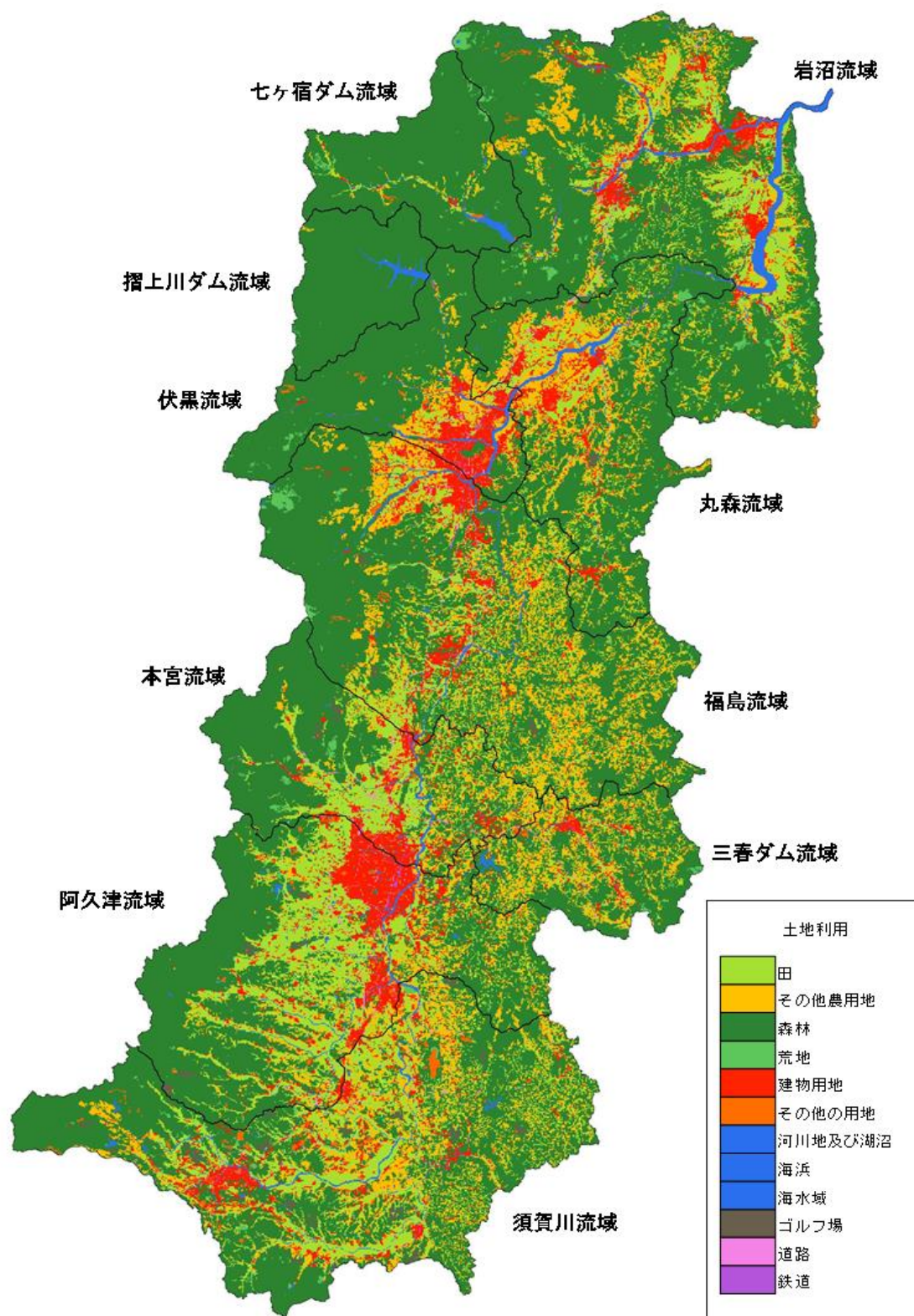
図 1-26 土地利用図（細分区画土地利用データ H26）
