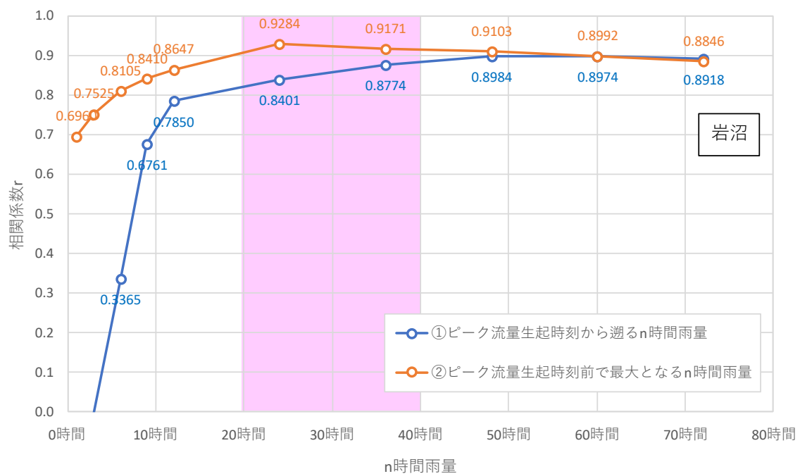
図 1-39 ピーク流量と短時間雨量との相関関係
