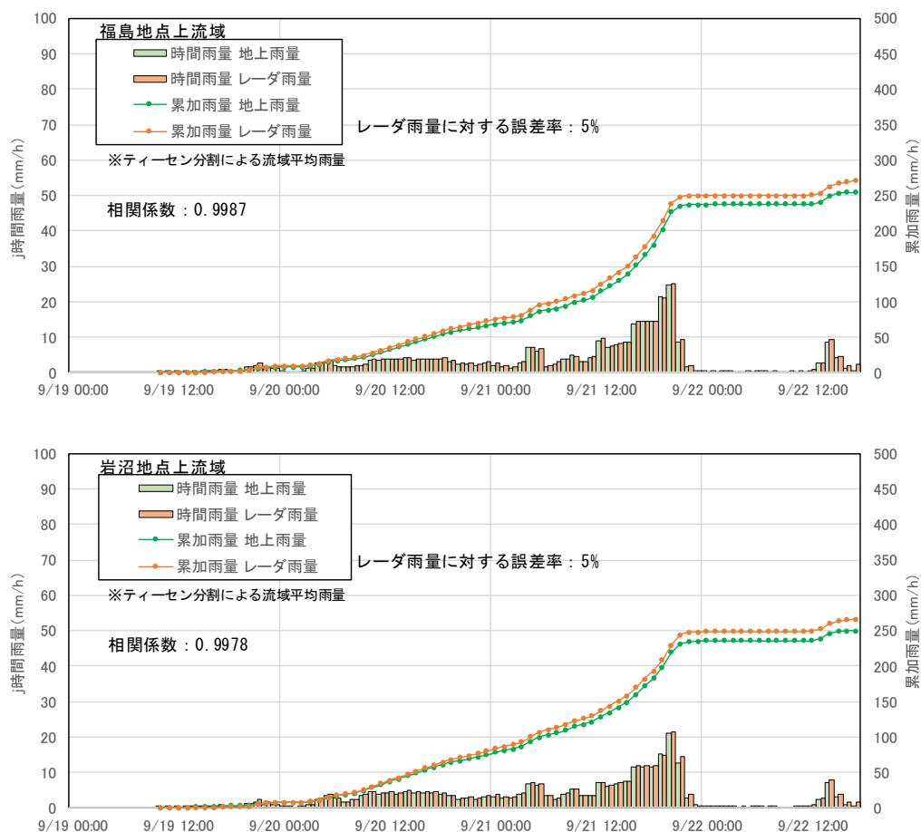
図 1-5 (1) 地上観測所雨量とレーダ雨量の比較（平成 23 年（2011 年）9 月洪水）
