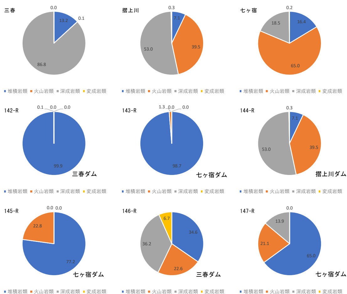
図 1-22 各流域の地質分布
