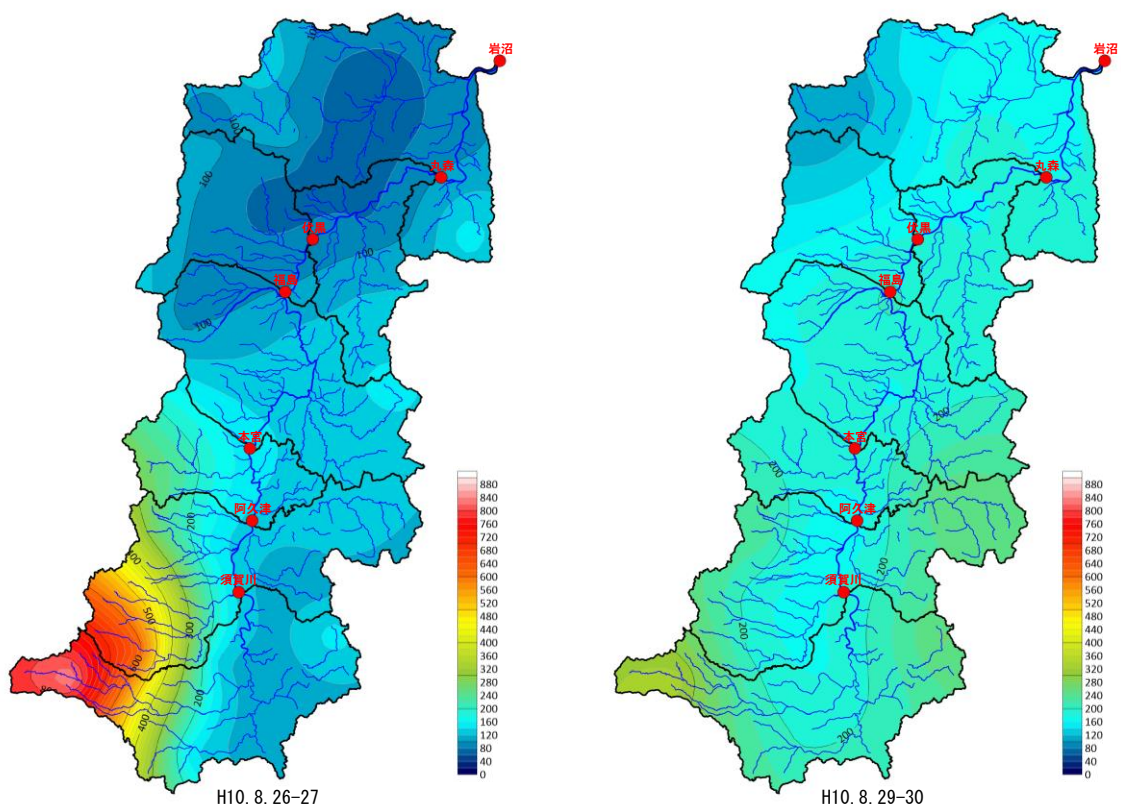
図 1-4 (6) 台風経路図及び等雨量線図 (H10.8 洪水 (前線))
