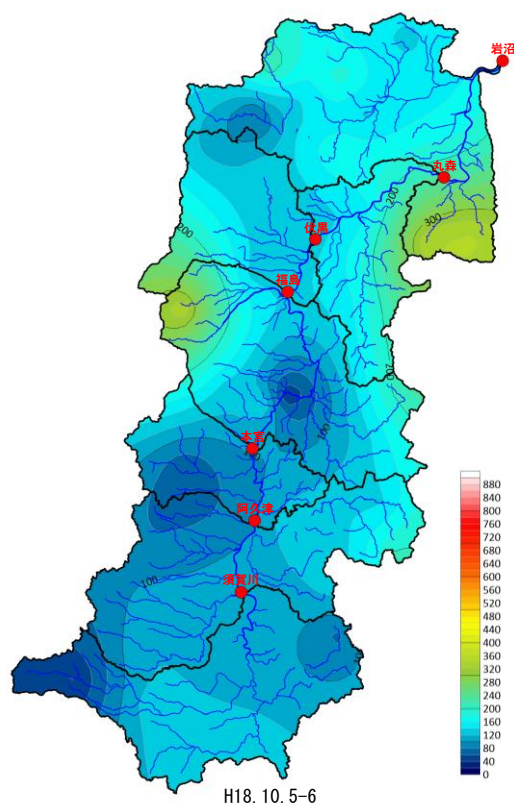
図 1-4 (10) 台風経路図及び等雨量線図 (H18.10.5-6 洪水 (低気圧・前線))
