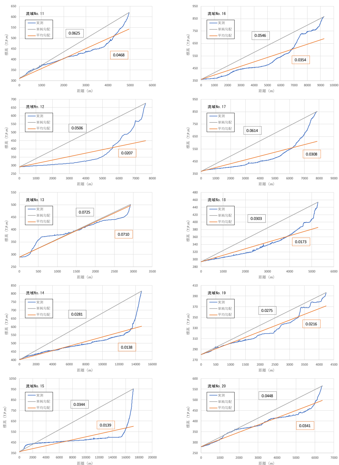
图 1-28 (2) 流域流路勾配
