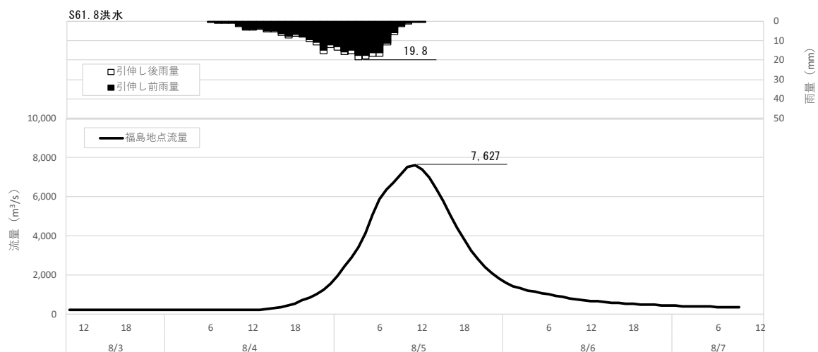
図 1-46 (10) 対象降雨の降雨 36hr 拡大による流出計算結果 (S61.8 洪水、福島地点)
