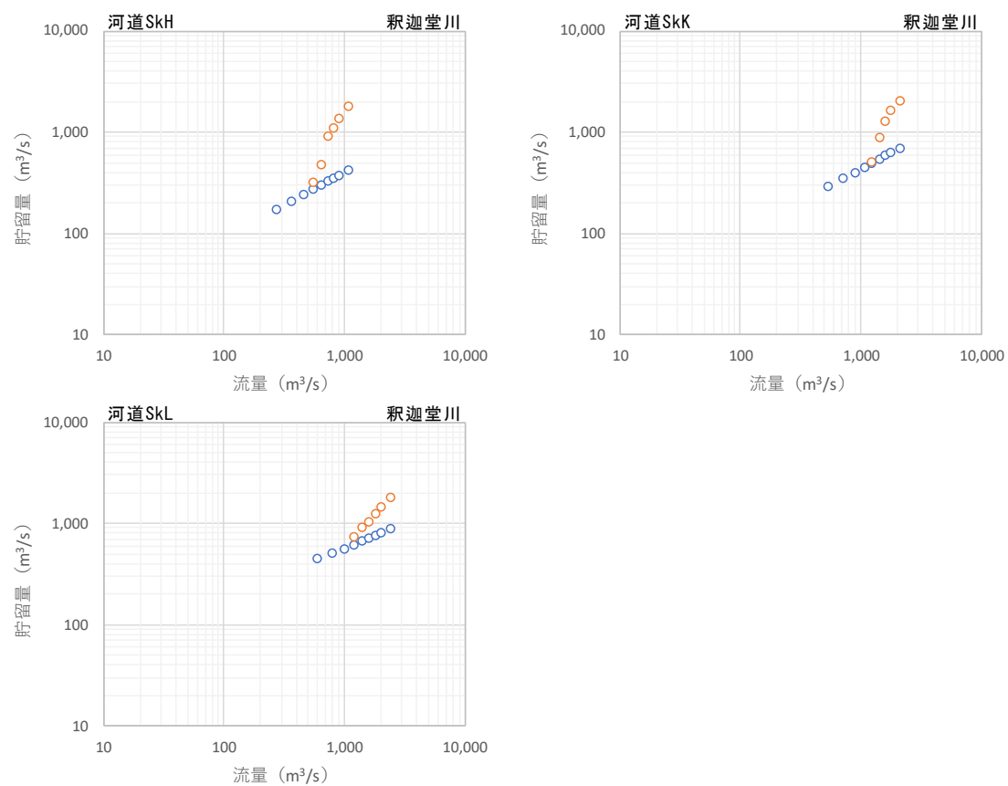
図 1-29 (6) S-Q 関係図
