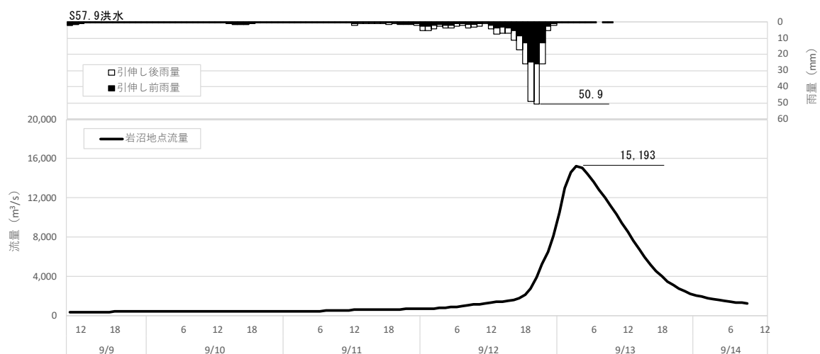
図 1-46 (9) 対象降雨の降雨 36hr 拡大による流出計算結果 (S57.9 洪水、岩沼地点)
