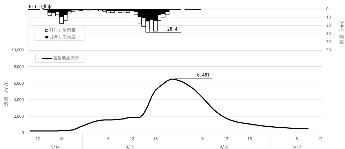
図 1-46 (14) 対象降雨の降雨 36hr 拡大による流出計算結果 (H11.9 洪水、福島地点)
