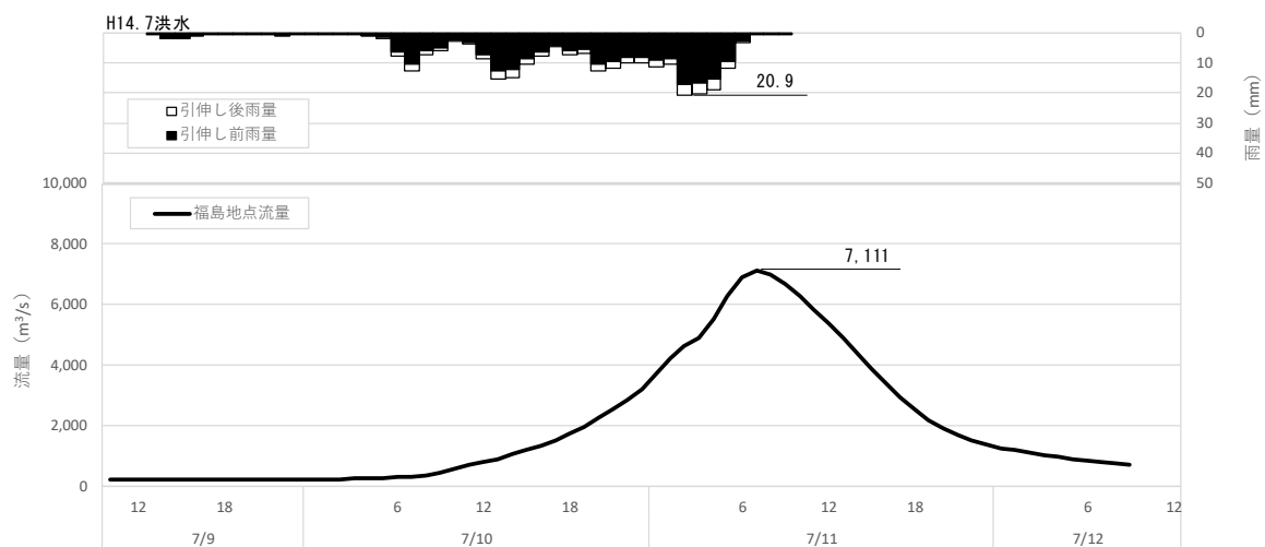
図 1-46 (16) 対象降雨の降雨 36hr 拡大による流出計算結果 (H14.7 洪水、福島地点)
