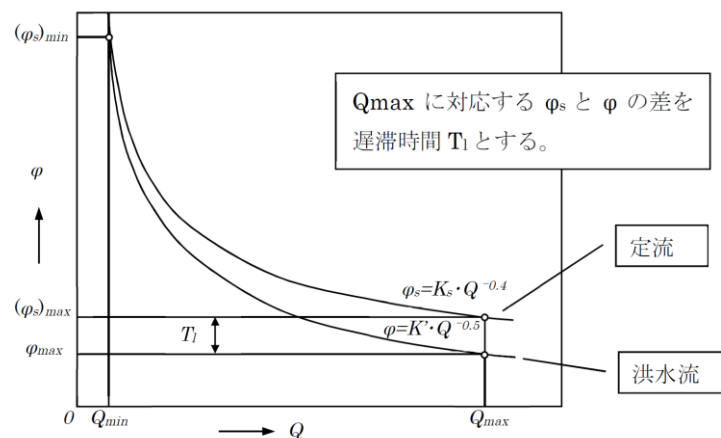
図 1-30 定流の貯留関数 \varphi_s と洪水流の貯留関数 \varphi の関係
