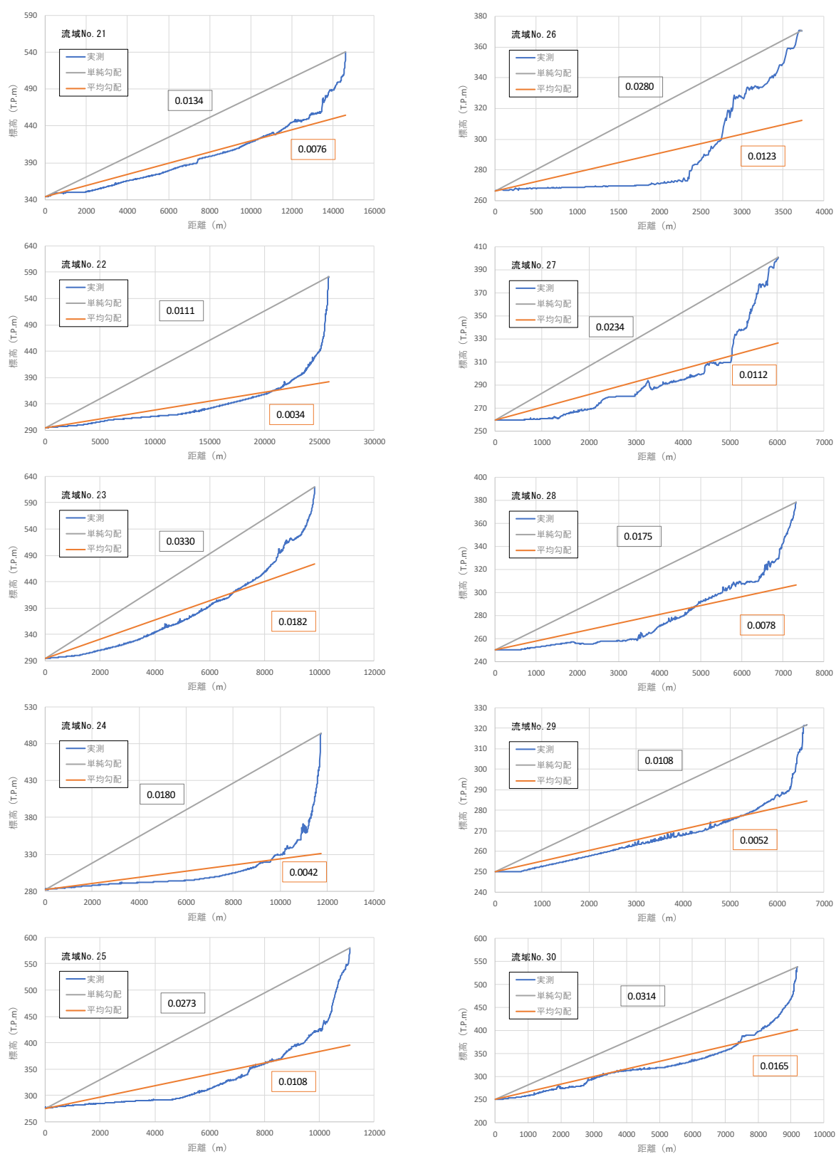
图 1-28 (3) 流域流路勾配
