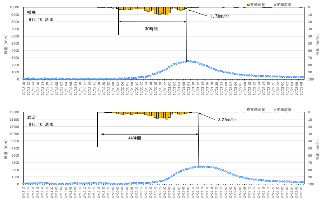
図 1-36 (3) Kinematic Wave 法による洪水到達時間
