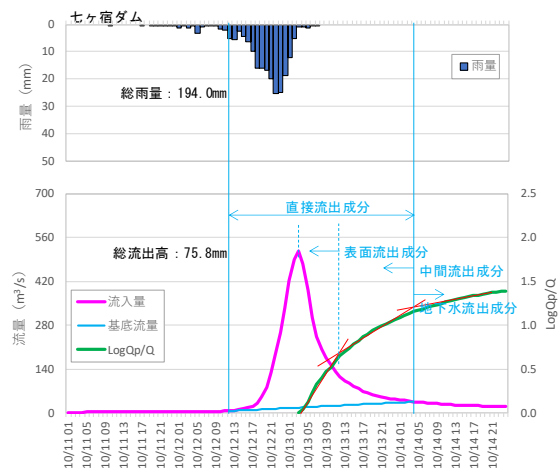
図 1-17 (2) 成分分離の事例 (R1.10 洪水)
