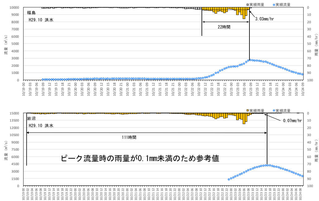
図 1-36 (1) Kinematic Wave 法による洪水到達時間
