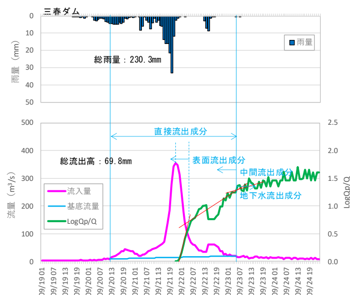
図 1-10 成分分析の概念図
