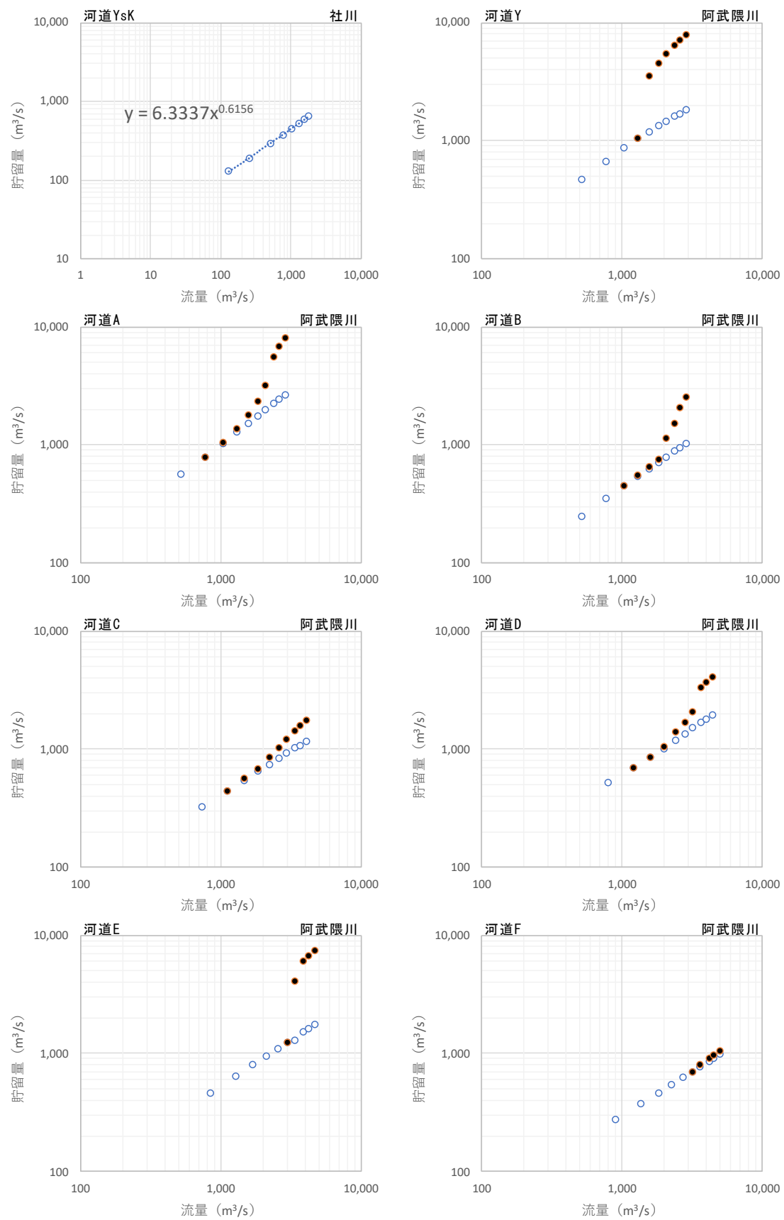
図 1-29 (2) S-Q 関係図
