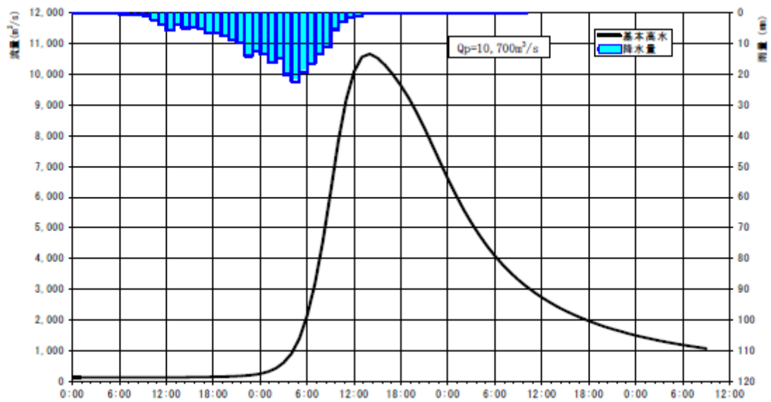
図 1-1 (2) 基本高水ハイドログラフ（岩沼地点：昭和 61 年 8 月型）
