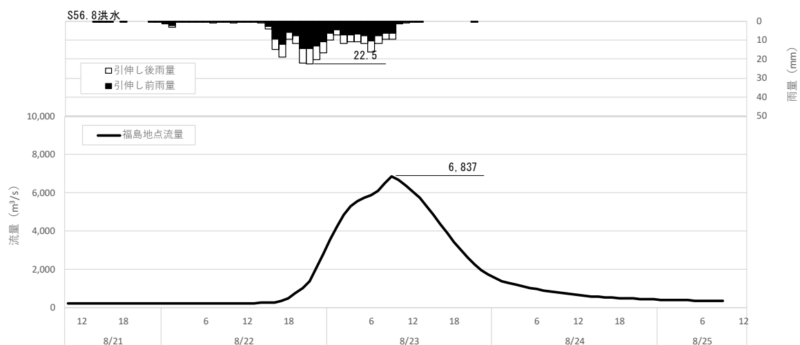
図 1-46 (6) 対象降雨の降雨 36hr 拡大による流出計算結果 (S56.8 洪水、福島地点)
