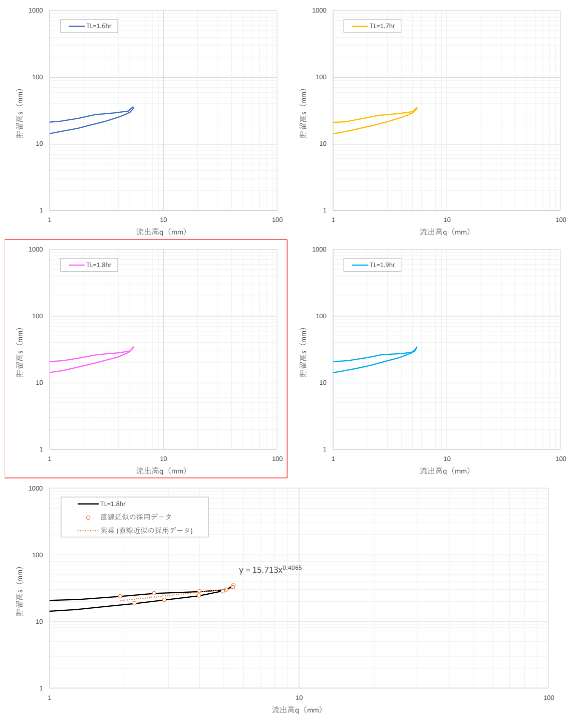
図 1-21 (1) 貯留高－流出高関係図（三春ダム地点：H23.9 洪水）
