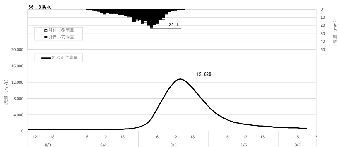
図 1-46 (11) 対象降雨の降雨 36hr 拡大による流出計算結果 (S61.8 洪水、岩沼地点)
