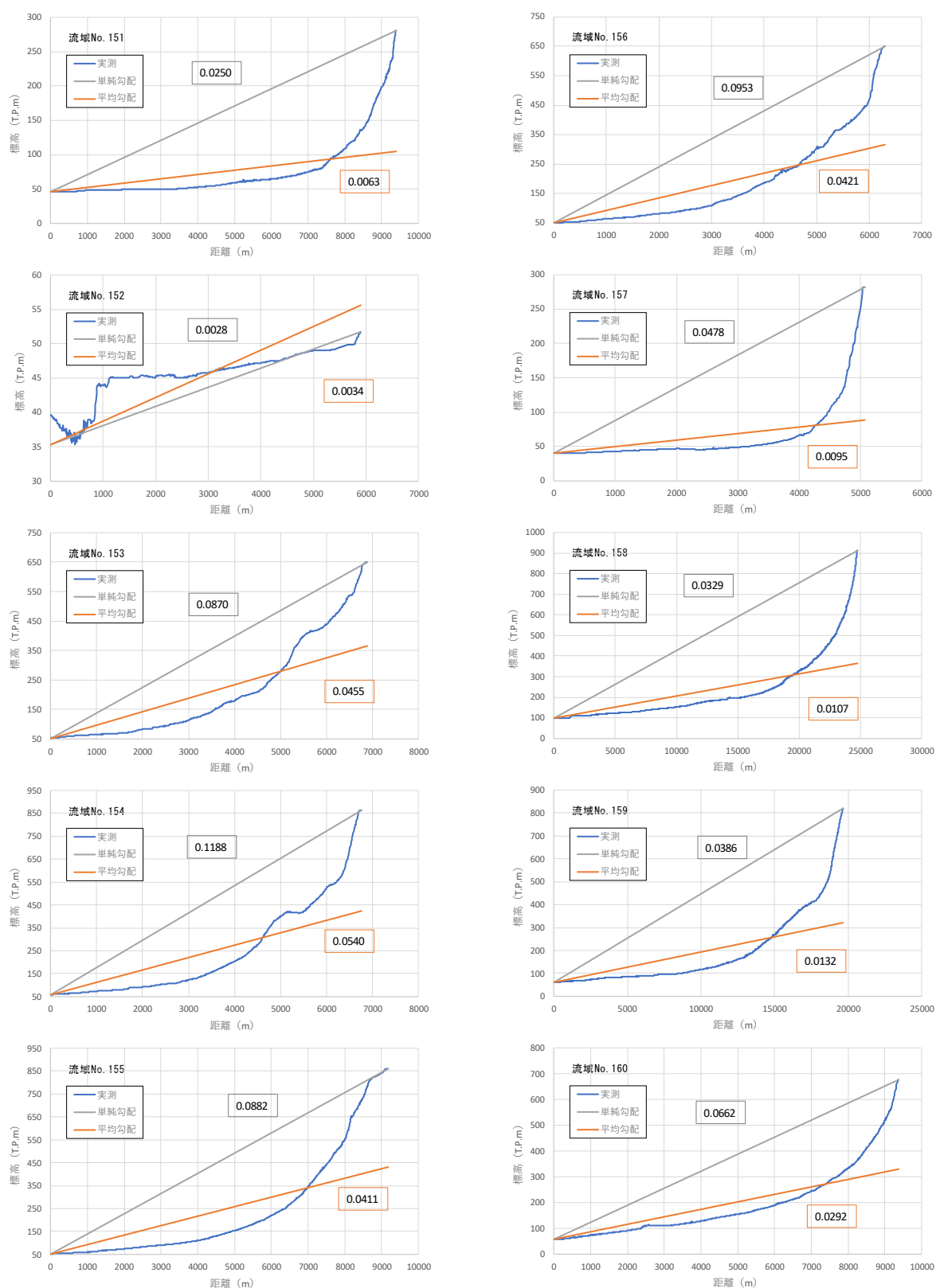
图 1-28 (16) 流域流路勾配
