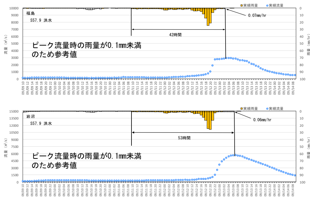
図 1-36 (6) Kinematic Wave 法による洪水到達時間
