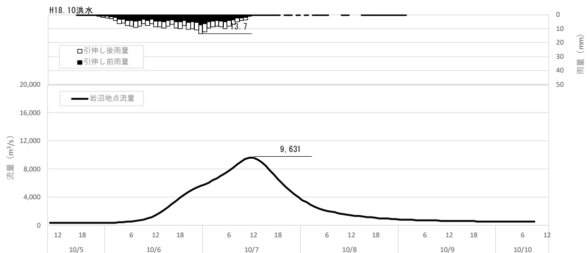
図 1-46 (19) 対象降雨の降雨 36hr 拡大による流出計算結果 (H18.10 洪水、岩沼地点)
