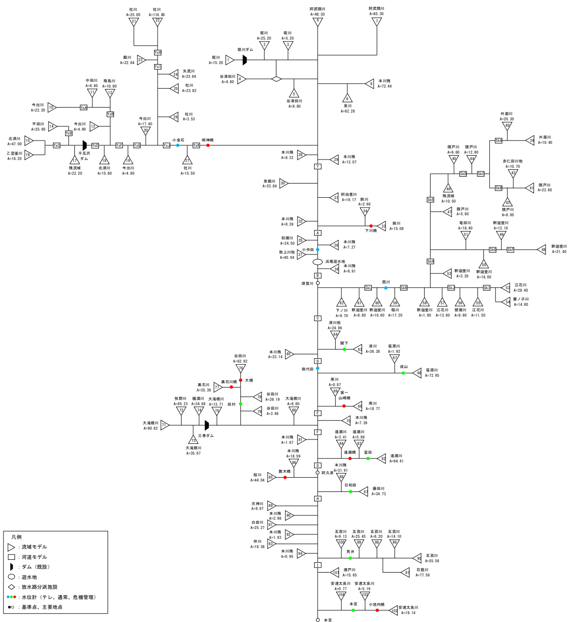
図 1-14 (1) 流出モデル模式図
