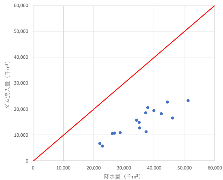
図 1-12 (3) ダム地点における流入量と降雨量の関係（セヶ宿ダム）
