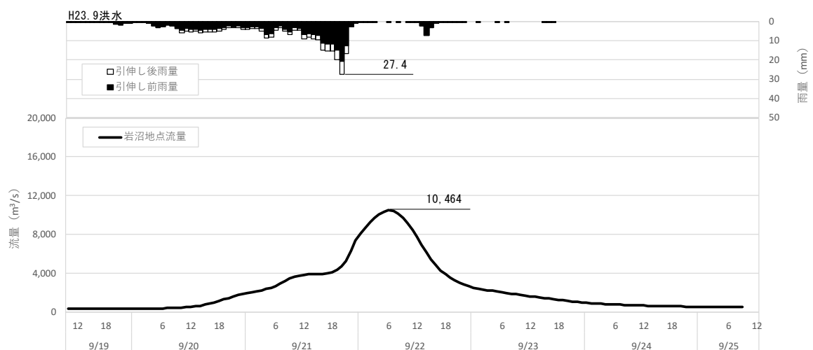
図 1-46 (21) 対象降雨の降雨 36hr 拡大による流出計算結果 (H23.9 洪水、岩沼地点)
