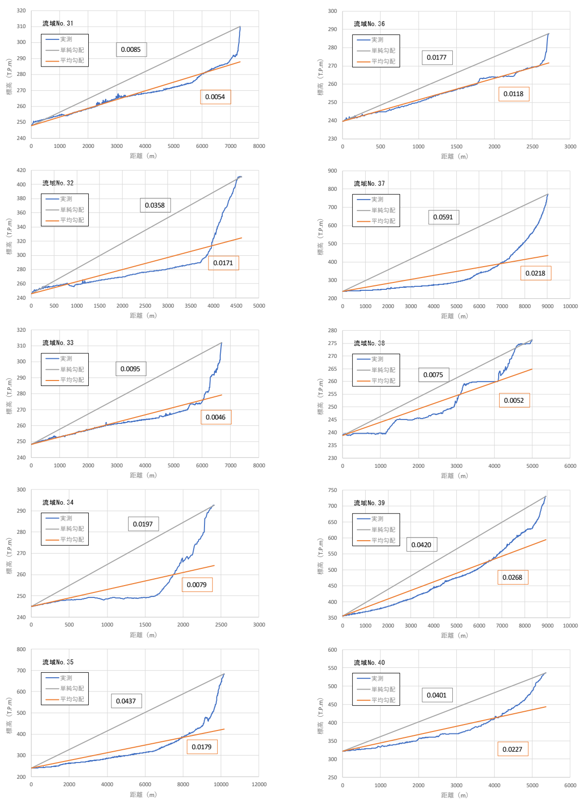
图 1-28 (4) 流域流路勾配
