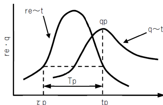
図 1-35 Kinematic Wave 法による T_p の定義
