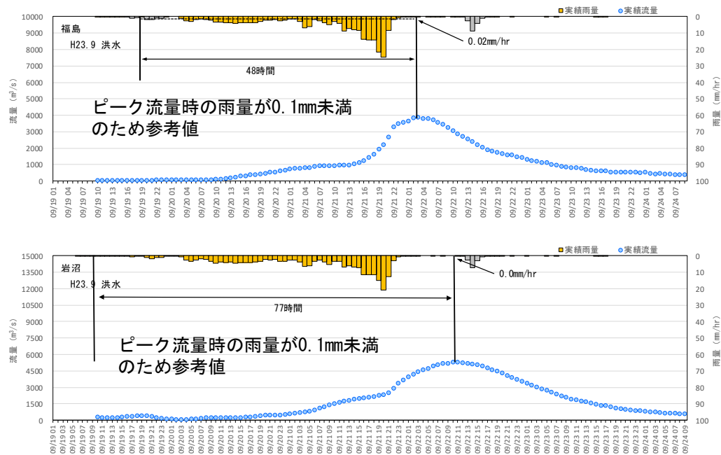
図 1-36 (2) Kinematic Wave 法による洪水到達時間
