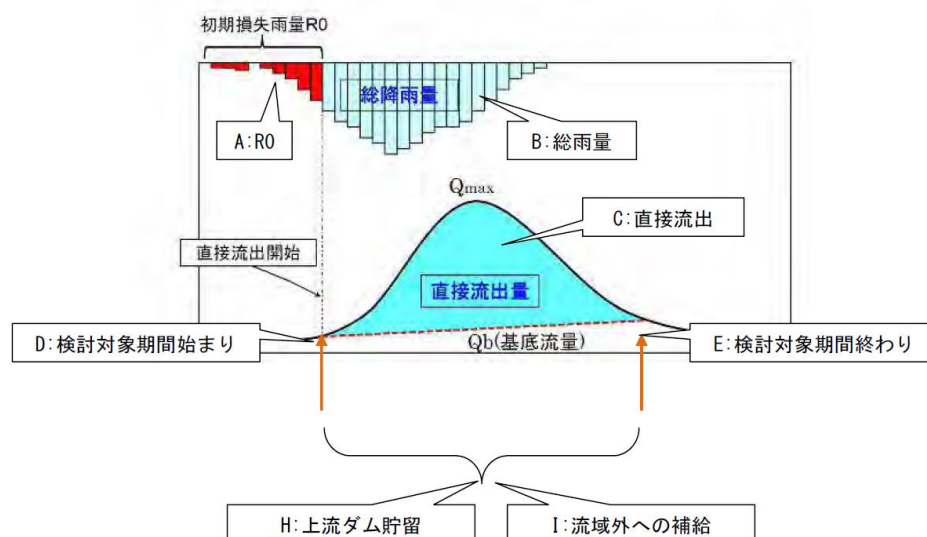
図 1-16 成分分離の概念図
