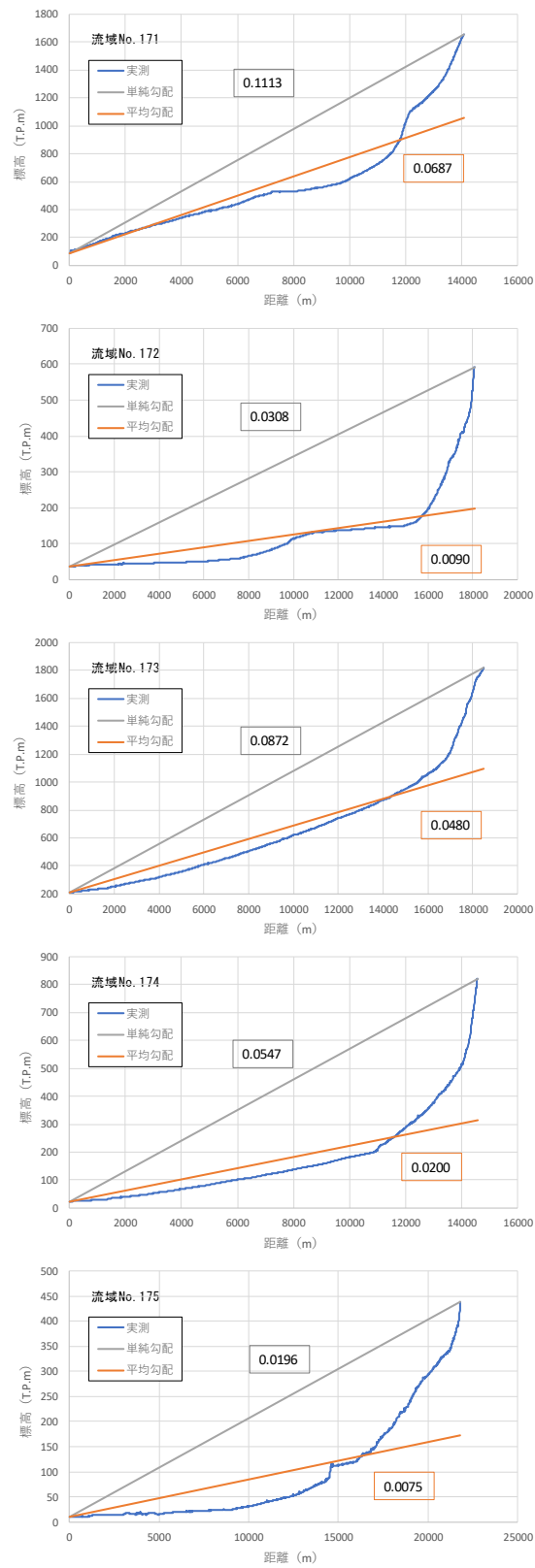
图 1-28 (18) 流域流路勾配
