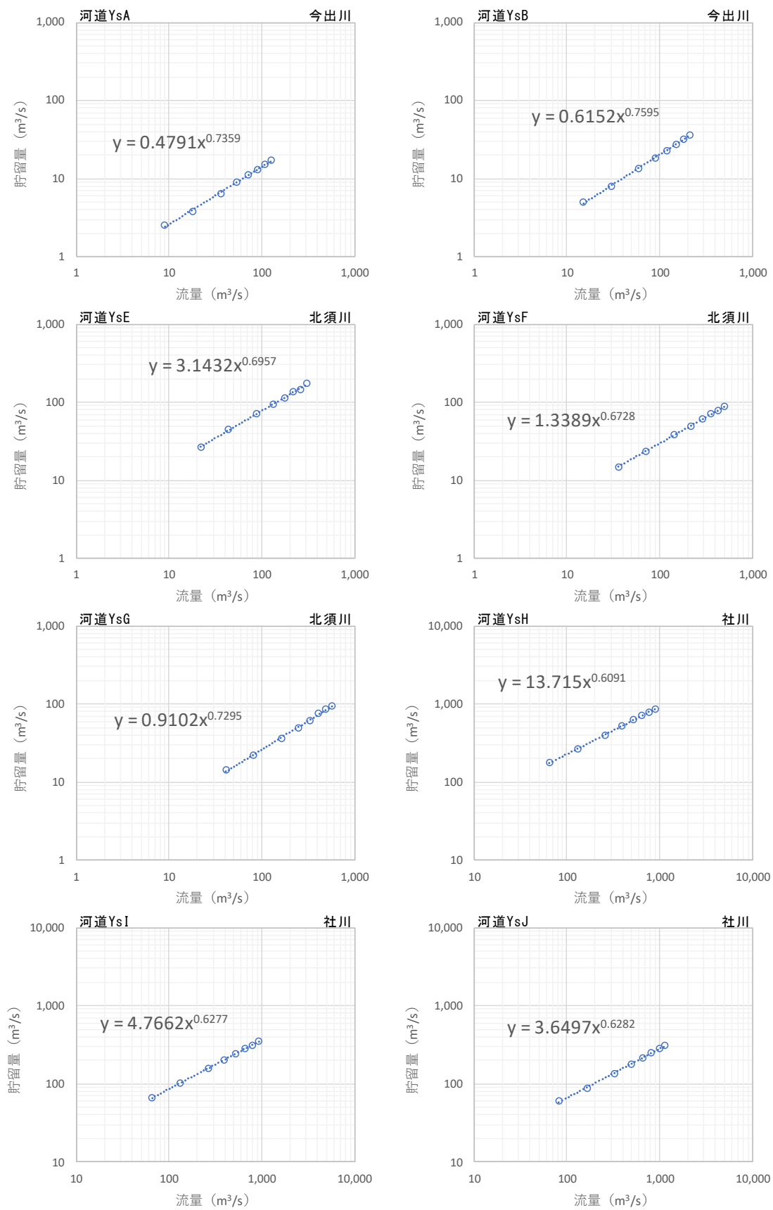
図 1-29 (1) S-Q 関係図
