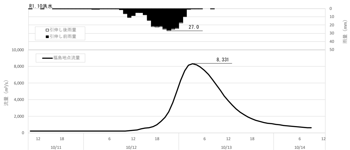
図 1-46 (24) 対象降雨の降雨 36hr 拡大による流出計算結果 (R1.10 洪水、福島地点)
