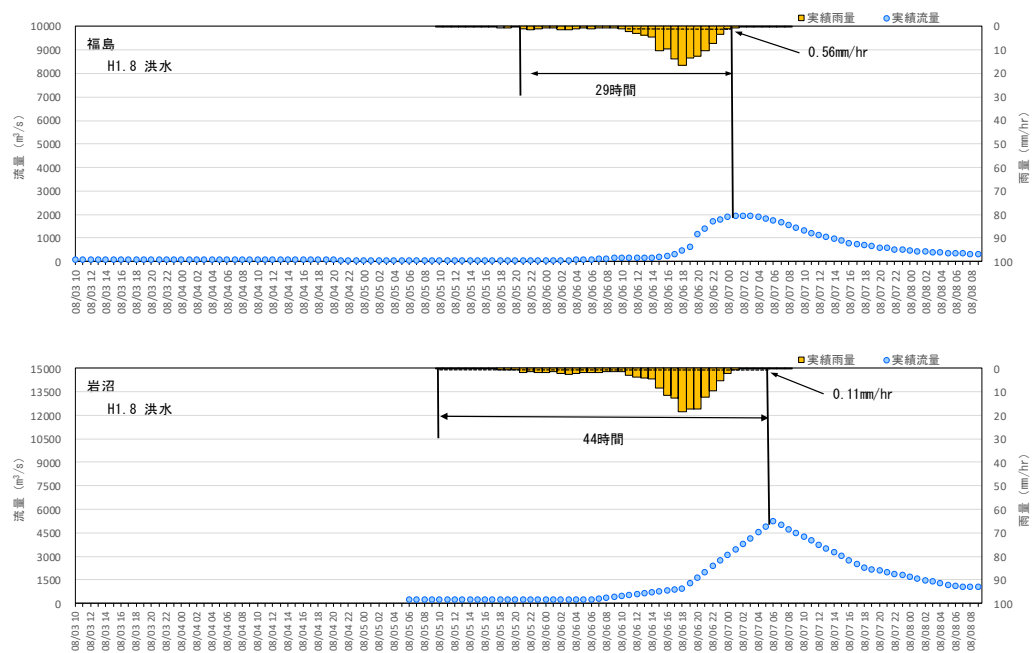
図 1-36 (5) Kinematic Wave 法による洪水到達時間
