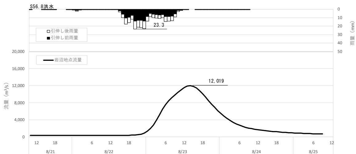
図 1-46 (7) 対象降雨の降雨 36hr 拡大による流出計算結果 (S56.8 洪水、岩沼地点)
