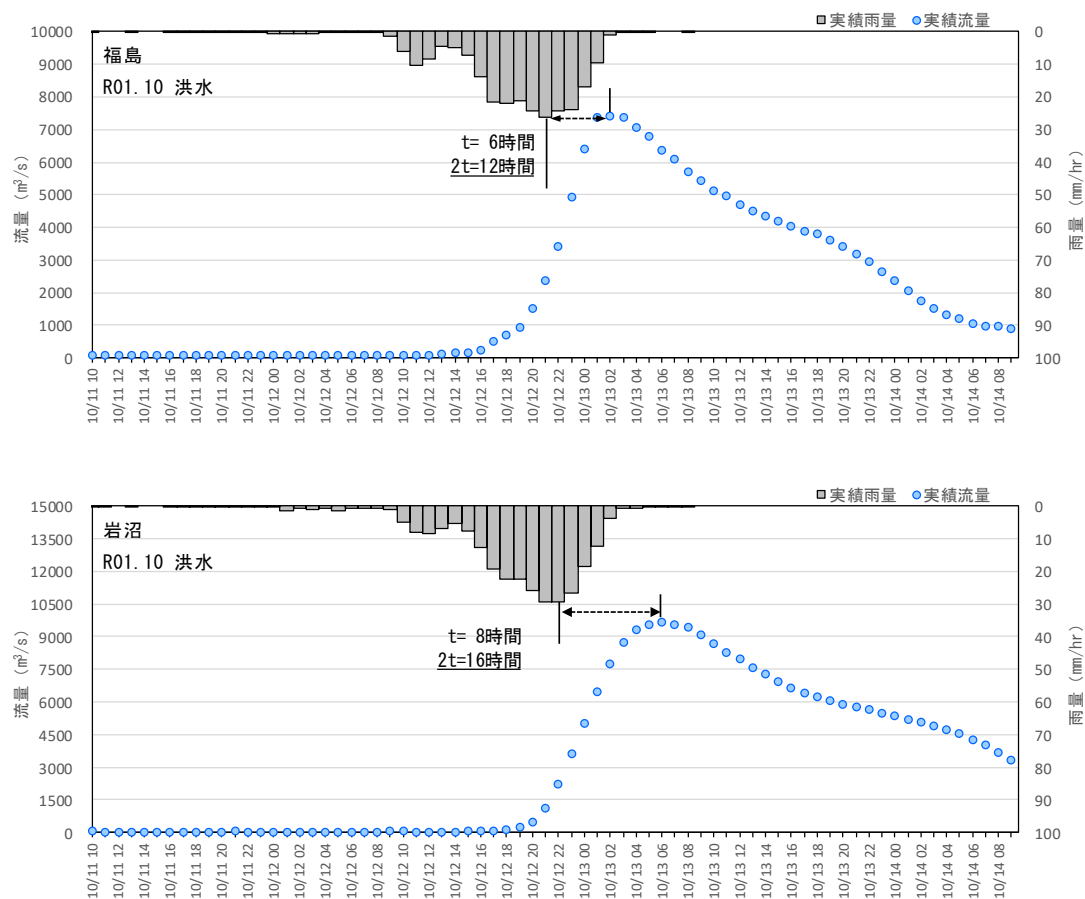
図 1-37 降雨ピークと流量ピークとの時差の2倍による洪水到達時間の算定例
