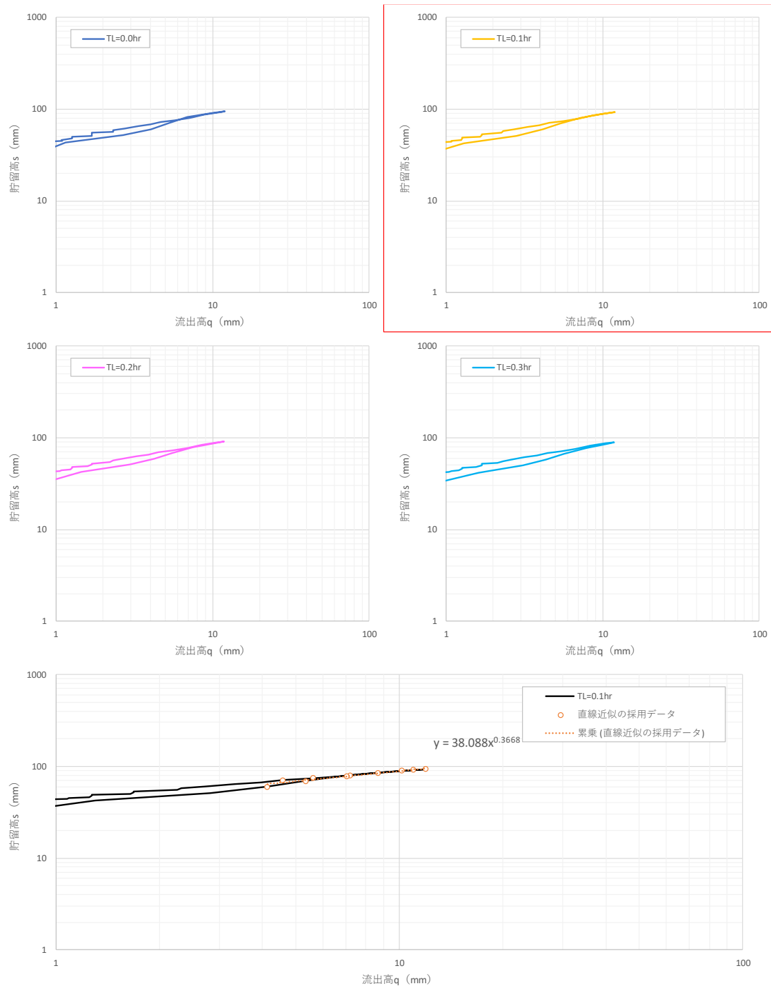
図 1-21 (2) 貯留高－流出高関係図（摺上川ダム地点：R1.10 洪水）
