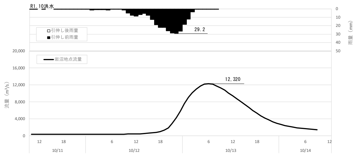
図 1-46 (25) 対象降雨の降雨 36hr 拡大による流出計算結果 (R1.10 洪水、岩沼地点)
