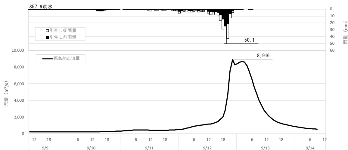
図 1-46 (8) 対象降雨の降雨 36hr 拡大による流出計算結果 (S57.9 洪水、福島地点)
