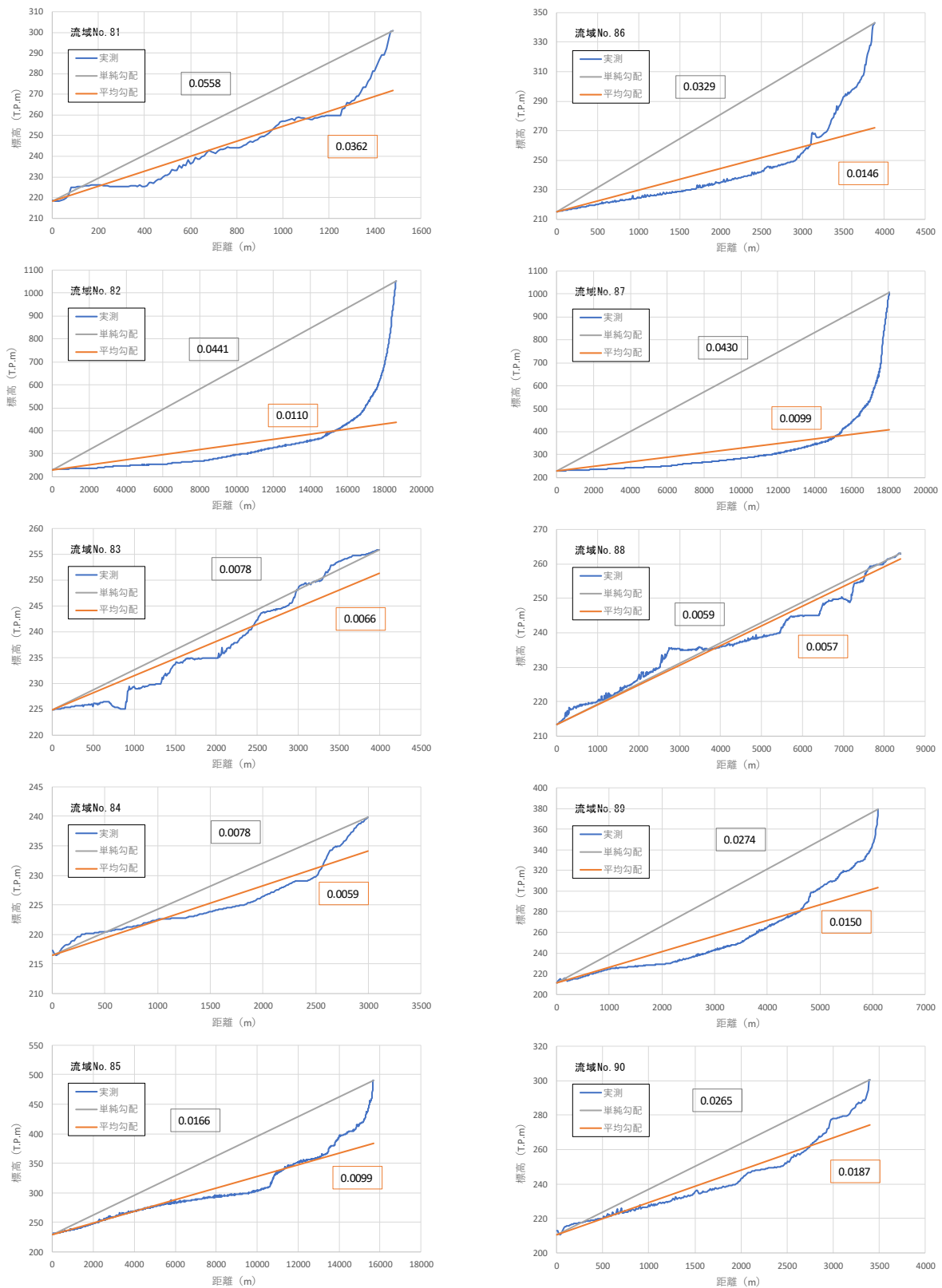
图 1-28 (9) 流域流路勾配
