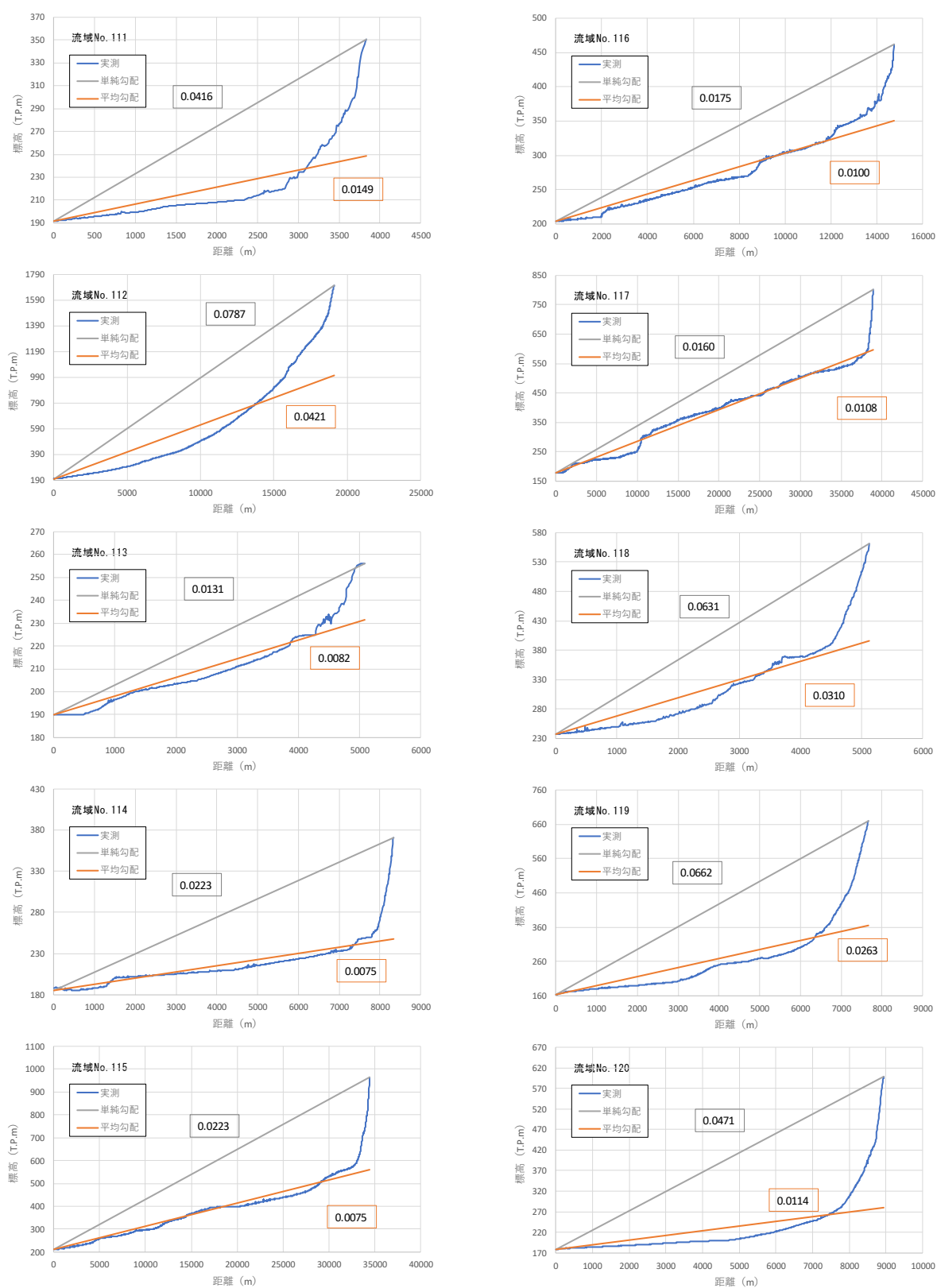
图 1-28 (12) 流域流路勾配
