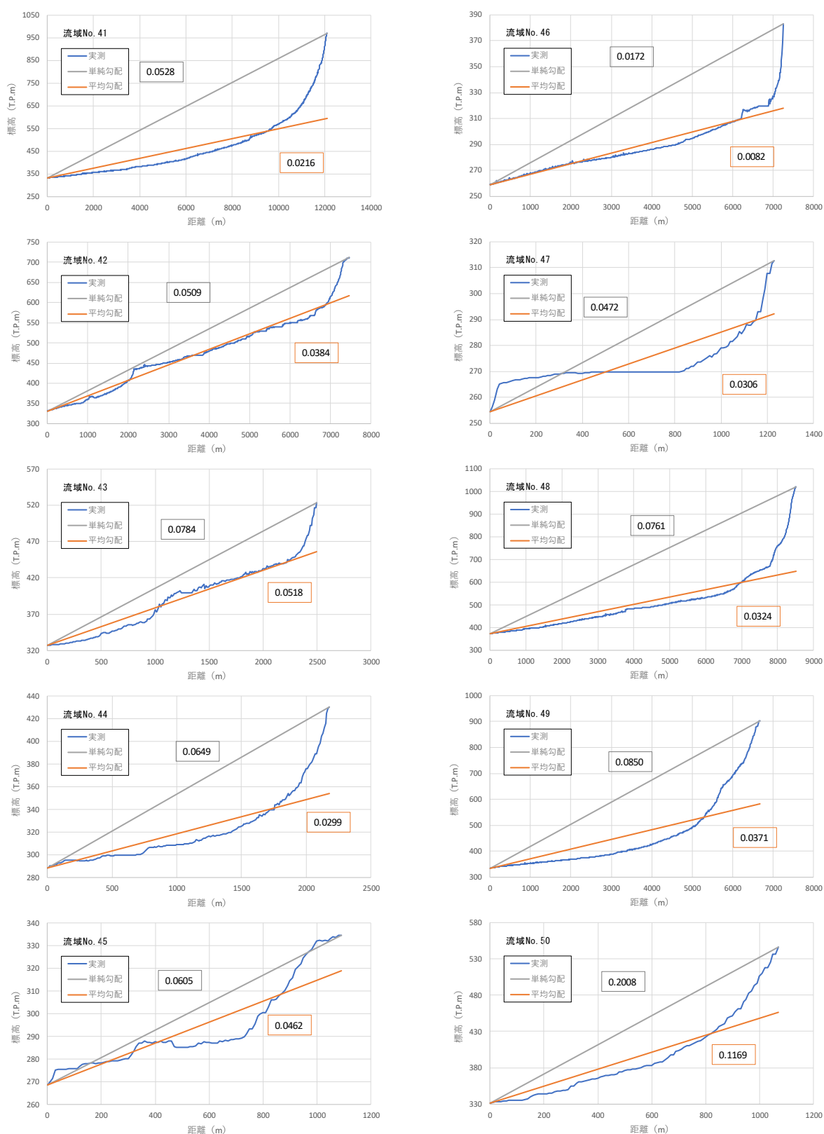
图 1-28 (5) 流域流路勾配
