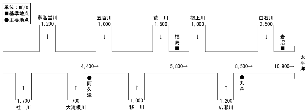
図 3-1 阿武隈川計画流量図
