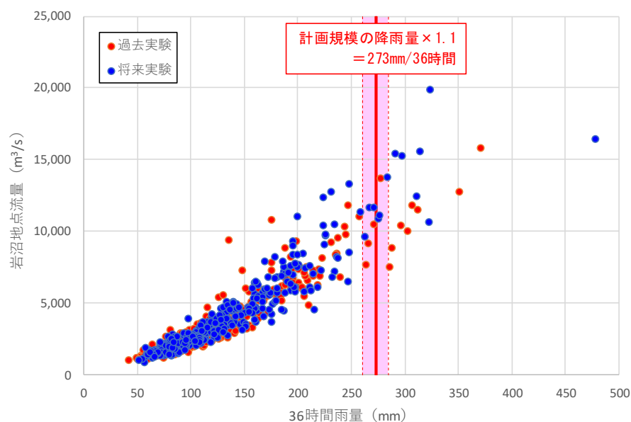
図 1-48 (2) アンサンブル予測降雨波形による流出計算結果（岩沼地点）
