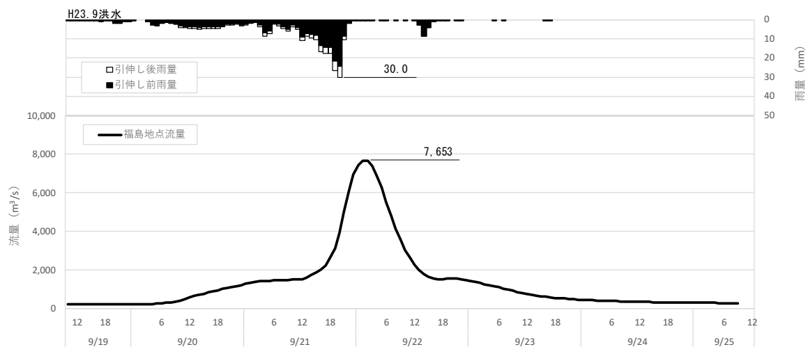
図 1-46 (20) 対象降雨の降雨 36hr 拡大による流出計算結果 (H23.9 洪水、福島地点)
