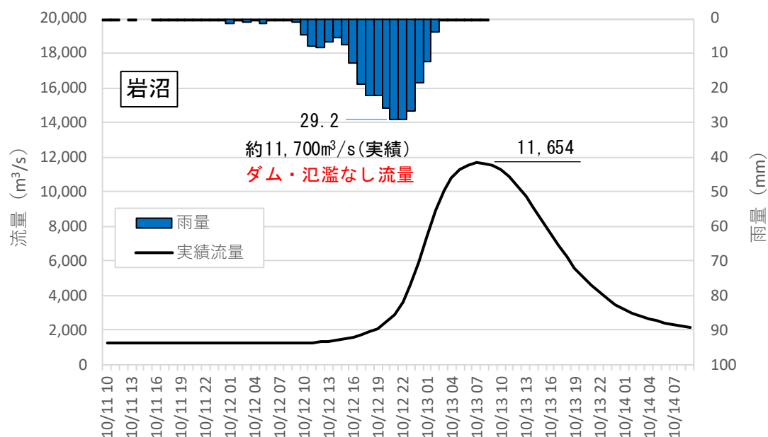
図 1-53 (2) 令和元年 10 月洪水実績流量（基準地点岩沼）
