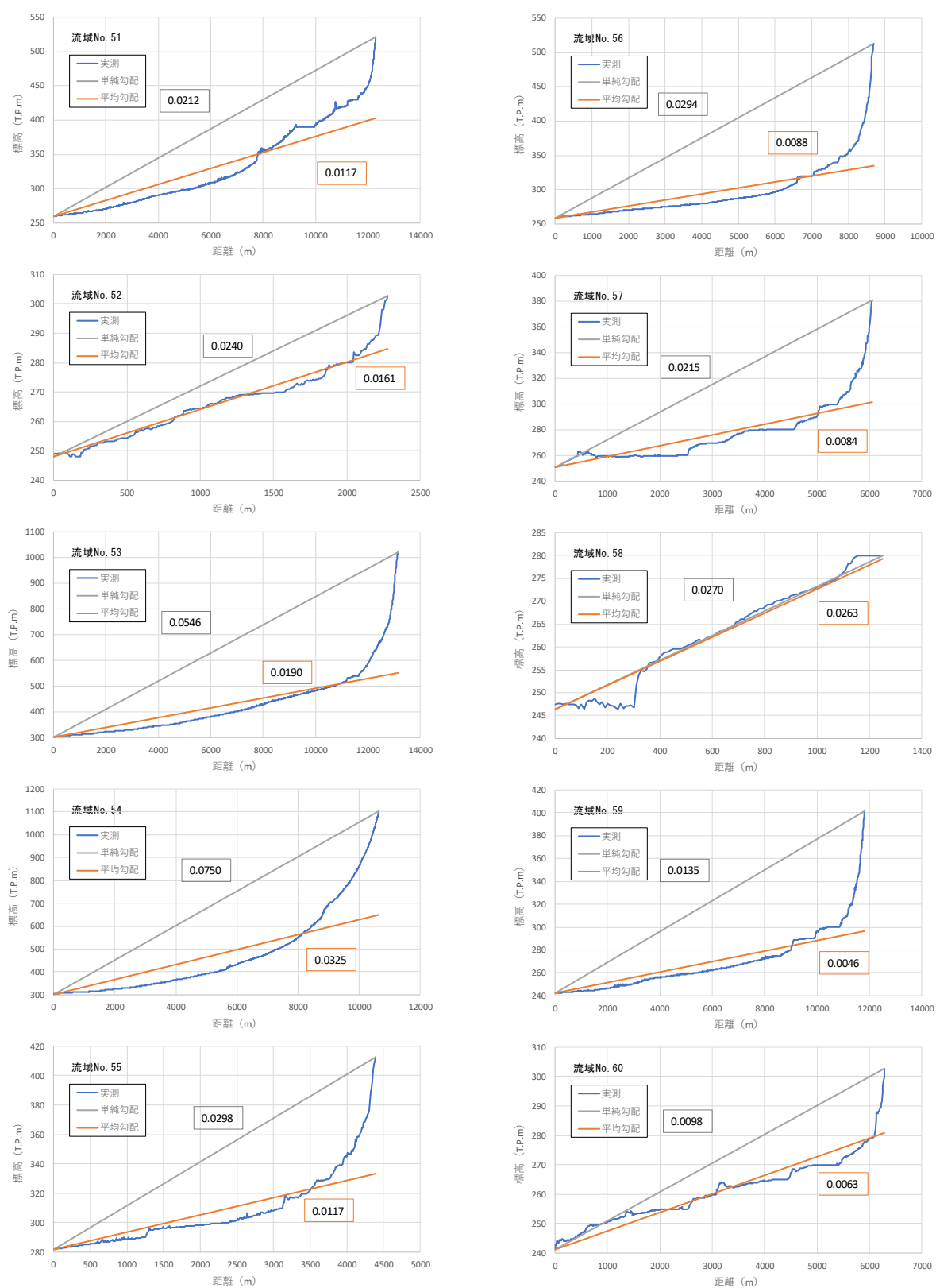
图 1-28 (6) 流域流路勾配
