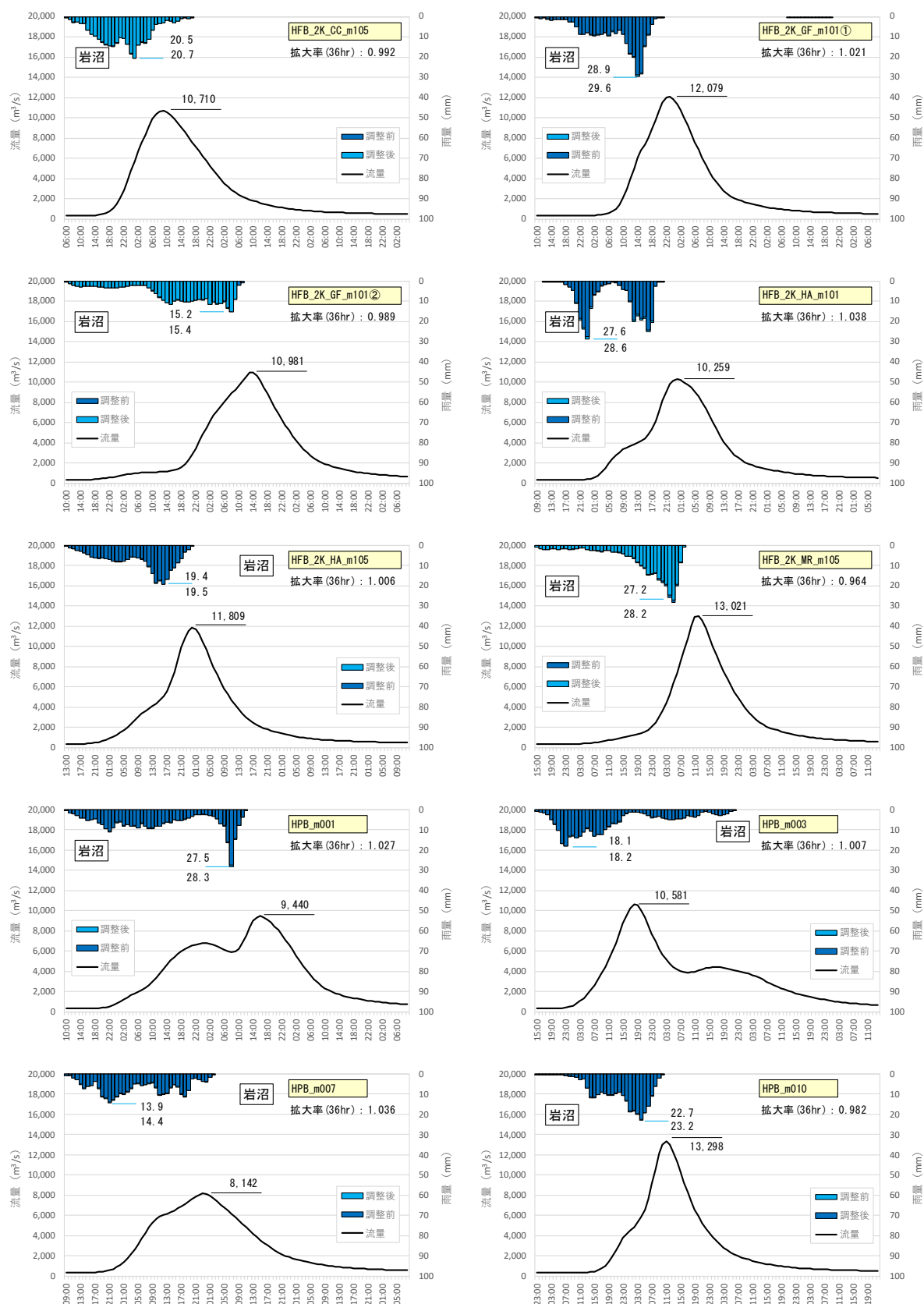
図 1-49 (2) アンサンブル予測降雨波形による流出計算結果 (岩沼地点)
