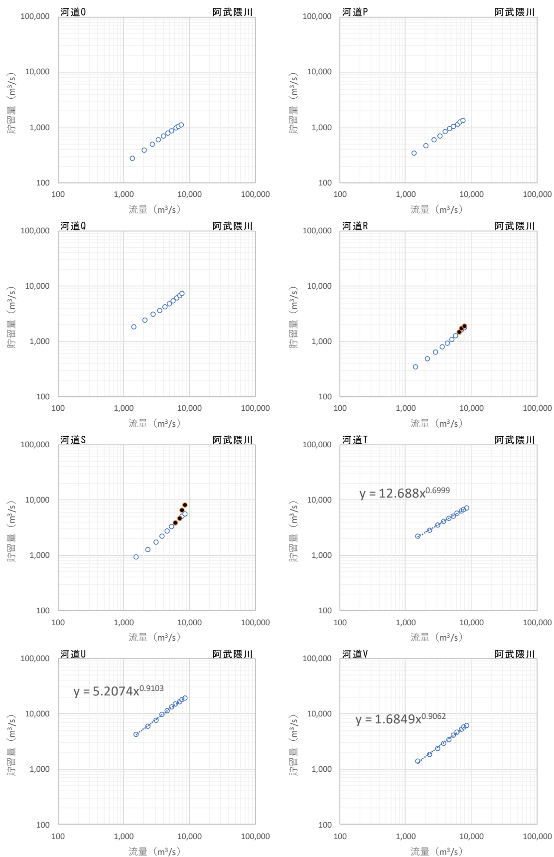
図 1-29 (4) S-Q 関係図
