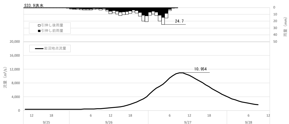
図 1-46 (2) 対象降雨の降雨 36hr 拡大による流出計算結果 (S33.9 洪水、岩沼地点)
