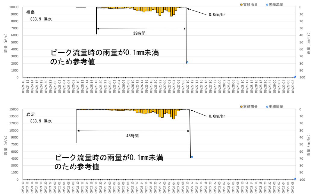
図 1-36 (7) Kinematic Wave 法による洪水到達時間
