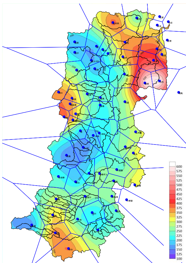
図 1-6 (2) 等雨量線図（左：地上雨量、右：レーダ雨量）（令和元年（2019 年）10 月洪水）
