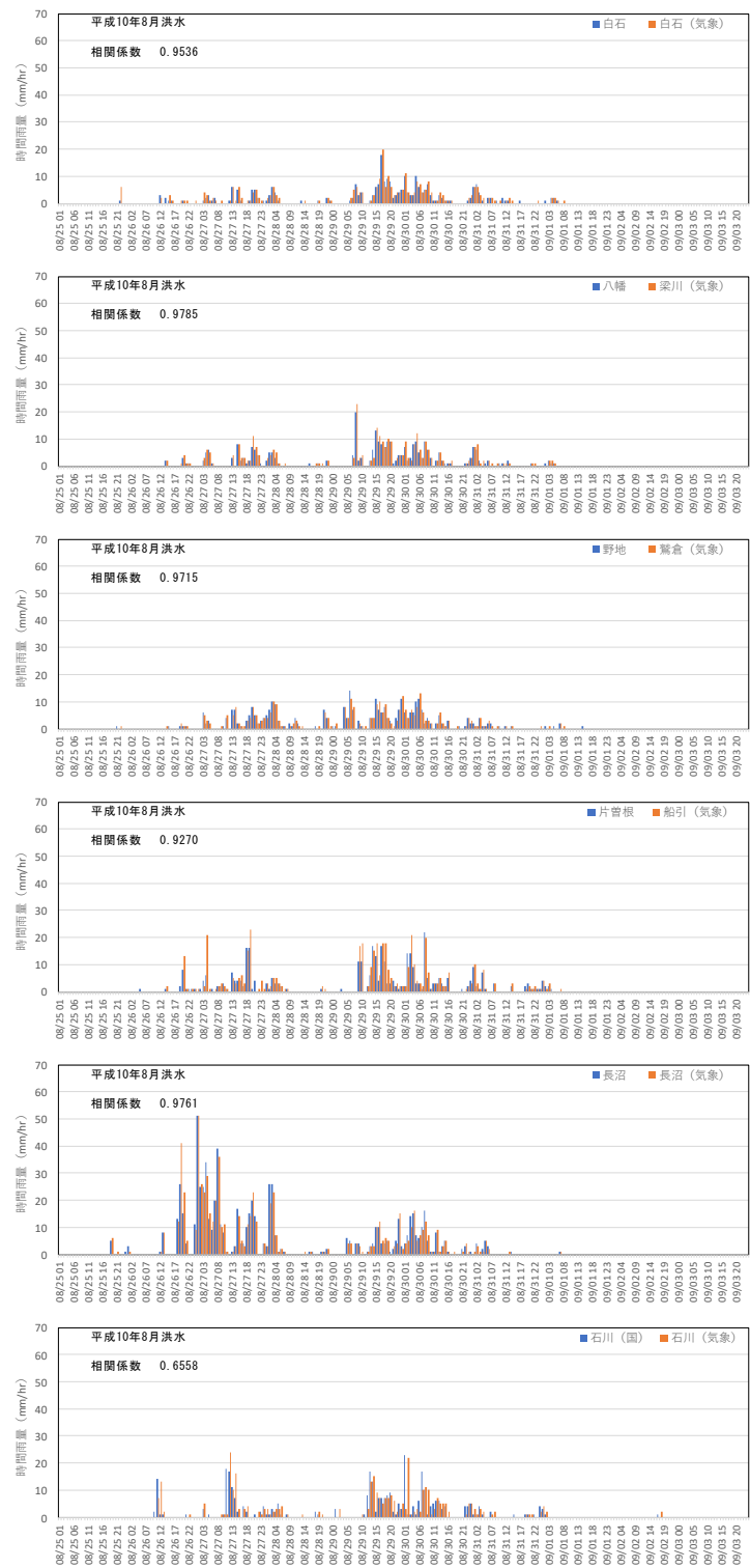
図 1-9 (2) 近傍観測所における降雨ハイトグラフの比較 (平成 10 年 8 月洪水)
