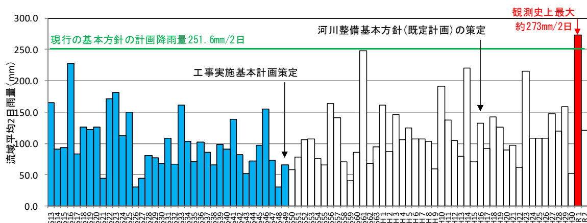
図 1-2 (2) 年最大2日雨量（基準地点岩沼上流流域平均雨量）
