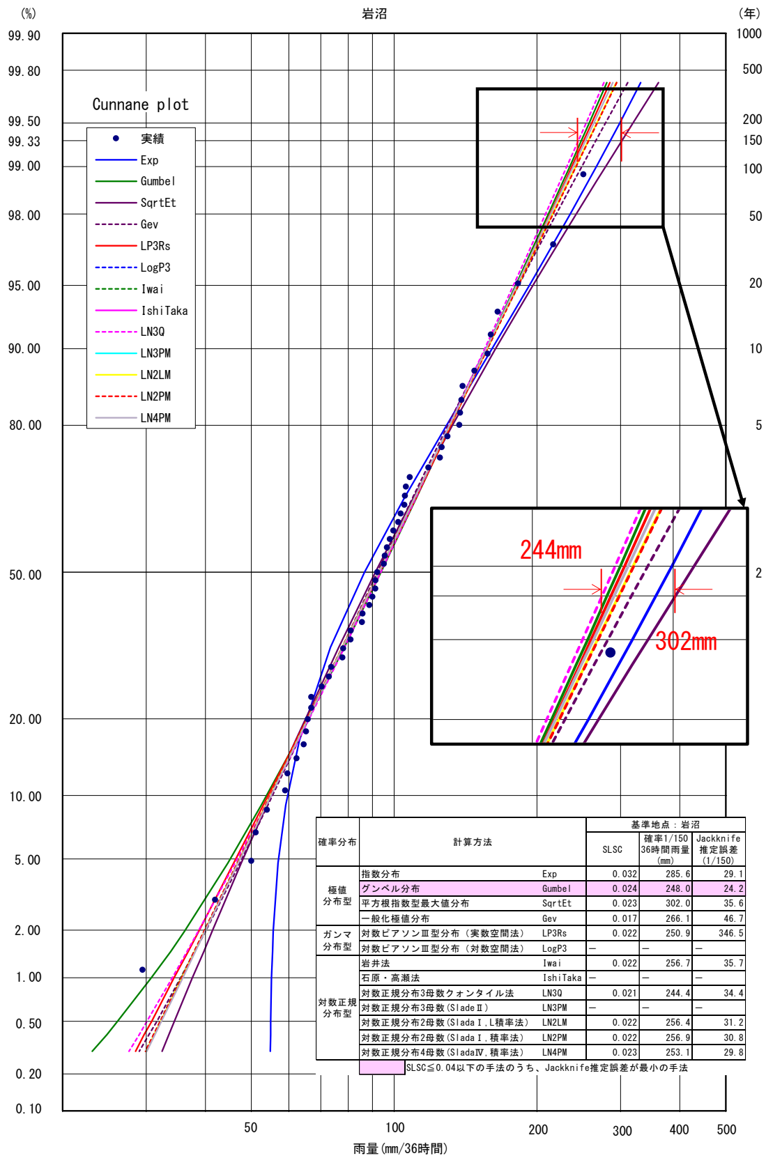
図 1-44 (2) 36 時間雨量確率図（岩沼地点）
