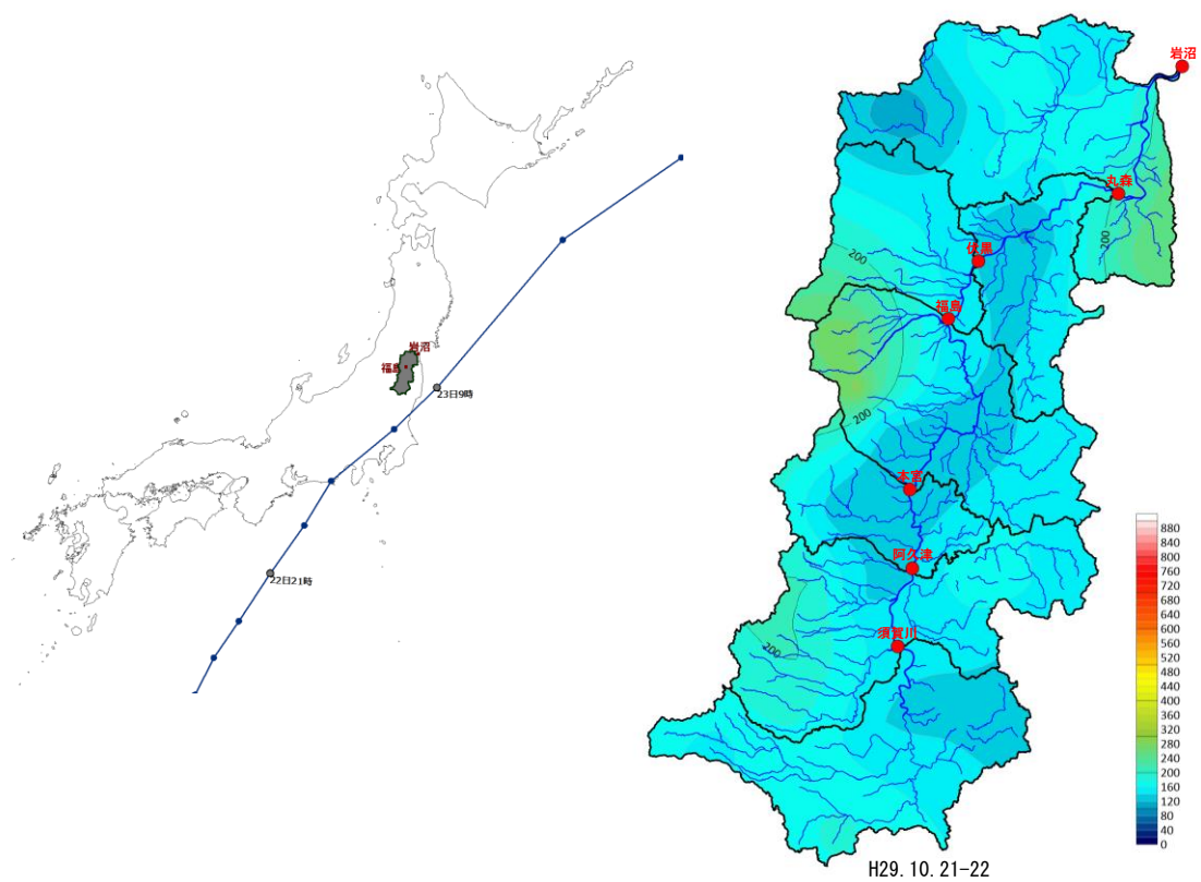
図 1-4 (13) 台風経路図及び等雨量線図 (H29.10.21-22 洪水)
