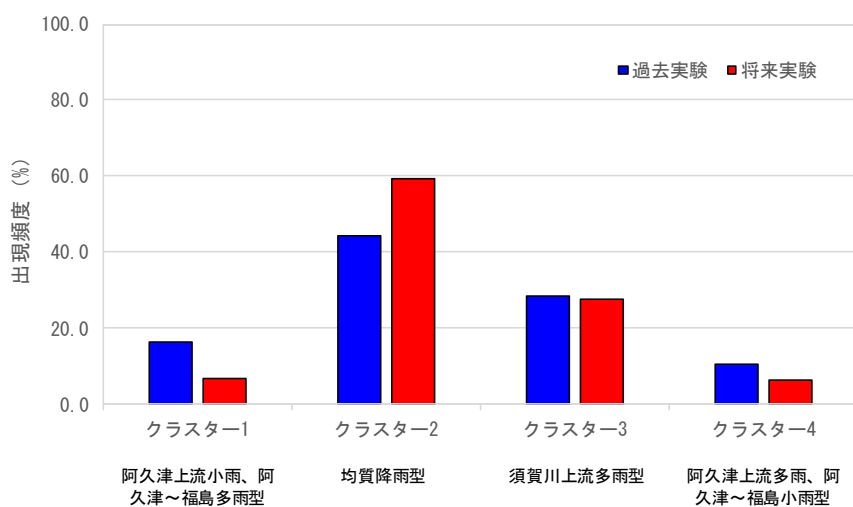
図 1-52 (1) 出現頻度 (福島地点)
