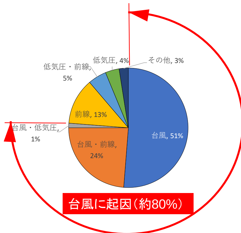
図 1-3 洪水要因比較図 (対象 80 洪水による)
