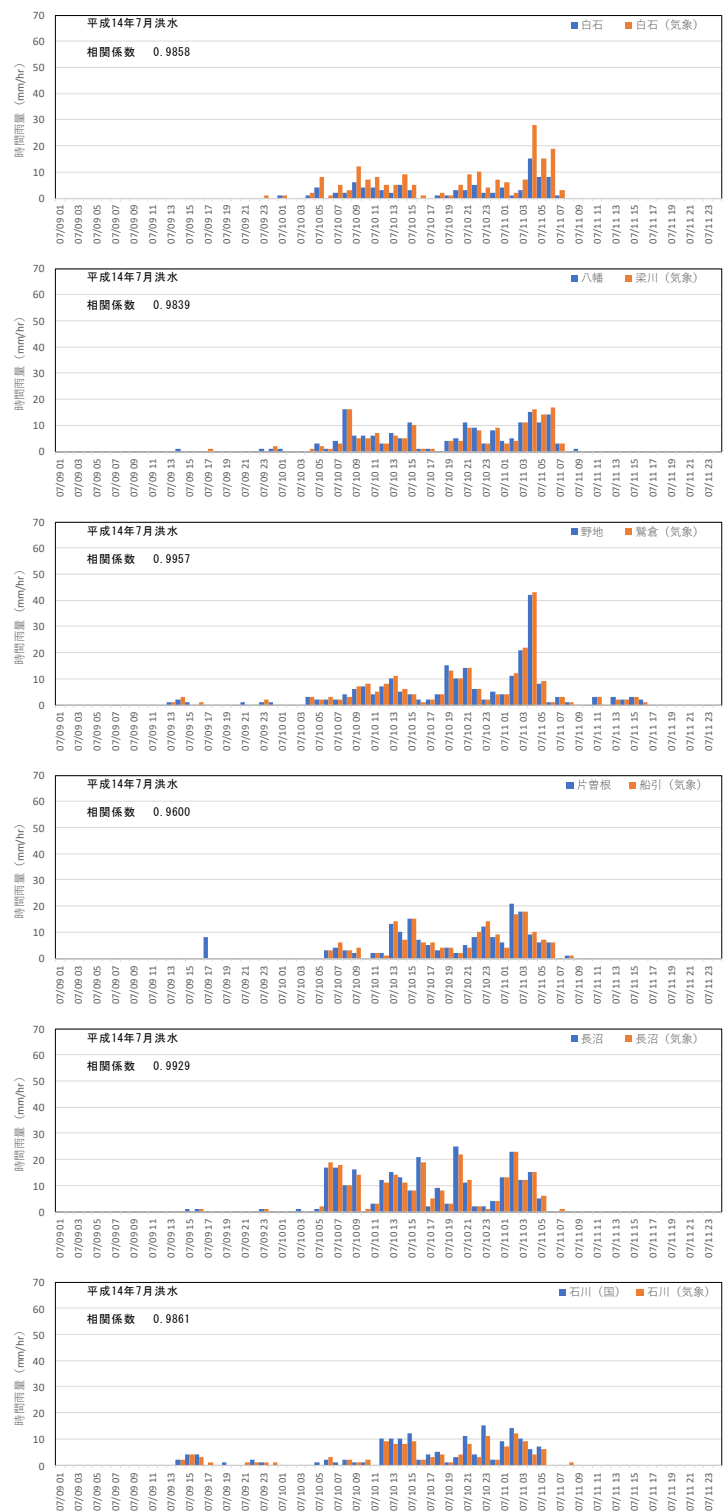
図 1-9 (3) 近傍観測所における降雨ハイトグラフの比較 (平成 14 年 7 月洪水)
