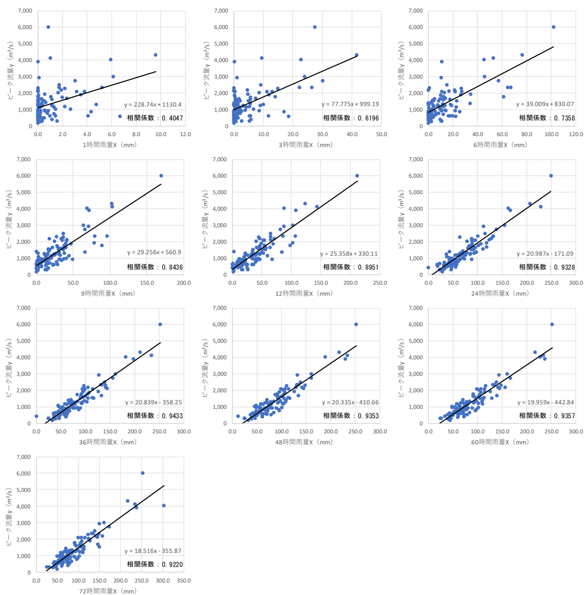
図 1-40 (1) ピーク流量と雨量との相関関係
