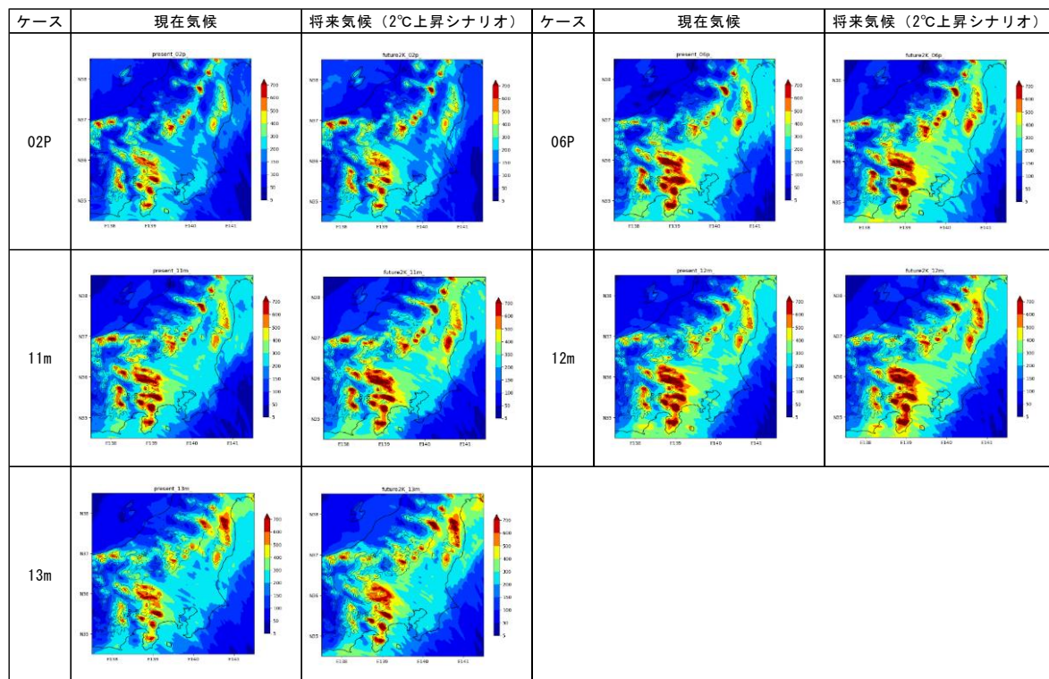
図 1-55 累積降水量(詳細)(5 ケース, NHRM)
