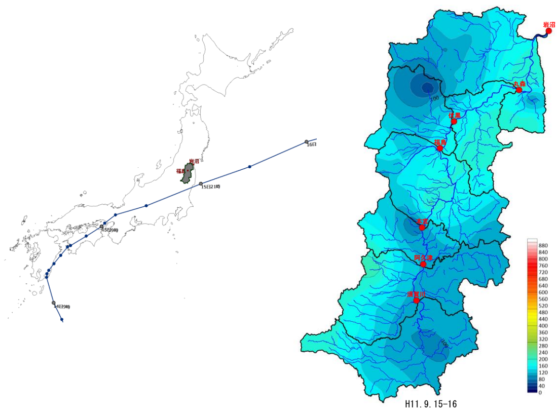
図 1-4 (7) 台風経路図及び等雨量線図 (H11.9.15-16 洪水)
