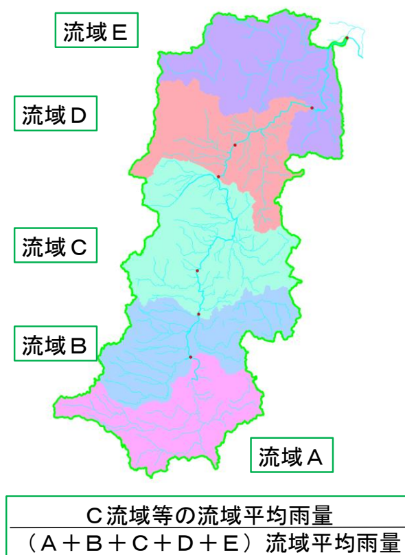
図 1-50 空間分布のチェック
