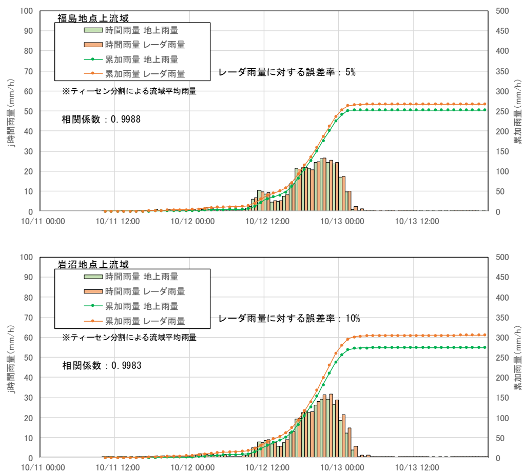
図 1-5 (2) 地上観測所雨量とレーダ雨量の比較（令和元年（2019 年）10 月洪水）
