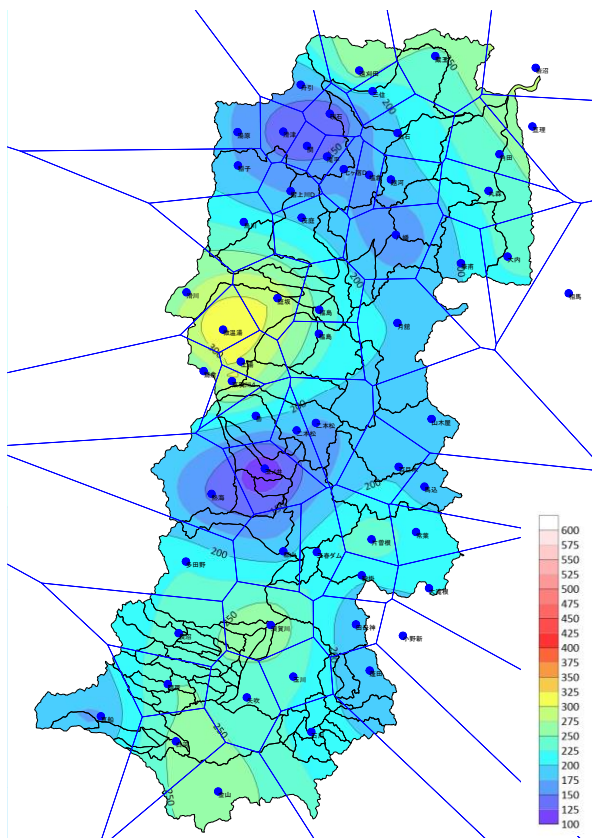
図 1-6 (1) 等雨量線図（左：地上雨量、右：レーダ雨量）（平成 23 年（2011 年）9 月洪水）
