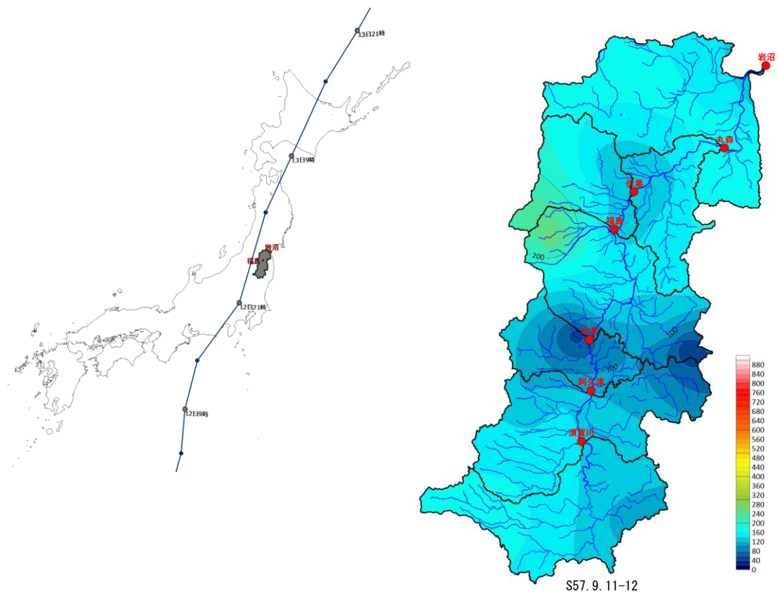
図 1-4 (3) 台風経路図及び等雨量線図 (S57.9.11-12 洪水)
