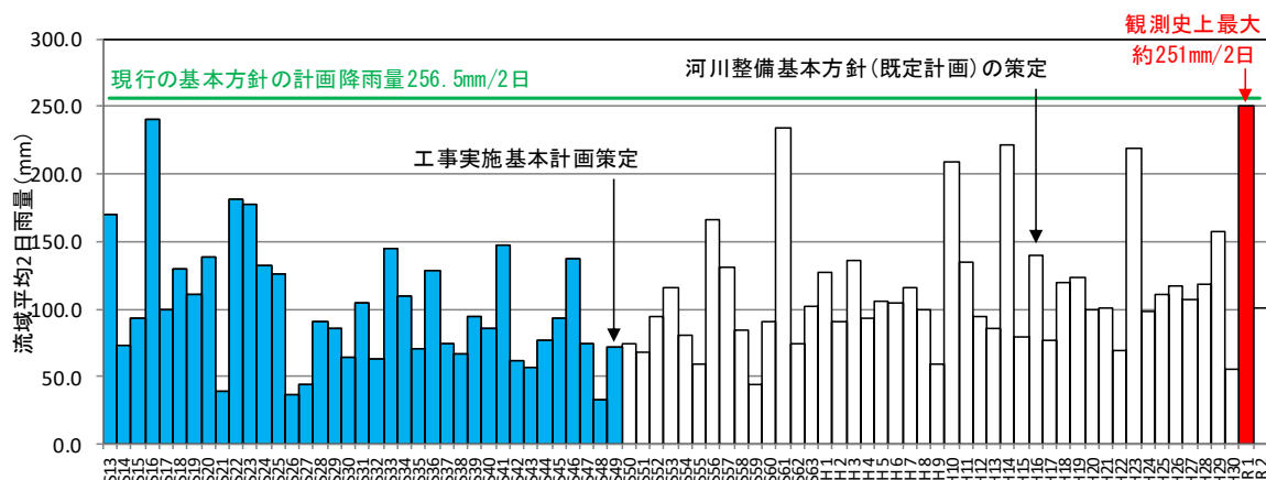
図 1-2 (1) 年最大2日雨量（基準地点福島上流流域平均雨量）
