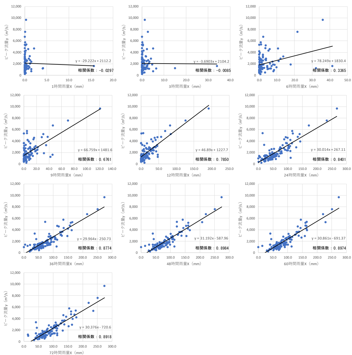
図 1-40 (3) ピーク流量と雨量との相関関係
