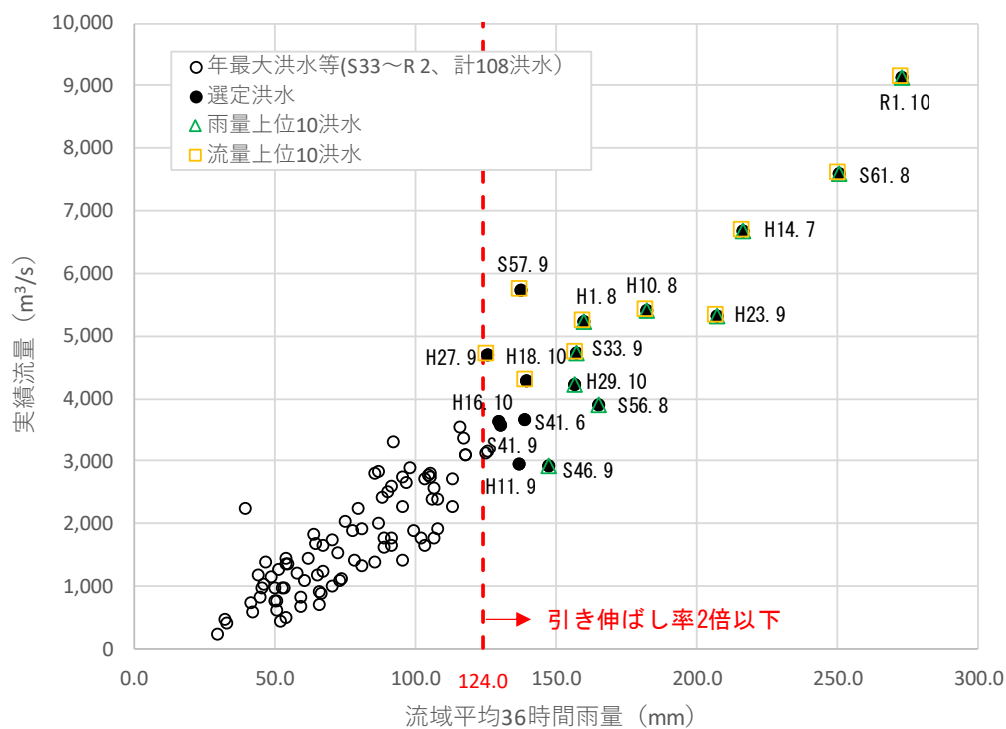
図 1-45 (2) 代表洪水の選定結果（岩沼地点）
