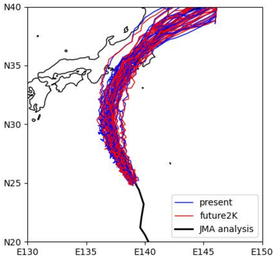
図 1-54 令和元年東日本台風の経路
