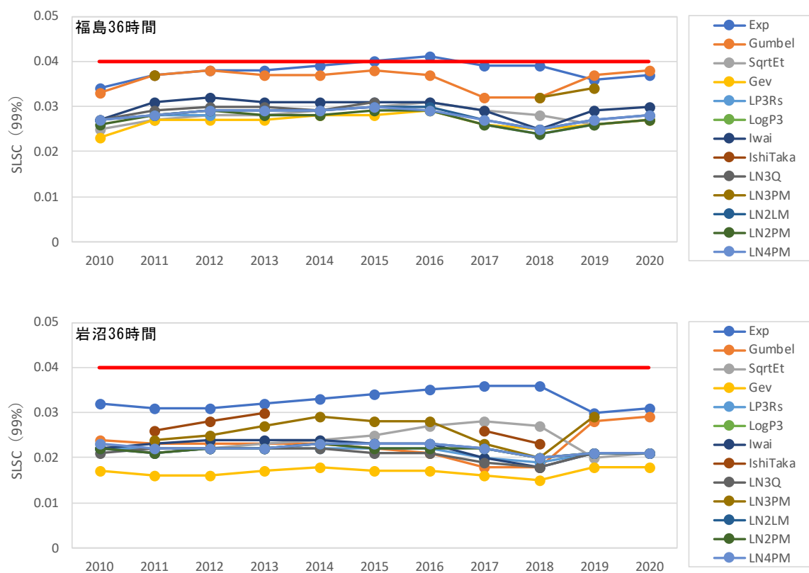
図 1-43 標本追加による SLSC の推移
