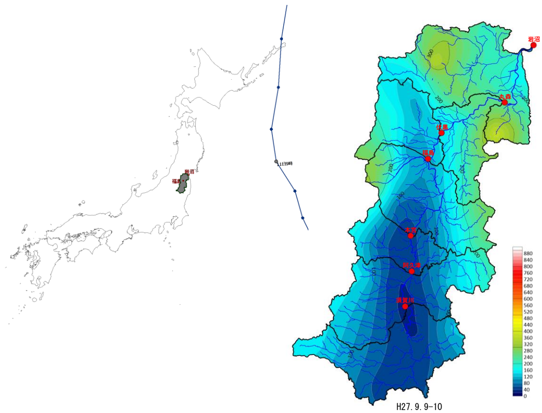
図 1-4 (12) 台風経路図及び等雨量線図 (H27.9.9-10 洪水)
