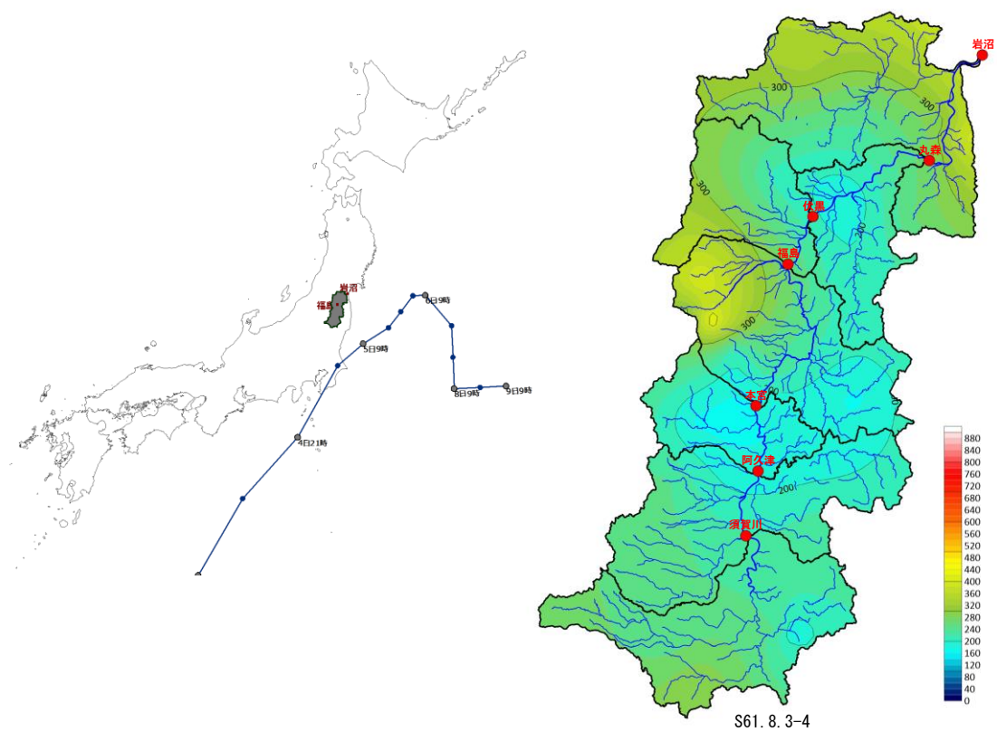
図 1-4 (4) 台風経路図及び等雨量線図 (S61.8.3-4 洪水)
