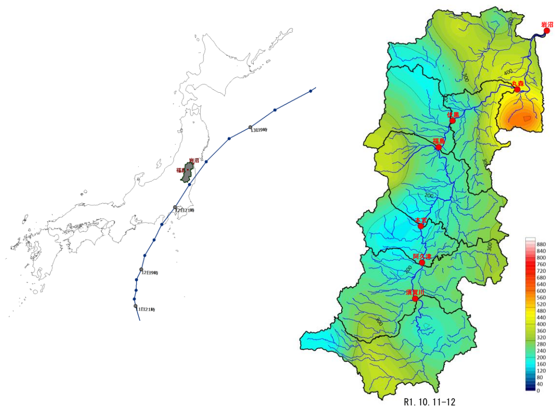
図 1-4 (14) 台風経路図及び等雨量線図 (R1.10.11-12 洪水)
