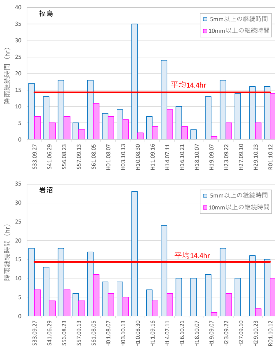
図 1-41 強い降雨強度の継続時間
