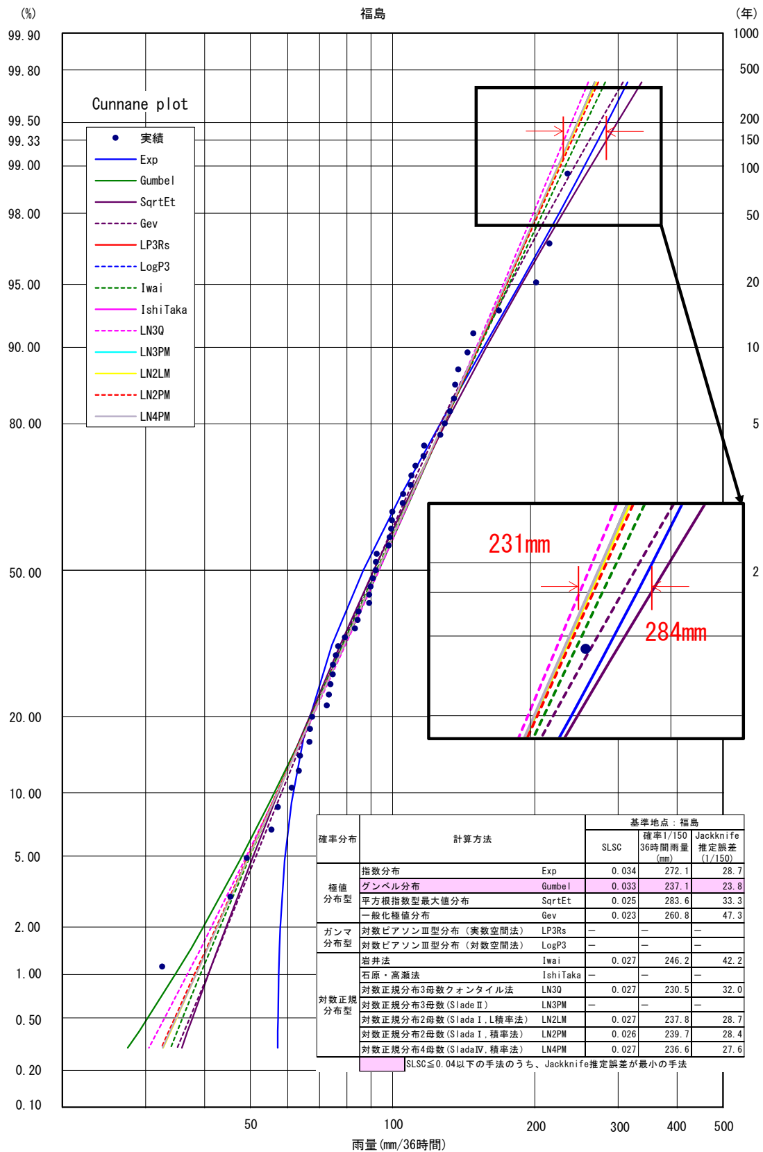
図 1-44 (1) 36 時間雨量確率図 (福島地点)
