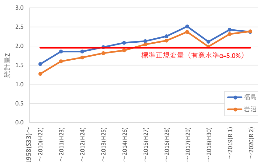
図 1-42 Mann-Kendall 検定結果
