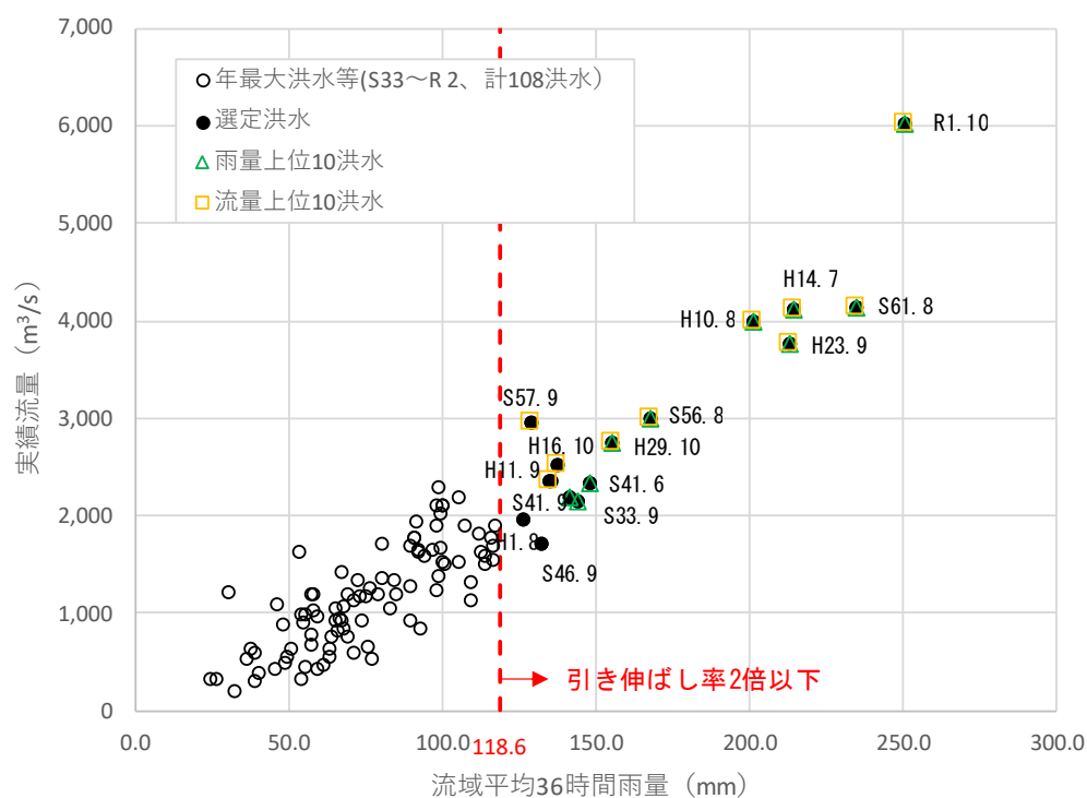
図 1-45 (1) 代表洪水の選定結果（福島地点）
