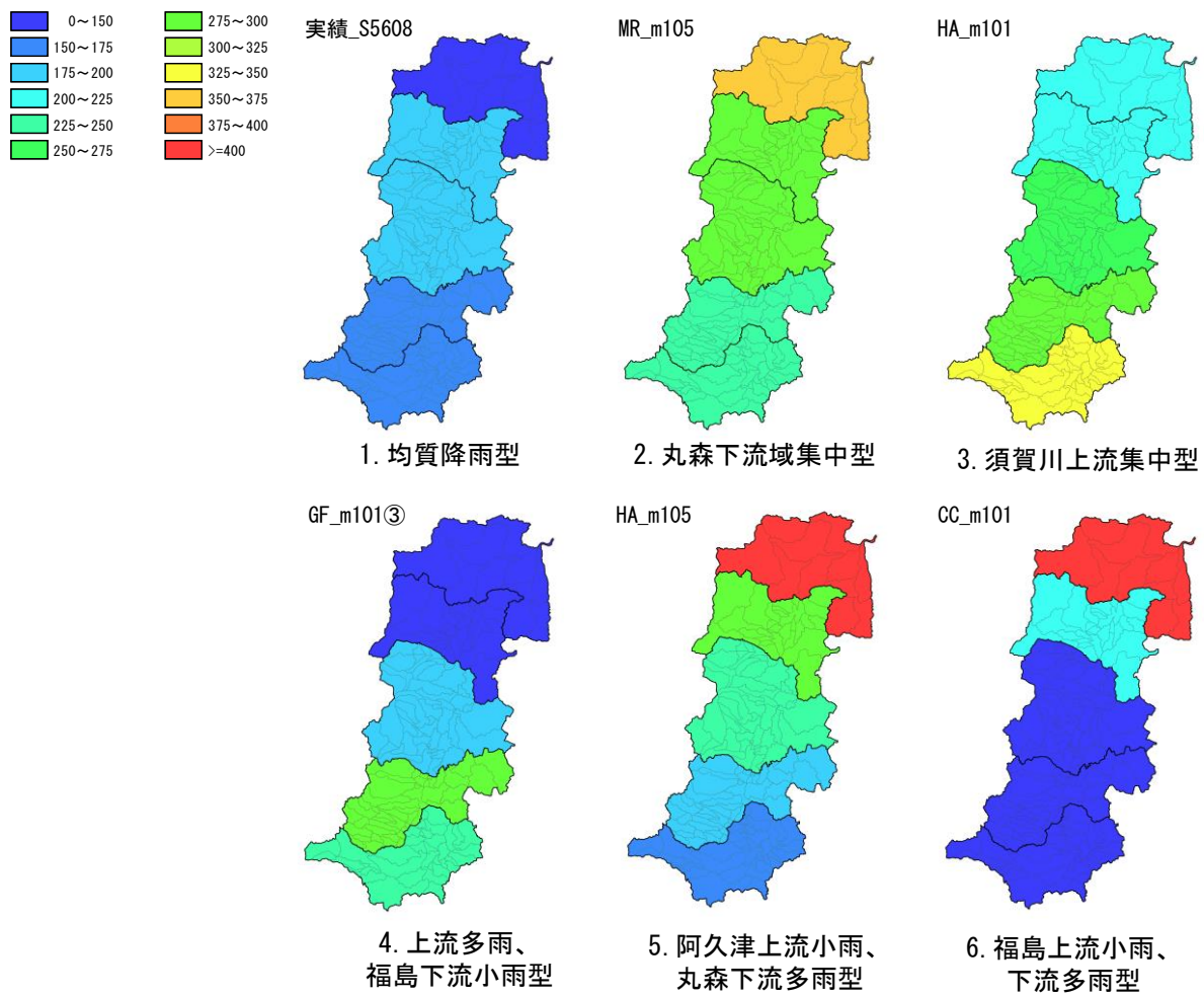
図 1-51 (2) 降雨パターンの分析結果 (岩沼地点)
