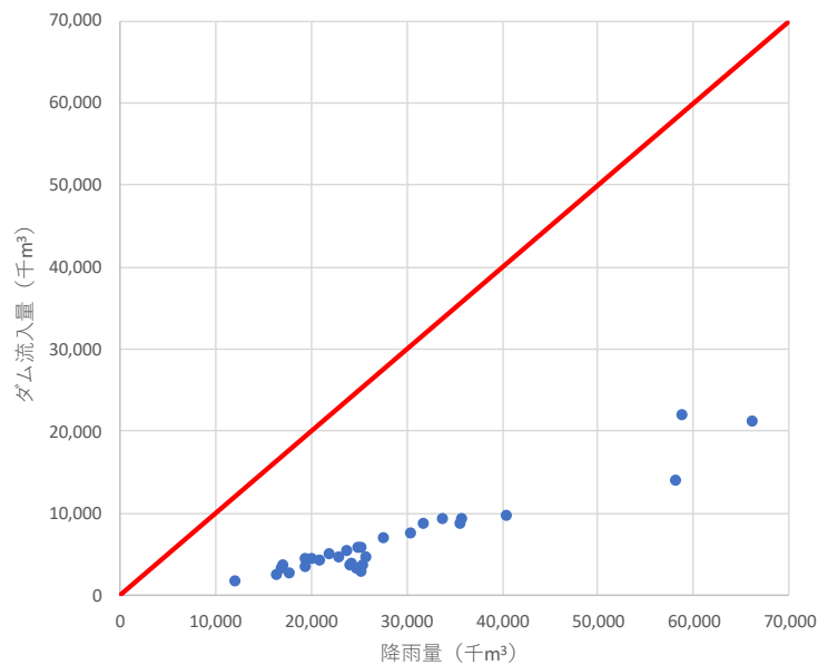
図 1-12 (1) ダム地点における流入量と降雨量の関係 (三春ダム)
