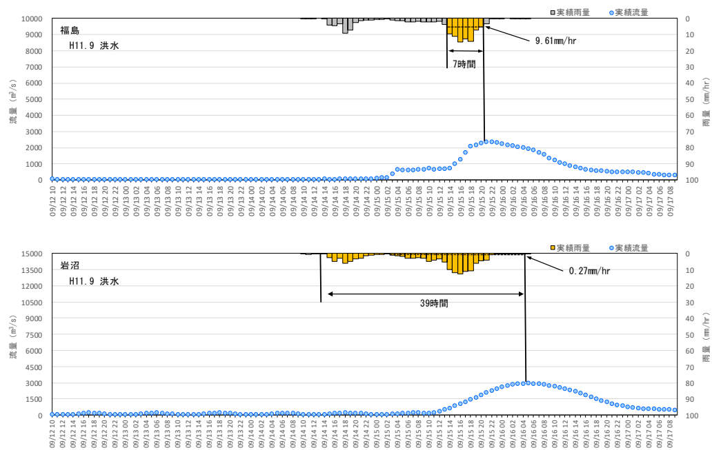
図 1-36 (4) Kinematic Wave 法による洪水到達時間
