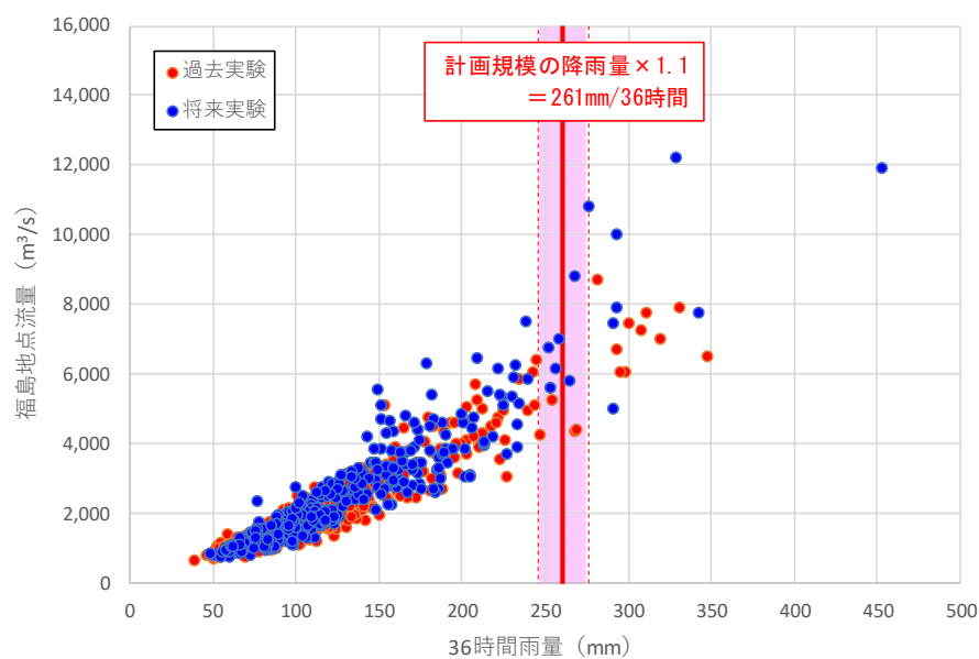
図 1-48 (1) アンサンブル予測降雨波形による流出計算結果（福島地点）
