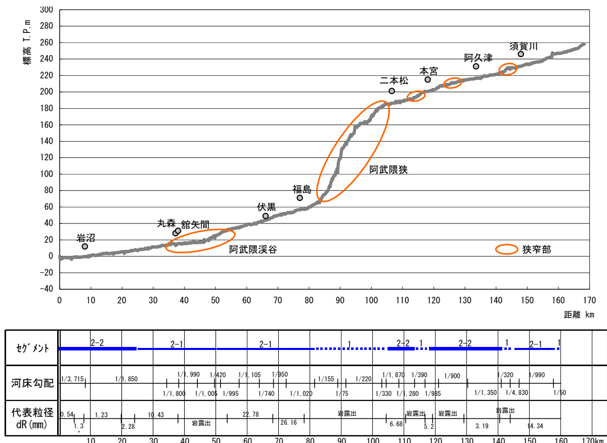
図 2-1-1 阿武隈川における平均河床高縦断図と河道特性図
