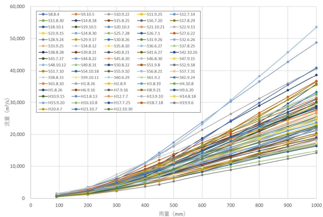
図 1.20 Q_p - P_{(Q_p)} 図
