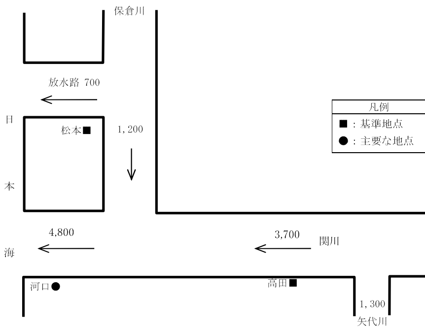
図 4-2 関川計画高水流量図（単位：m³/s）（平成 19 年関川水系河川整備基本方針記載）
