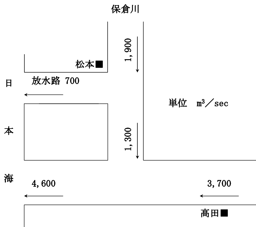
図 4-1 関川計画高水流量図（昭和 62 年度工事実施基本計画記載）
