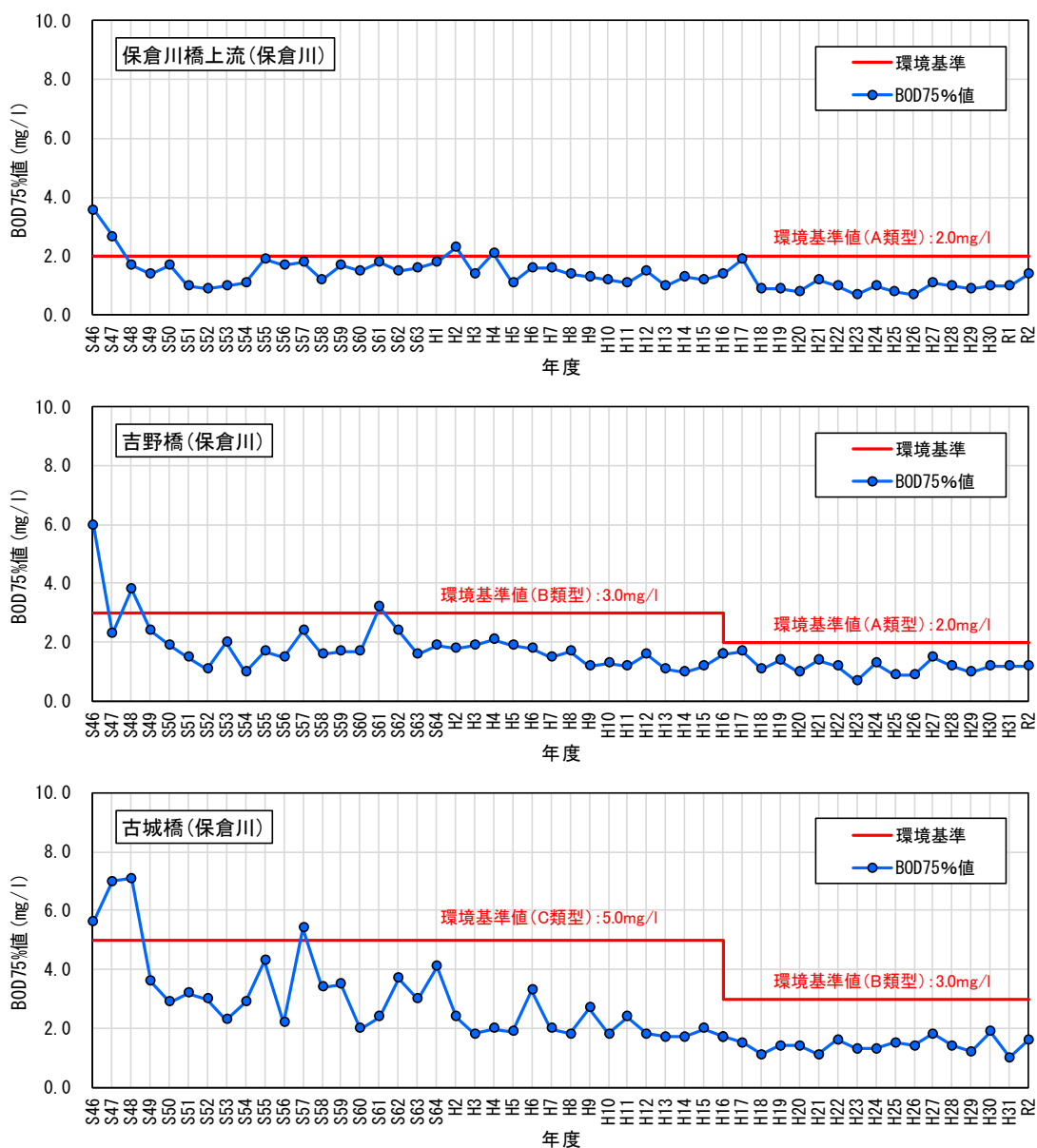
図 6-2 (2) 水質 (BOD75%値) の経年変化 (保倉川)
