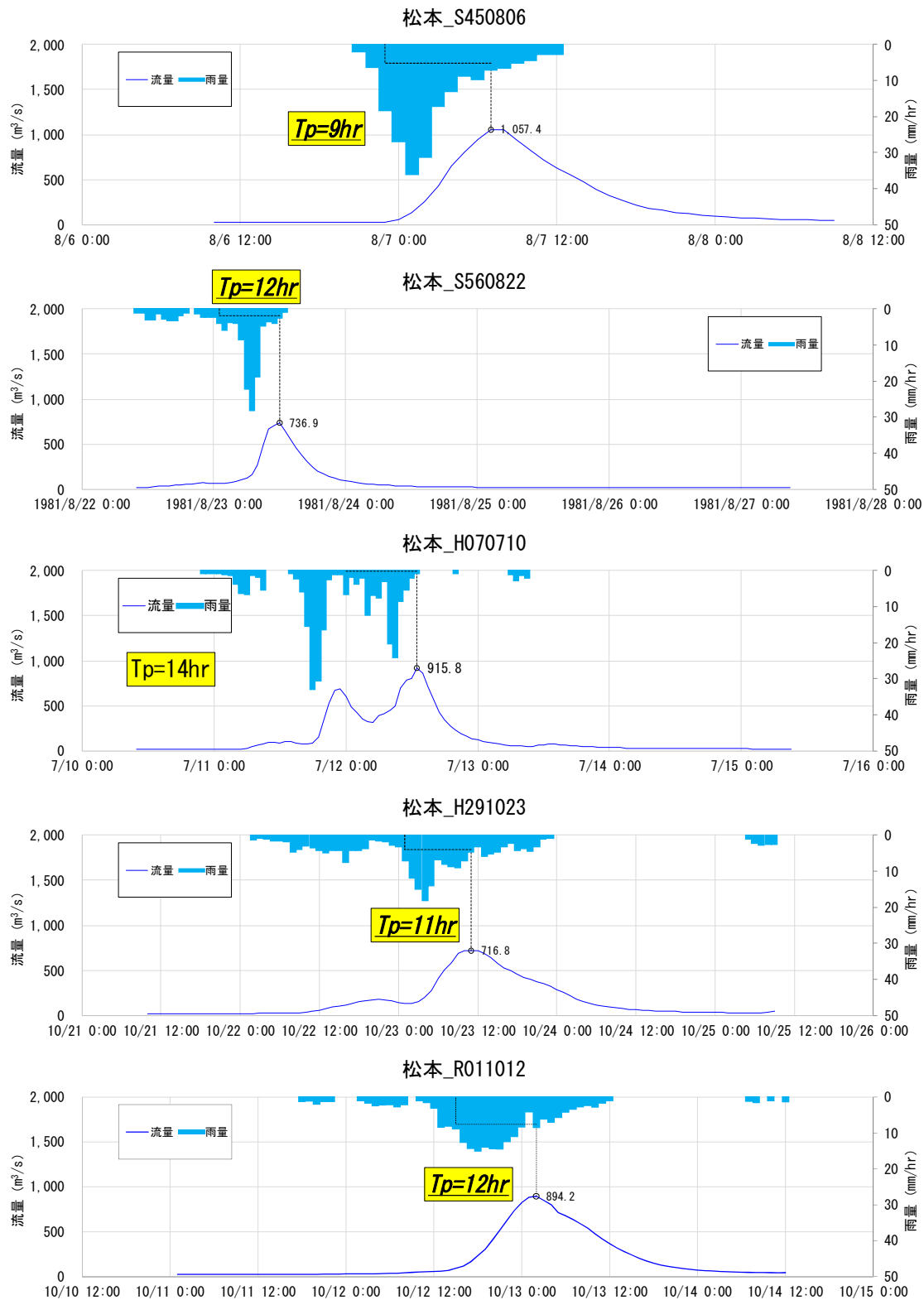
図 1-4(2) Kinematic Wave 法による洪水到達時間 (基準地点 松本)
