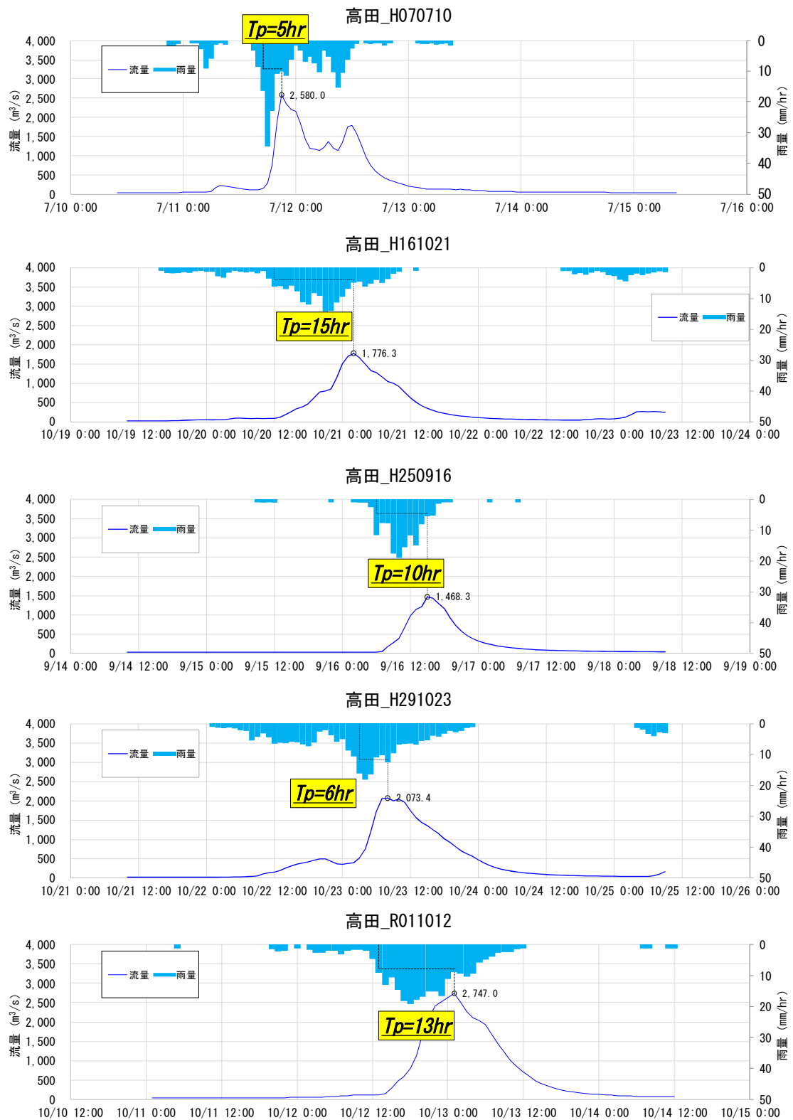
図 1-3 (2) Kinematic Wave 法による洪水到達時間 (基準地点 高田)
