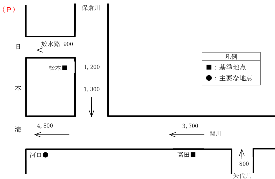
図 3-1 関川計画高水流量図 (単位 : \text{m}^3/\text{s} )
