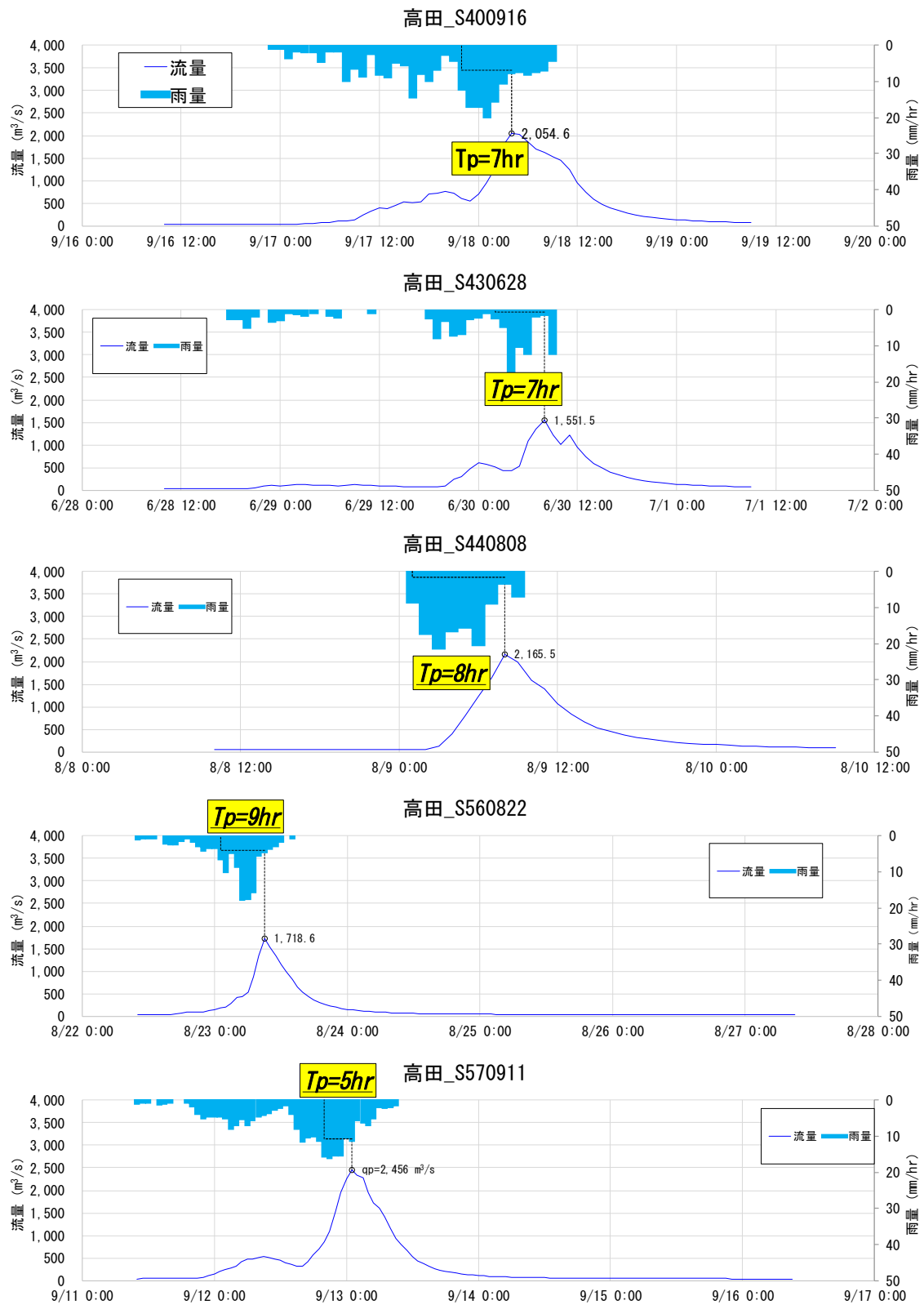
図 1-3(1) Kinematic Wave 法による洪水到達時間 (基準地点 高田)
