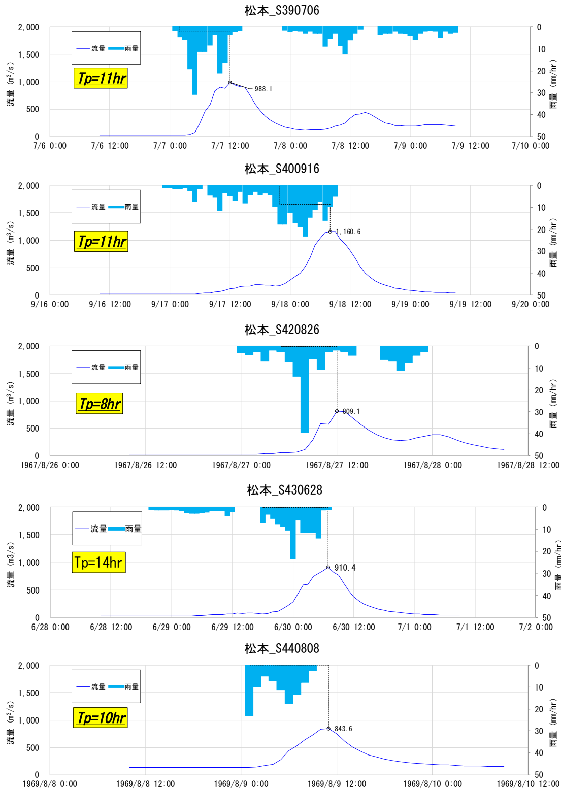
図 1-4(1) Kinematic Wave 法による洪水到達時間 (基準地点 松本)
