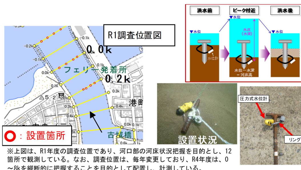
図4-1 洪水時河床モニタリング（リングセンサー設置）
