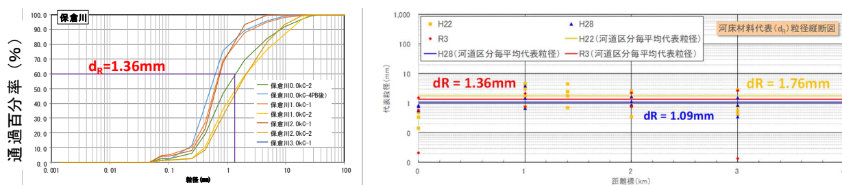
図 2 - 1 4 令和 3 年河床材料調査通過百分率図と保倉川代表粒径縦断面図
