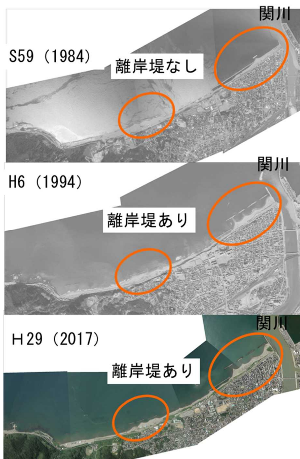
図3-4 関川河口部西側の離岸堤による汀線の変化
