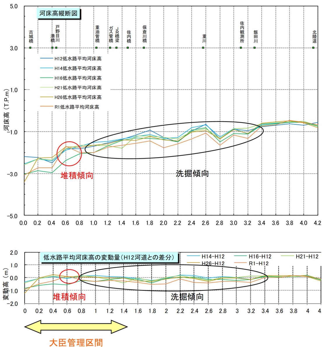
図 2 - 5 低水路平均河床高縦断面図と河床変動量縦断面図 (保倉川)
