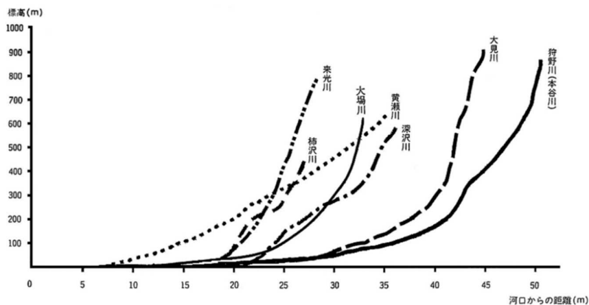
図 8-1-1 狩野川縦断図
