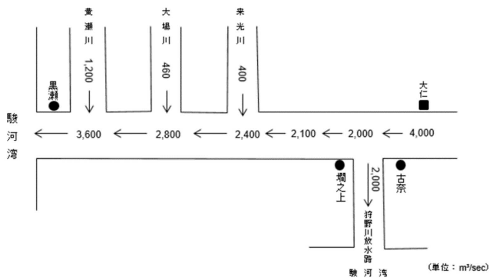
図 4-2-1 狩野川 計画高水流量図
