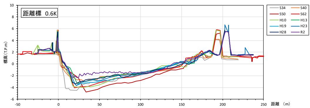
図 8-2-4 代表横断面図（狩野川 0k600）
