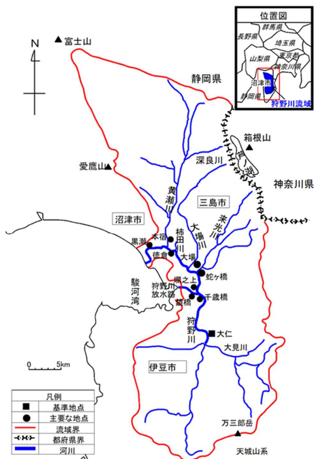
図 1-1-1 狩野川流域図
