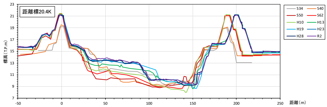
図 2-5 代表横断面図（狩野川 20k400）
