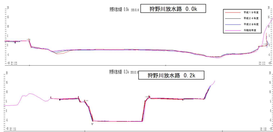
図 3-5 狩野川放水路河口部の代表横断図
