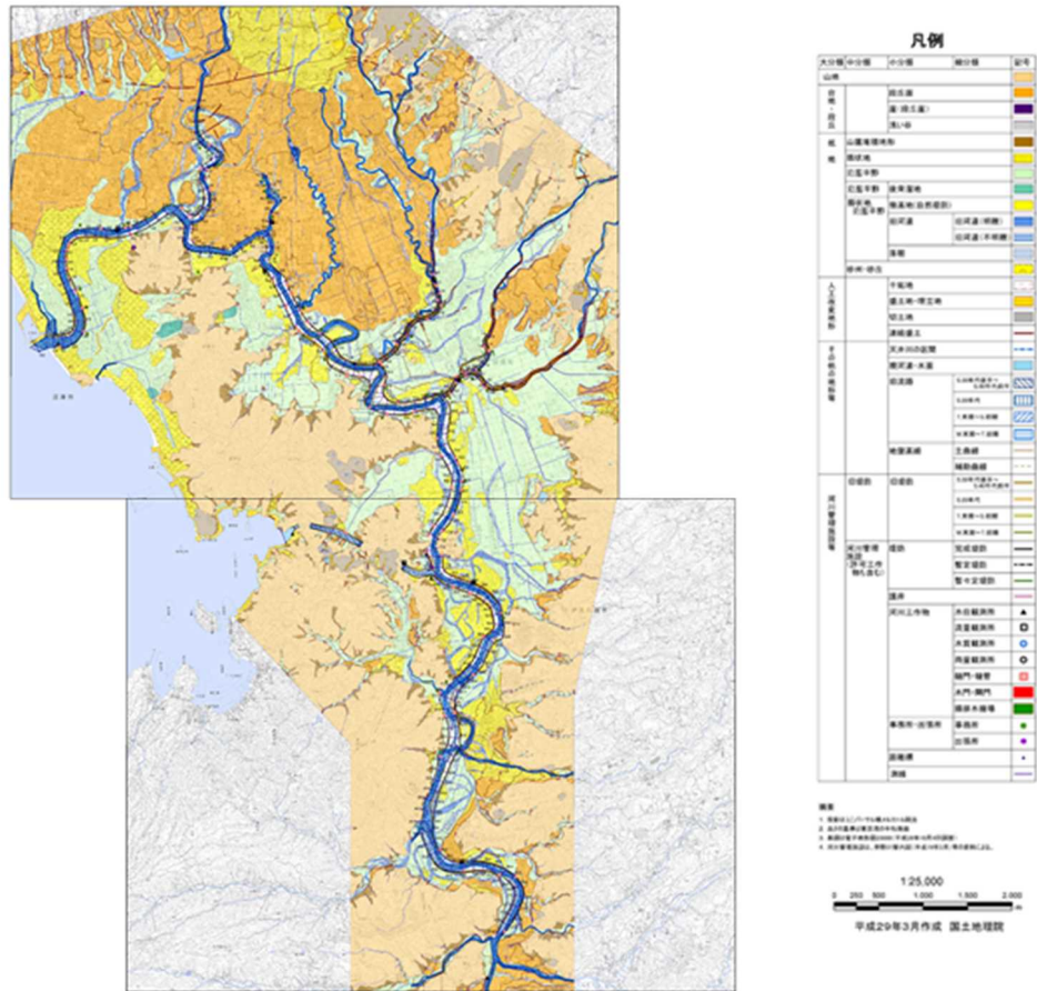
図 1-3 狩野川流域 地形分類
