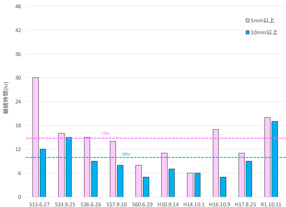
図 1-6-8 強い降雨強度の継続時間（基準地点大仁上流域平均雨量）
