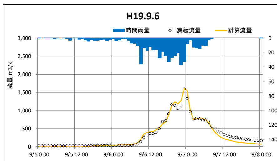
図 1-8-7 平成 19 年 9 月洪水再現計算結果
