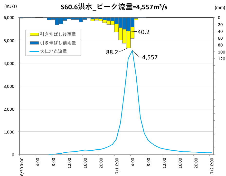
図 1-14-2 基本高水のピーク流量ハイドログラフ（昭和 60 年 6 月洪水：大仁）
