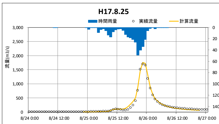
図 1-8-6 平成 17 年 8 月洪水再現計算結果
