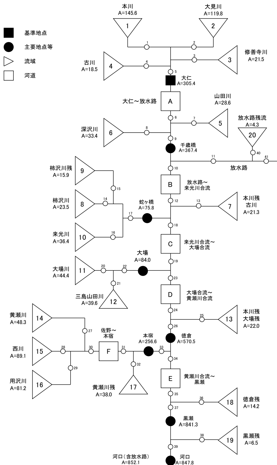
図 1-8-14 狩野川水系流出解析モデル図
