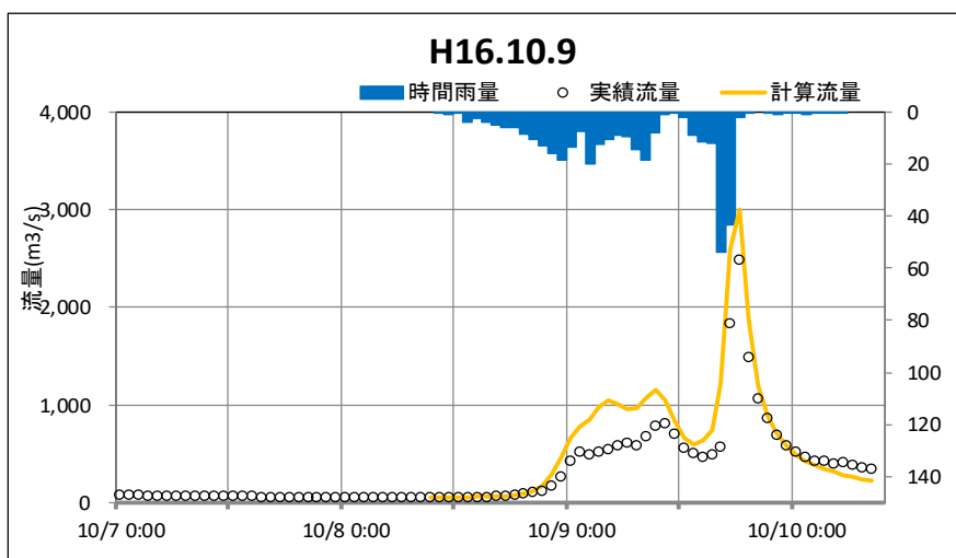
図 1-8-5 平成 16 年 10 月洪水再現計算結果
