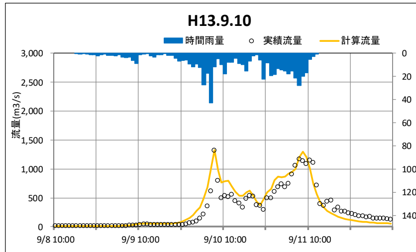
図 1-8-3 平成 13 年 9 月洪水再現計算結果
