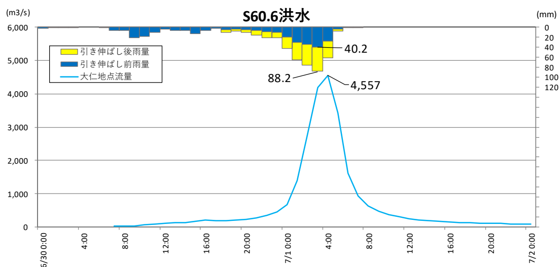
図 1-11-5 基本高水ハイドログラフ（昭和 60 年 6 月洪水 大仁地点）
