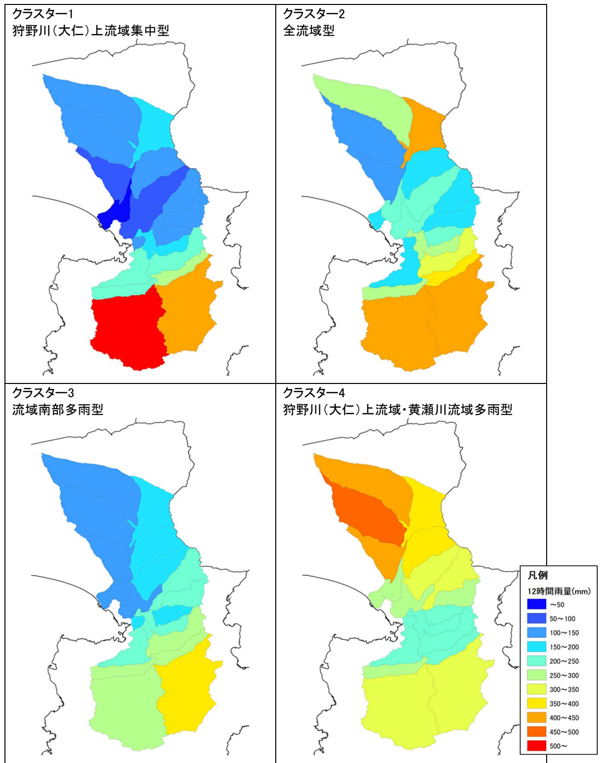
図 1-12-7 狩野川流域における将来実験アンサンブル予測降雨の クラスター分析結果
