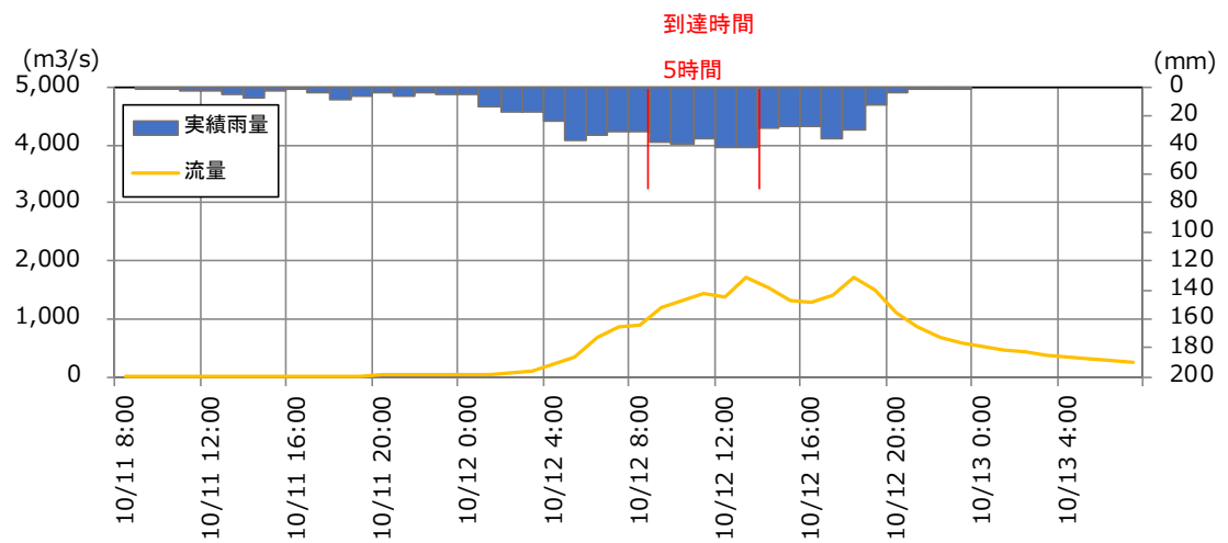
図 1-6-4 Kinematic Wave 法による洪水到達時間(4) (基準地点大仁)
