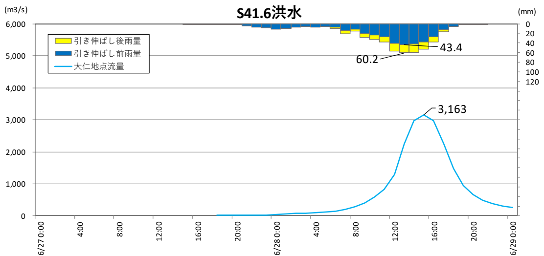
図 1-11-3 基本高水ハイドログラフ（昭和 41 年 6 月洪水 大仁地点）
