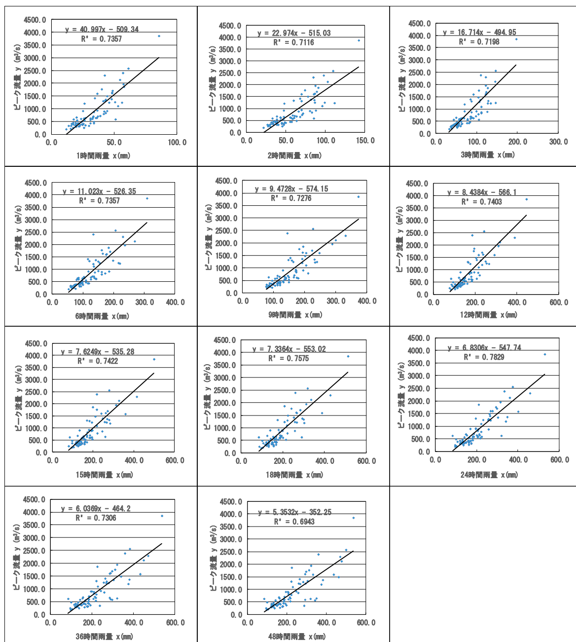
図 1-6-6 ピーク流量と流域平均時間雨量の相関図（基準地点大仁）【定義①】
