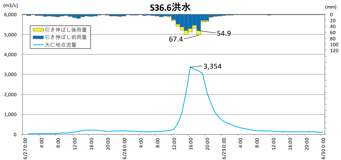
図 1-11-2 基本高水ハイドログラフ（昭和 36 年 6 月洪水 大仁地点）
