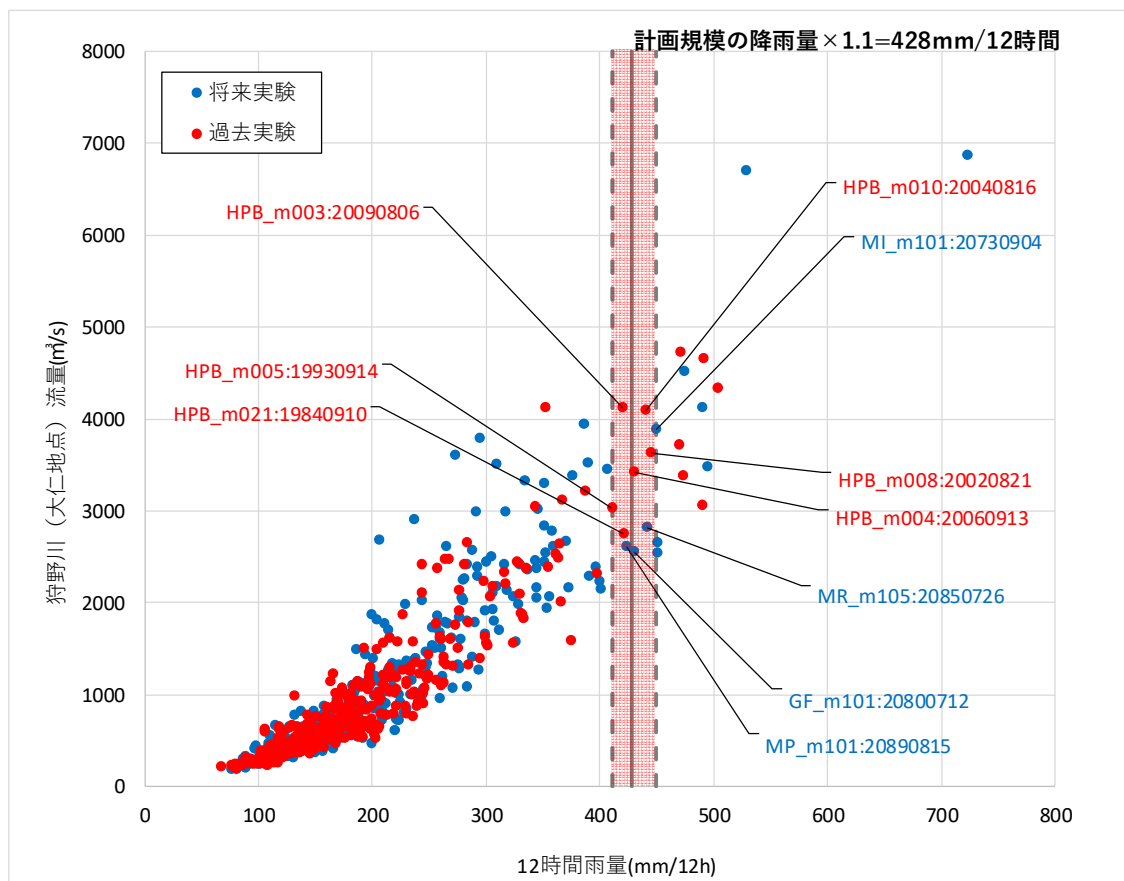
図 1-12-1 アンサンブル予測降雨波形からの抽出 (大仁地点)
