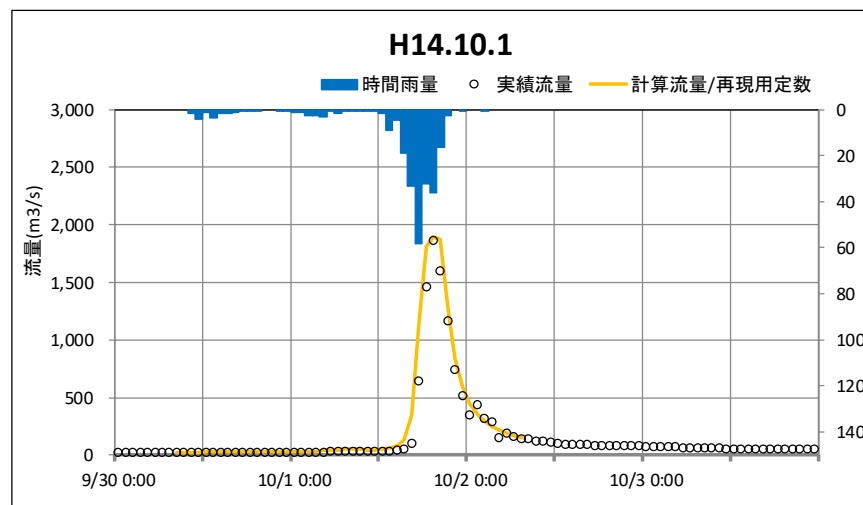
図 1-8-4 平成 14 年 10 月洪水再現計算結果
