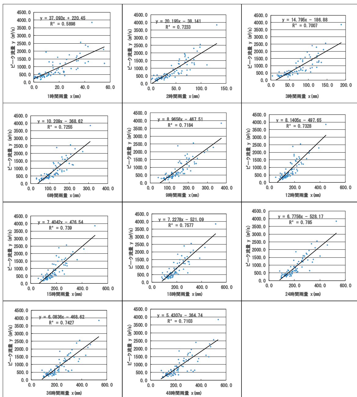
図 1-6-7 ピーク流量と流域平均時間雨量の相関図（基準地点大仁）【定義②】
