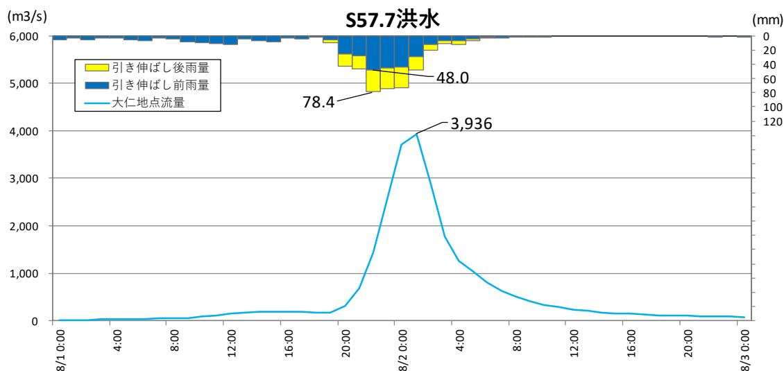
図 1-11-4 基本高水ハイドログラフ（昭和 57 年 7 月洪水 大仁地点）
